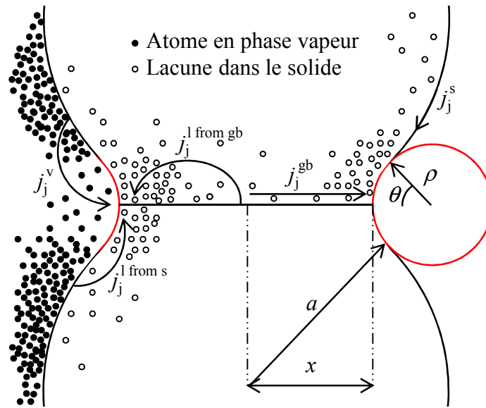
Figure 11 : Modèle à deux sphères couramment utilisé pour décrire le premier stade du frittage. Le transport de matière est induit par la courbure négative du cou entre les deux particules (en rouge). A cet endroit, la concentration en lacunes, dans le solide, y est plus élevée et la concentration en atomes, dans la phase vapeur, y est plus faible. Les flux de matières peuvent alors suivre cinq chemins différents. Trois d'entre eux sont originaires de la surface des particules et sont donc non-densifiant : le transport vapeur, j_j^v , la diffusion de surface, j_j^s , et la diffusion en volume depuis la surface des particules, j_j^{l from s} . Deux d'entre eux sont originaires du joint de grain, ils induisent alors un rapprochement des particules et sont donc densifiant : la diffusion au joint de grain, j_j^{gb} , et la diffusion en volume depuis le joint de grain, j_j^{l from gb} .
