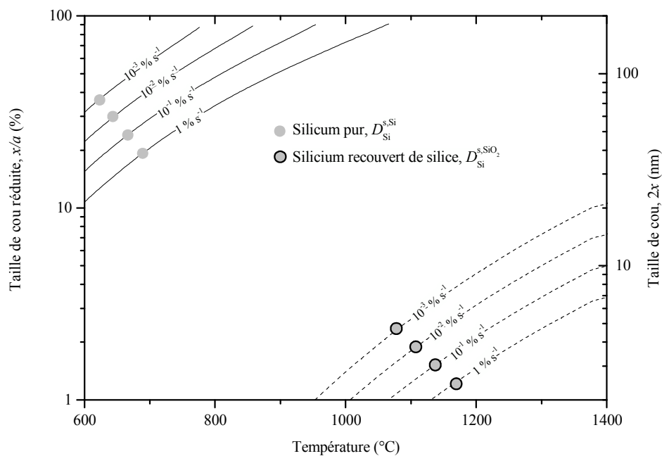
Figure 12 : Courbes de vitesse de croissance de taille de cou pour le mécanisme de diffusion de surface dans le cas du silicium pur et du silicium recouvert de silice. La taille des particules ( 2a = 220 \text{ nm} ) est représentative de la poudre VF utilisée.
