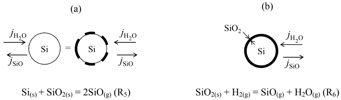
Figure 4 : Mécanismes de réduction de la silice envisagés pour deux configurations : (a) une couche de silice fragmentée à la surface de la particule de silicium, (b) une couche de silice continue et passive à la surface de la particule de silicium.
