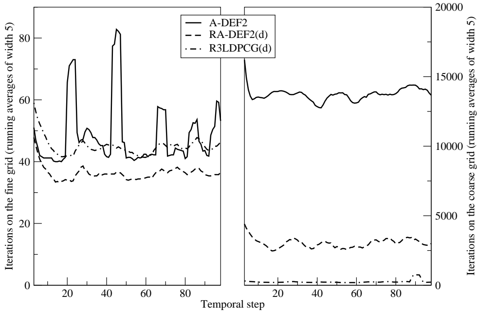
FIGURE 6.37 – Moyennes flottantes de largeur 5 des nombres d'itérations sur les deux premiers niveaux de maillages des méthodes A-DEF2 , RA-DEF2(d) et R3LDPCG(d) , pour la simulation de 100 pas de temps d'un écoulement à température constante dans le brûleur PRECCINSTA , sur un maillage de 110 millions d'éléments sur 512 processeurs, avec un critère de convergence de 10^{-10} .
