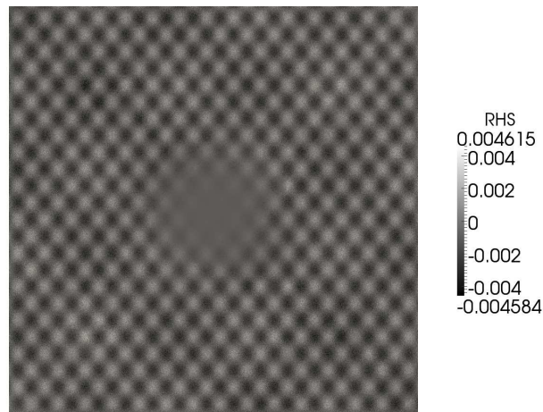
FIGURE 6.20 – Membre de droite de l'équation de Poisson résolue pour le cas-test Poisson_2D .
