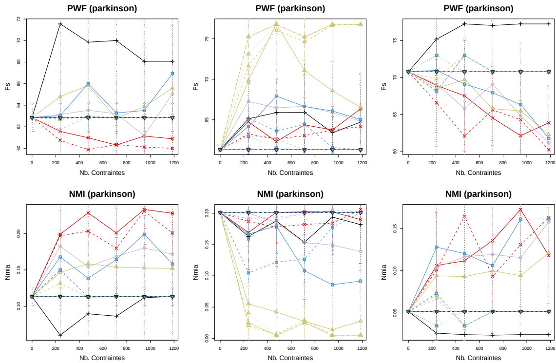
FIGURE 3.20 — Comparaison des approches BOc, UzABOc, ADAUzABOc et BC sur le jeu Parkinson centré et réduit avec contraintes bruitées.
