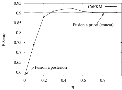
FIGURE 2.6 — CoFKM sur mfeat pour différentes valeurs de \eta . On remarque que l'heuristique de mfeat . FIGURE 2.7 — Évolution du critère CoFKM sur mfeat . Le choix de \eta permet de dépasser la performance de la fusion a priori .
