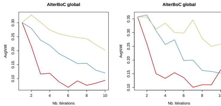
FIGURE 4.9 — Évolution de l' AvgNMI pour le clustering multi-vues et l'heuristique global. Dans l'ordre, les données mfeat avec le même algorithme pour toutes les six vues, et mfeat avec des algorithmes différents pour chaque vue.
