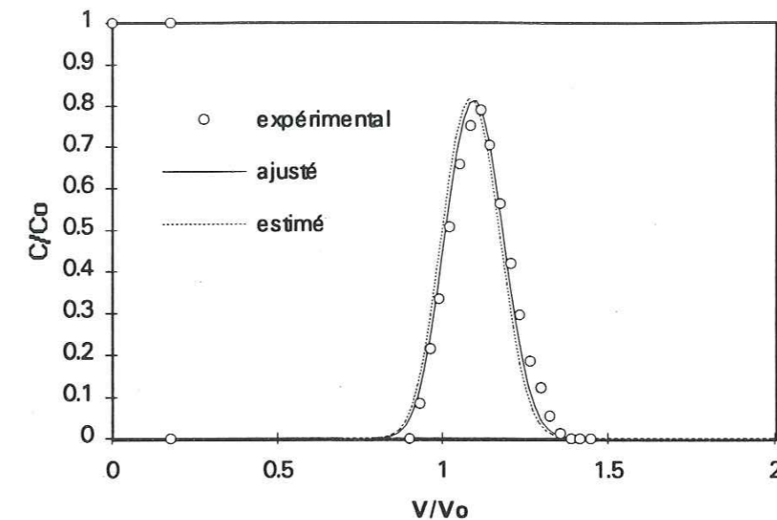
Figure 4.16 - Courbe de sortie du KCl calculée pour des valeurs de paramètres estimés et ajustés.
