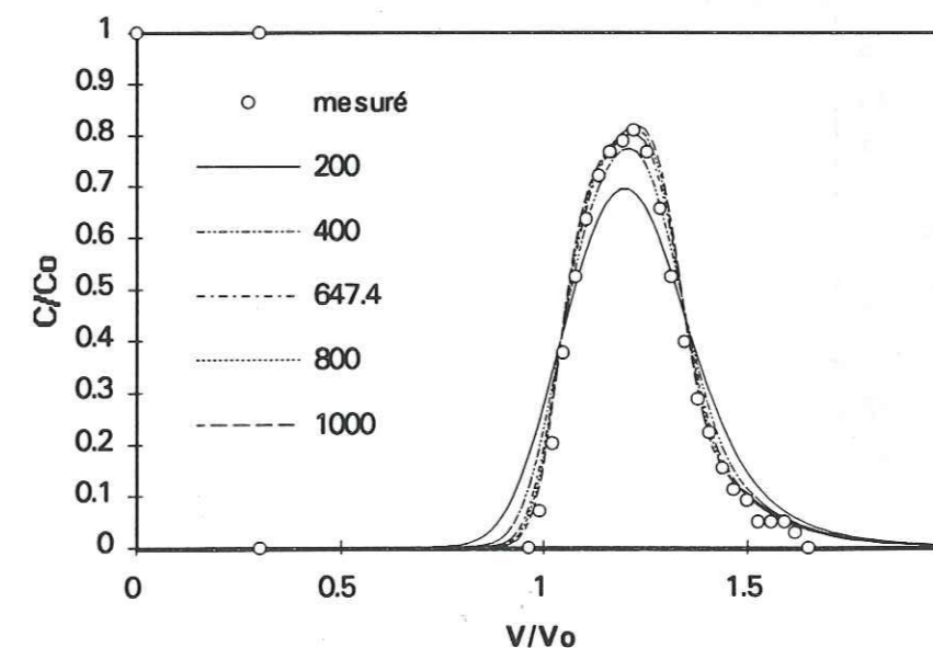
Figure 4.39 - Influence de la valeur du nombre de Péclet sur une courbe de sortie du PCP pour R = 1,085 ; \beta = 0,95 ; \omega = 0,5 ; \psi = 0,254 et un créneau = 0,3.
