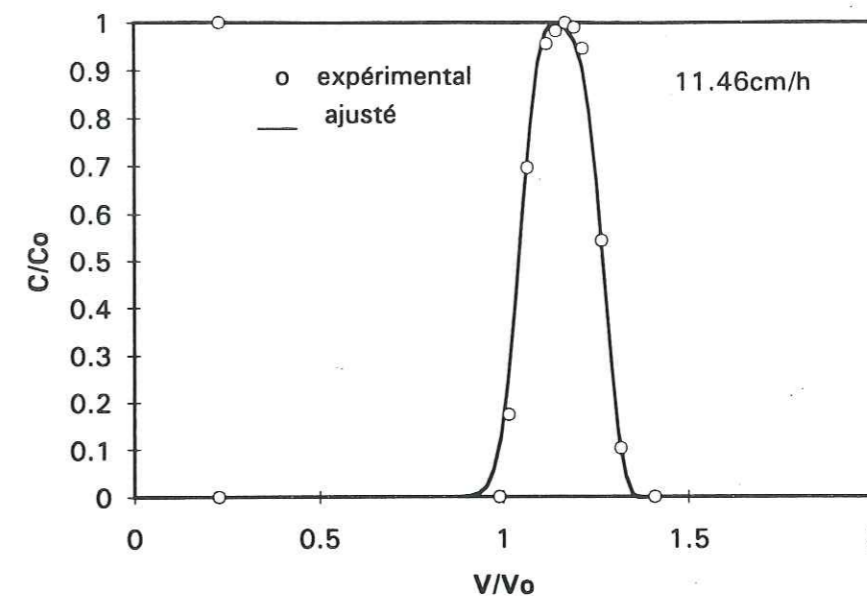
Figure 4.8 - Ajustement des paramètres sur la courbe de sortie du KCl à 11,46 cm h -1 .
