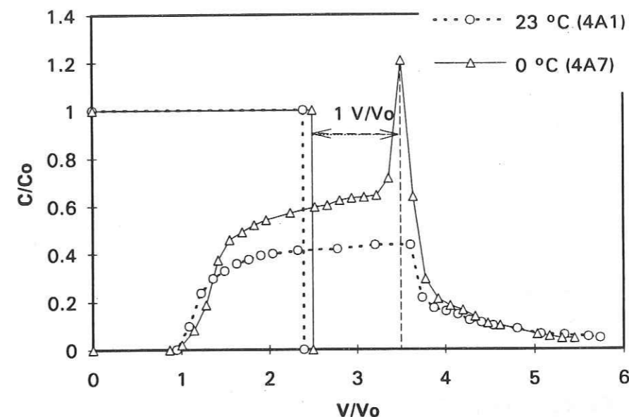
Figure 4.46 - Courbes de sortie du PCP dans la colonne de sable ensemencé avec des bactéries.
