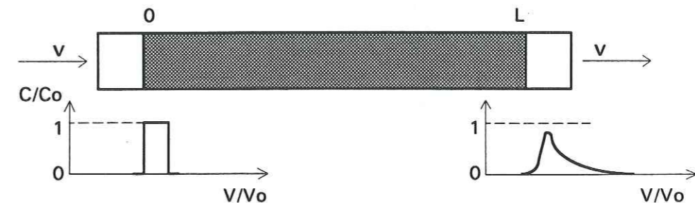
Figure 1.3 - Courbe de réponse à un créneau de soluté dans une colonne remplie d'un matériau poreux.
