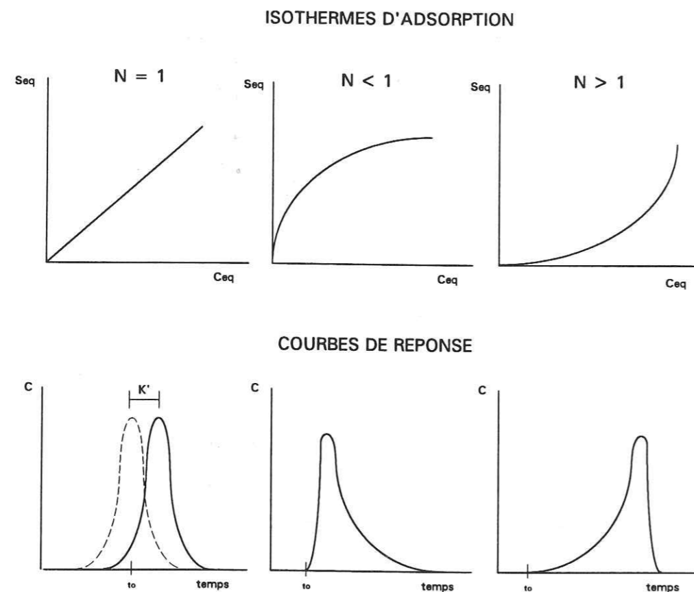
Figure 1.10 - Isothermes d'adsorption de Freundlich et courbes d'éluion respectives (d'après Schweich et Sardin, 1986).
