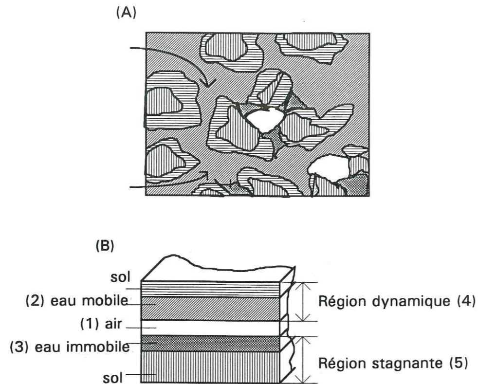
Figure 3.3 - Schéma du milieu poreux non saturé constitué d'agrégats. (A) Modèle réel. (B) Modèle simplifiée. Les hachures sur les différentes régions sont les mêmes en (A) et (B).
