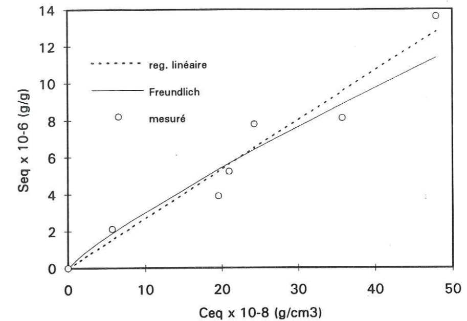
Figure 2.6 - Isotherme d'adsorption du PCP sur le sol de la Côte St André.
