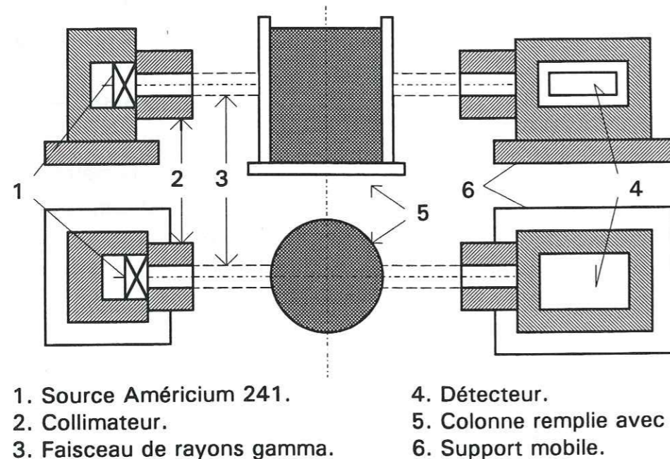
Figure 2.8 - Schéma du dispositif expérimental pour la mesure de la teneur en eau en utilisant la gammamétrie.
