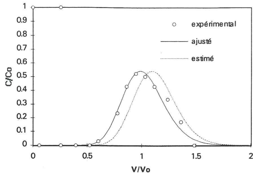
Figure 4.52 - Comparaison entre des courbes calculées avec des valeurs ajustées et estimées.
