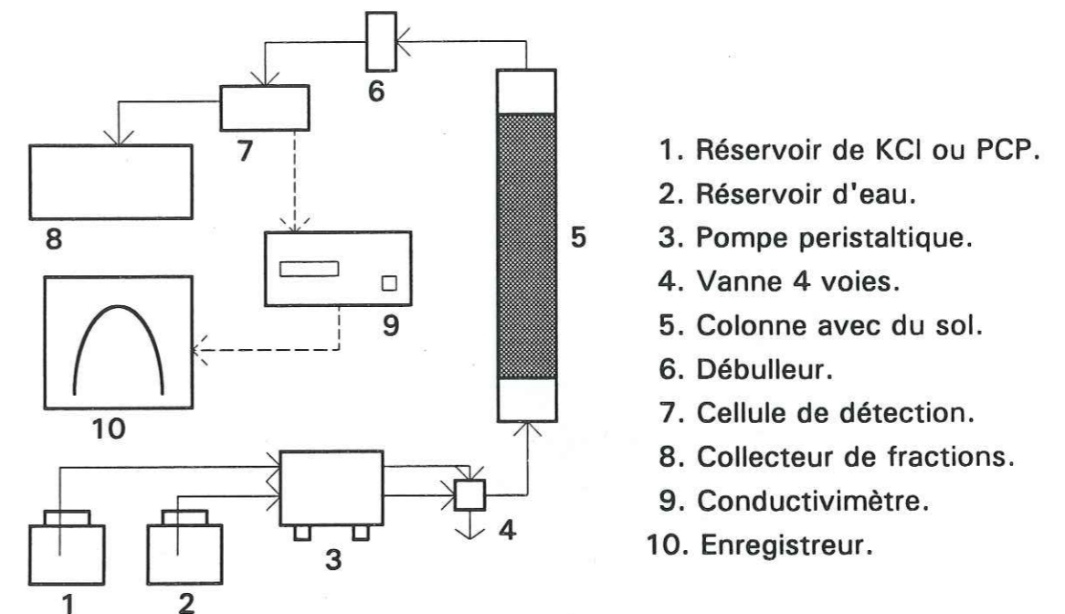
Figure 2.7 - Schéma du dispositif de transfert de solutés.
