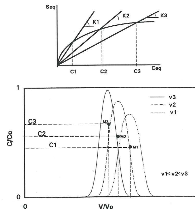
Figure 4.36 - Illustration de l'effet de la variation de vitesse sur le coefficient d'adsorption K, en considérant une isotherme non linéaire.
