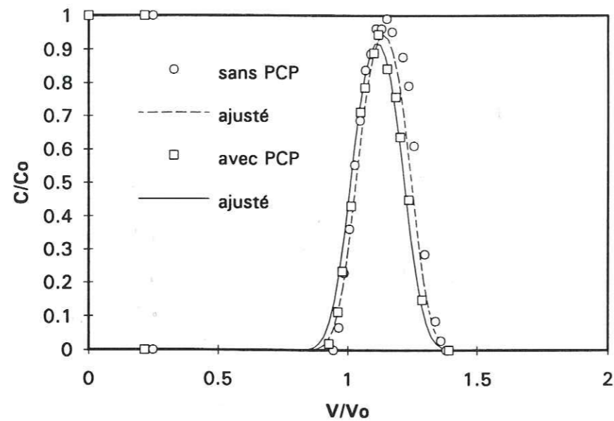
Figure 4.13 - Effet du PCP sur la courbe de sortie du KCl.
