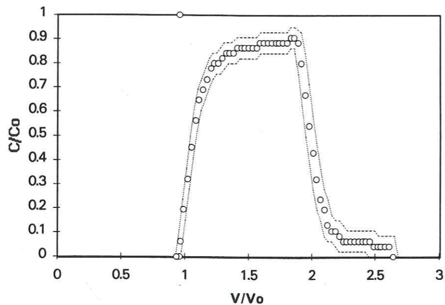
Figure 4.18 - Calcul d'erreur sur un créneau de 0.961 V/V_0 de PCP.
