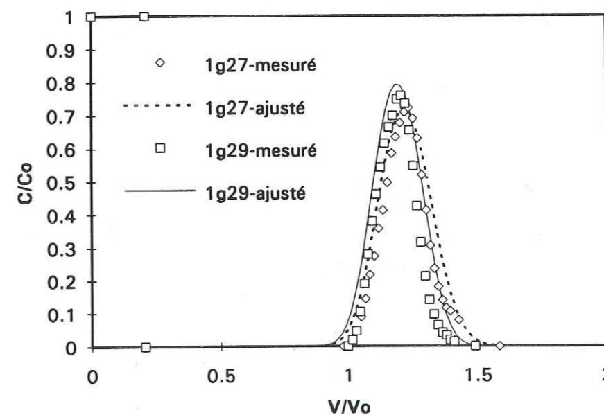
Figure 4.31 - Effet de la présence et absence de KCl dans la solution de PCP injectée.
