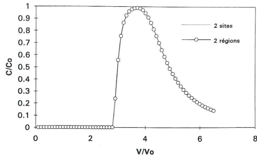
Figure 3.11 - Courbe de sortie du soluté pour N = 0,5 .
