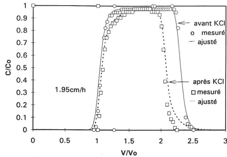
Figure 4.27 - Effet d'un premier conditionnement de la colonne en KCl sur les courbes de sortie du PCP à 1,95 \text{ cm h}^{-1} .
