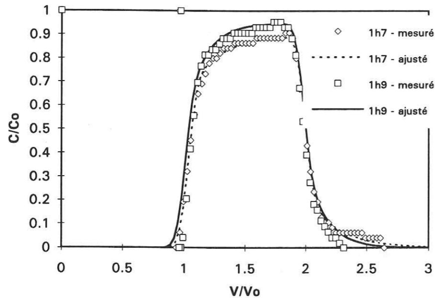
Figure 4.28 - Effet d'un conditionnement de la colonne en KCl sur les courbes de sortie du PCP à 0,64 \text{ cm h}^{-1} .
