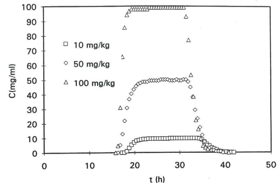
Figure 4.35 - Courbes dimensionnelles d'éluion du PCP aux concentrations de 10 \text{ mg kg}^{-1} , 50 \text{ mg kg}^{-1} et 100 \text{ mg kg}^{-1} .
