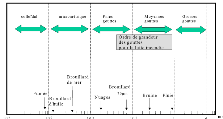
Fig.1.5 - Nomenclature des différents types de jets de gouttes dépendant de leur taille caractéristique
