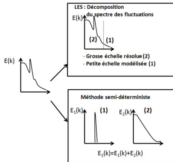
Fig.1.15 - Schématisation des méthodes LES et semi-déterministe avec une séparation du spectre en une partie modélisée et une partie résolue
