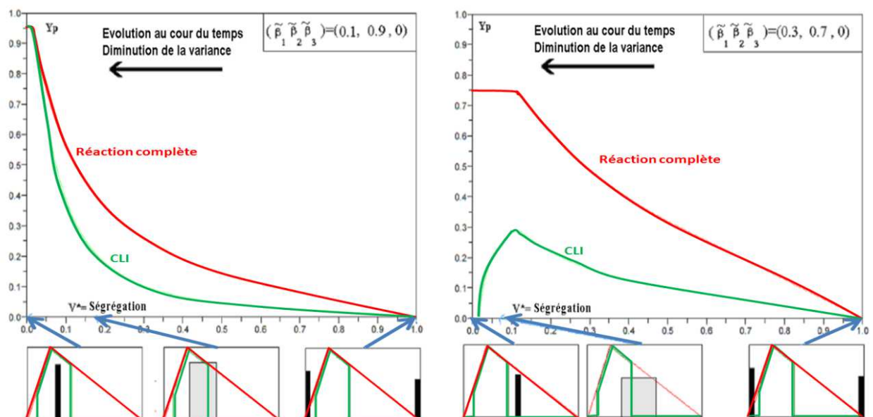
Fig.3.12 - Visualisation de l'évolution des produits moyens lors du mélange intime en prenant ou pas en compte les limites d'inflammabilité lorsque le mélange est introduit dans des proportions inflammables (a) ou non inflammables (b)
