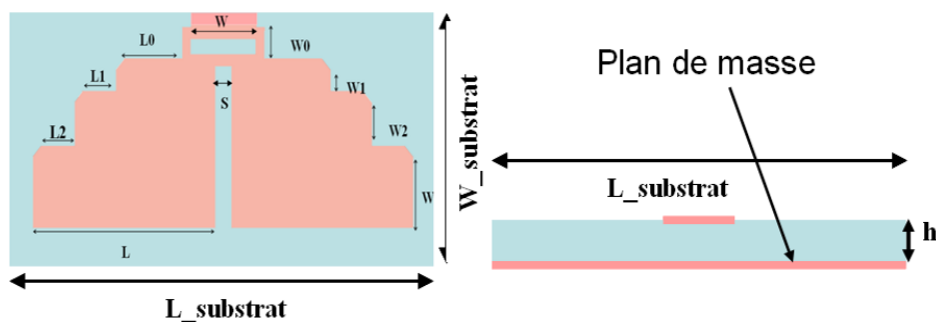
Figure 97 : Structure de l'antenne proposée (a) vue de dessus (b) vue de face
