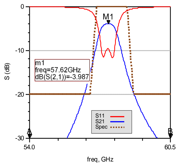
Figure 121 : Réponse de la proposition de filtre à lignes couplées d'ordre 3
