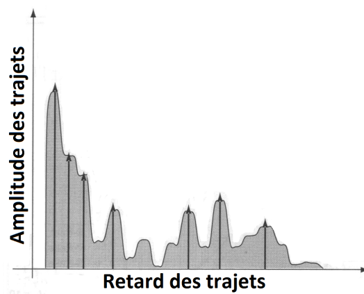
(b) S-rake
