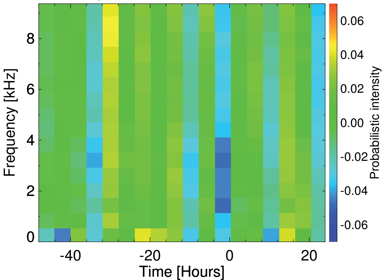
FIGURE C.21 – Spectrogram fréquence-temps de la densité de probabilité obtenu en utilisant les données électriques mesurées pendant la nuit avec des distances entre la projection du satellite au sol et l'épicentre d'un tremblement de terre inférieures à 440 km. Seuls les tremblements de terre de magnitude supérieure ou égale à 5,0, et des données mesurées pour des latitudes géographiques inférieures ou égales à 24 degrés ont été traitées.
