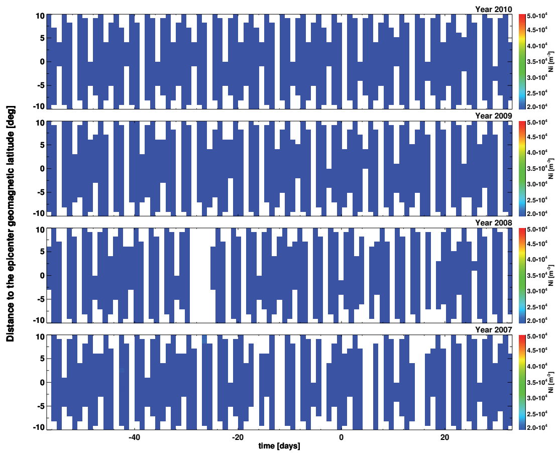
FIGURE B.2 – Représentation des données enregistrées pendant 4 ans au voisinage du point (35,85°S;110,50°W). L'échelle des couleurs est la même que pour la figure B.1.
