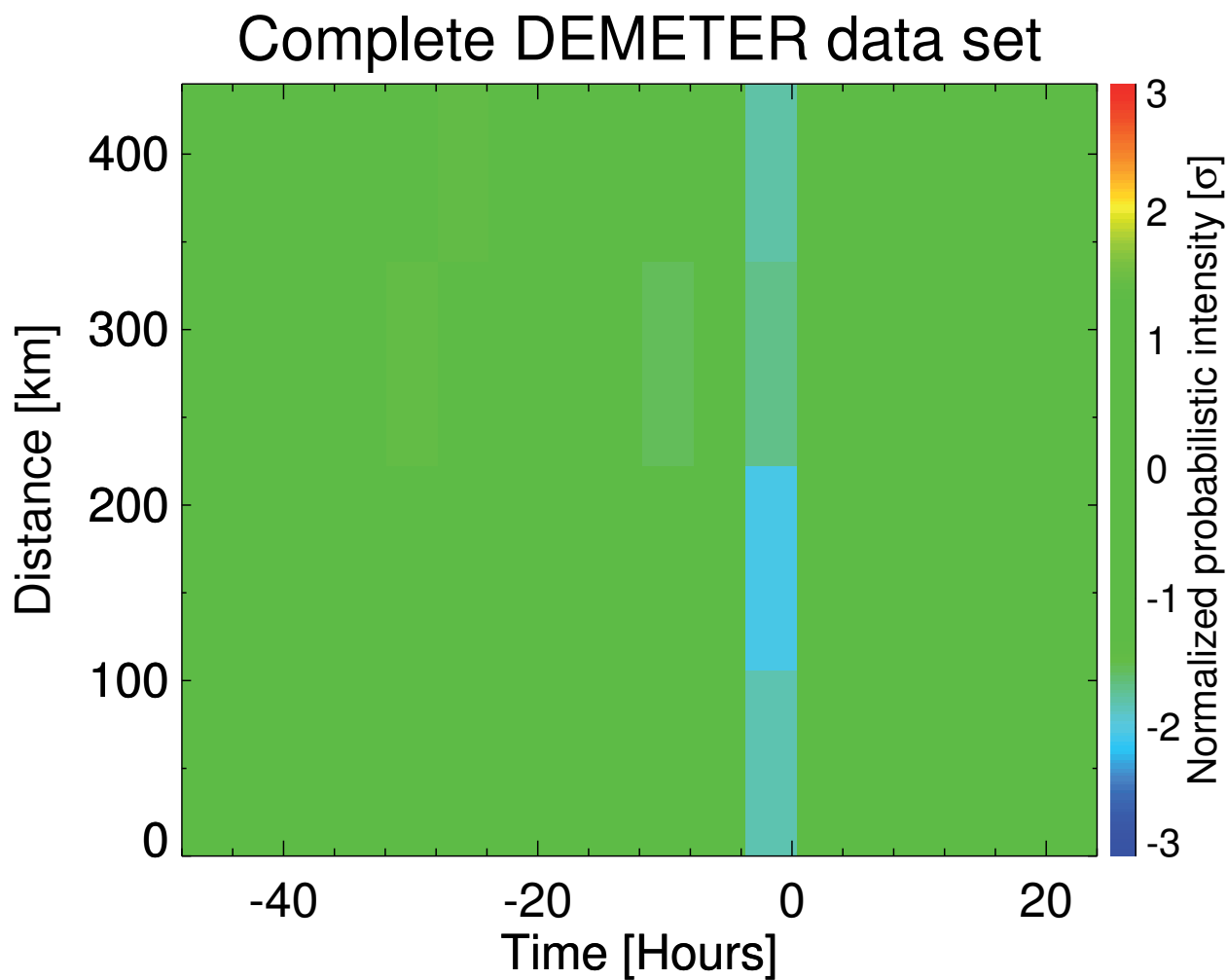
FIGURE 4.9 – Densité de probabilité obtenue en utilisant les données électriques mesurées pendant la nuit en fonction de la distance à l'épicentre et du temps relatif au choc principal. Seuls les tremblements de terre de magnitude supérieure à 5.0 ont été pris en compte. La bande de fréquence 1620-1721 Hz a été utilisée.
