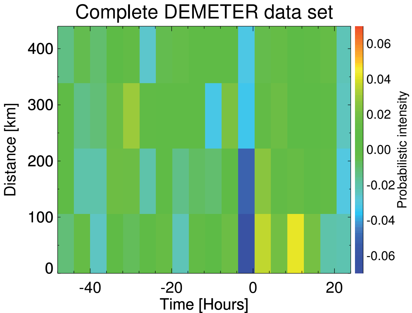
FIGURE C.4 – Spectrogramme fréquence-temps de la densité de probabilité obtenu en utilisant les données électriques mesurées pendant la nuit pour des distances entre la projection du satellite au sol et l'épicentre d'un tremblement de terre inférieures à 440 km. Seuls les tremblements de terre de magnitude supérieure ou égale à 5.0 ont été utilisés.
