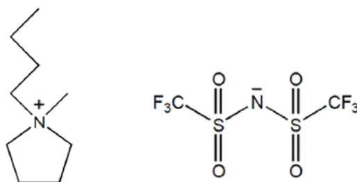
Figure 4 : Le cation \text{BMP}^+ (à gauche) et l'anion \text{TFSA}^- (à droite)
