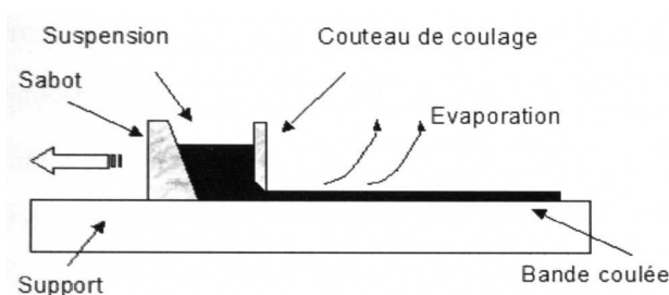
Figure 105 : Représentation schématique de l'enduction d'une électrode
