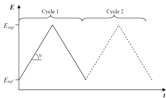
Figure 108 : Programmation du potentiel en fonction du temps en voltammétrie cyclique
