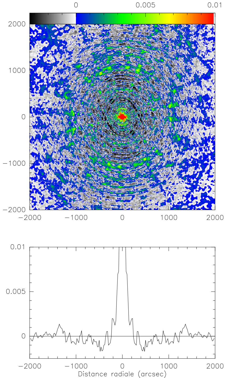
FIGURE 3.5: En haut : Image de la réponse impulsionnelle normalisée du VLA pour les observations du H \alpha dans M33, les valeurs sont fortement écrêtées pour mettre en avant les lobes secondaires et le bol négatif autour du pic principal. En bas : moyenne radiale de la réponse impulsionnelle B_{dirty} . Pour les rayons compris entre 200'' et 1200'', la réponse impulsionnelle est en moyenne inférieure à zéro.
