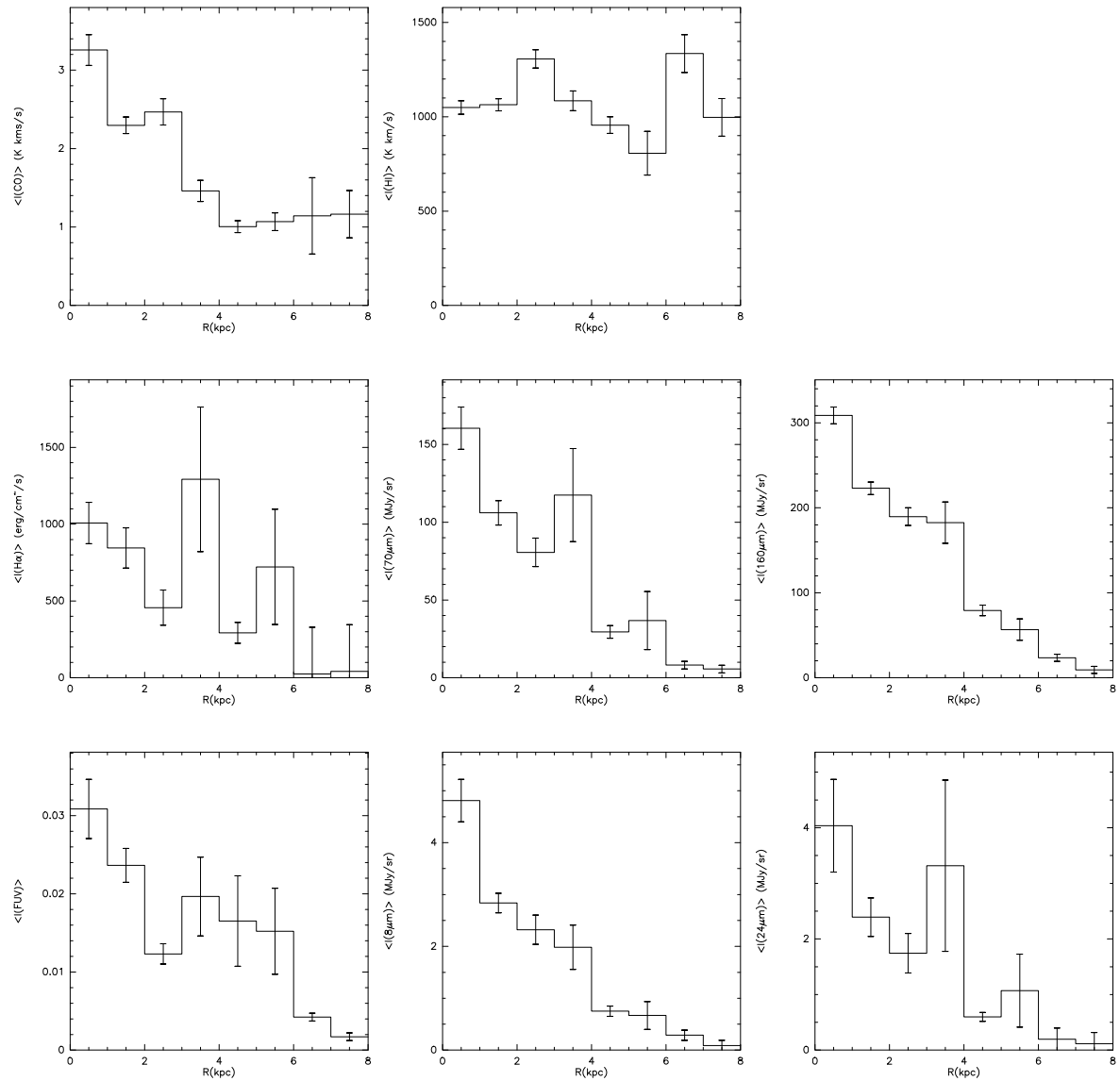
FIGURE 7.10: Variation de l'intensité des nuages en fonction du rayon pour différentes bandes. Dans l'ordre lexicographique : CO, HI, H \alpha , 70 \mu\text{m} , 160 \mu\text{m} , FUV, 8 \mu\text{m} , 24 \mu\text{m} .
