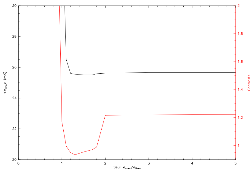
FIGURE 2.7: Graphique de la valeur moyenne du bruit et du contraste de la carte de bruit, après construction du cube, en fonction du seuil de coupure pour le rapport \sigma_{\text{spec}}/\sigma_{\text{theo}} .
