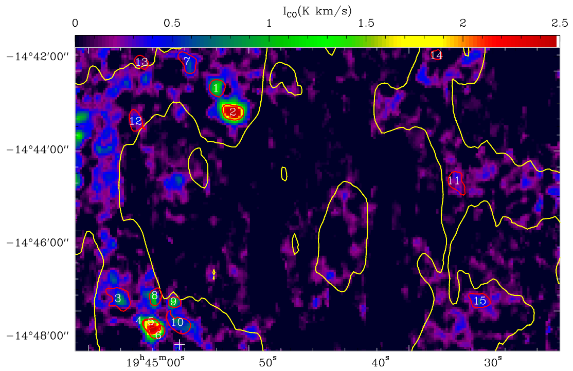
FIGURE 2.10: Carte de l'intensité intégrée CO(2-1) de NGC6822 en \text{K km s}^{-1} . Les contours jaunes correspondent à l'émission HI avec un niveau N(\text{HI}) = 1 \cdot 10^{21} \text{ cm}^{-2} , les rouges aux contours à mi-hauteur des nuages moléculaires identifiés dont l'étude détaillée est présentée au chapitre 6. La croix blanche est la position des offsets (0,0).
