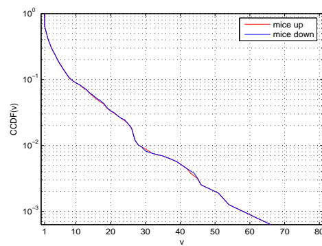
FIG. 1.19 – CCDF du nombre de souris par adresse externe
