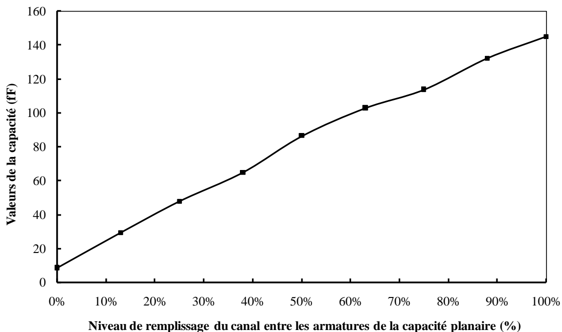
Figure II-14 : Variation de la capacité en fonction du niveau de remplissage du canal.
