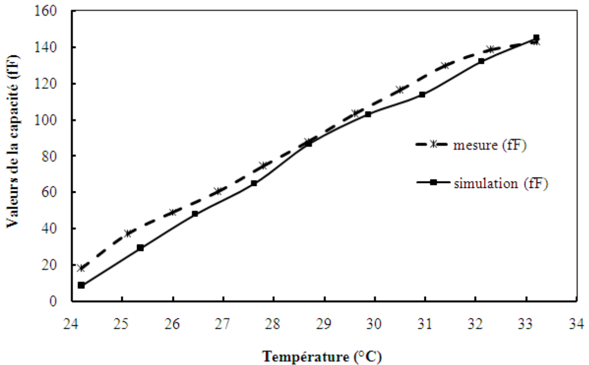
Figure II-28 : La valeur de la capacité mesurée et simulée en fonction de la température appliquée.
