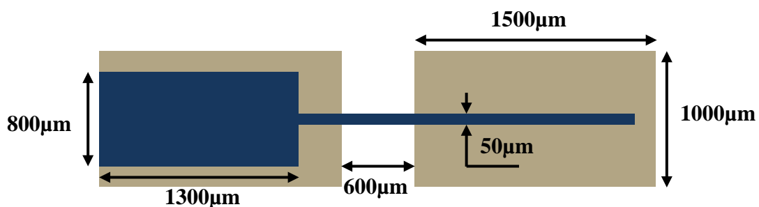
Figure III-12 : Dimensions du dipôle et de la microstructure fluïdique
