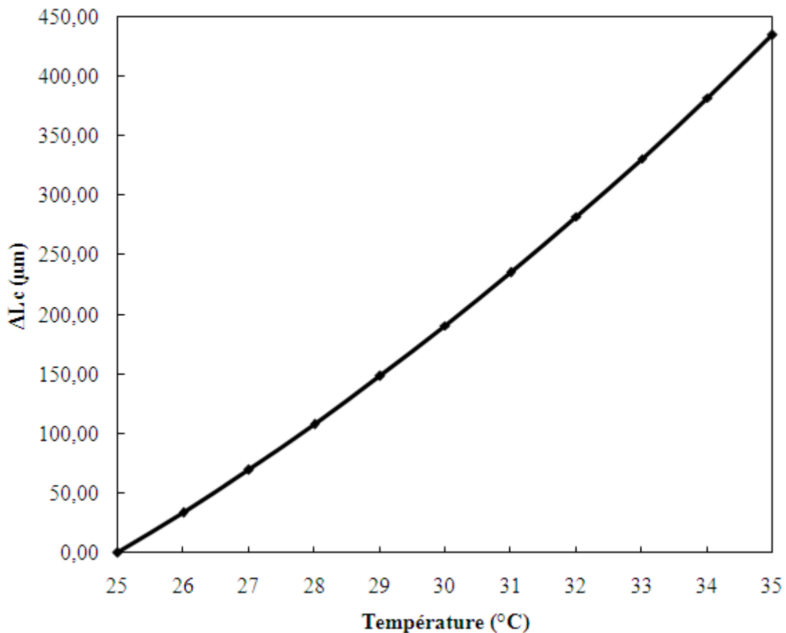
Figure II-9 : Simulation de la variation de la position du front d'eau dans le canal en fonction de la température ( V_0 = 2.10^9 \mu\text{m}^3 )
