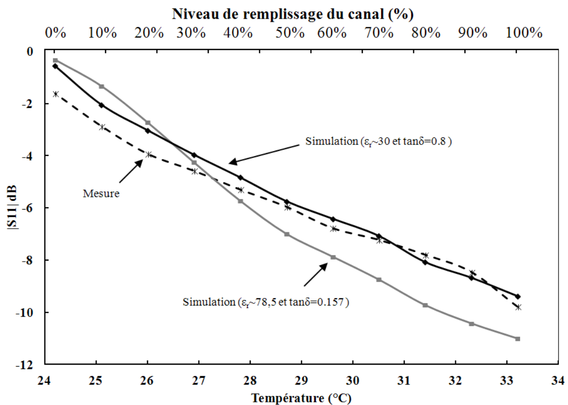
Figure II-26 : Coefficient de réflexion mesuré et simulé de la capacité en fonction de la température à la fréquence de 29,75GHz.
