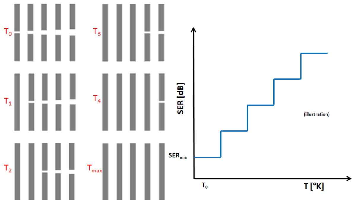
Figure III-2 : Principe du capteur de température avec 5 dipôles T_0 : aucun dipôles court-circuités, T_{max} : tous dipôles court-circuités
