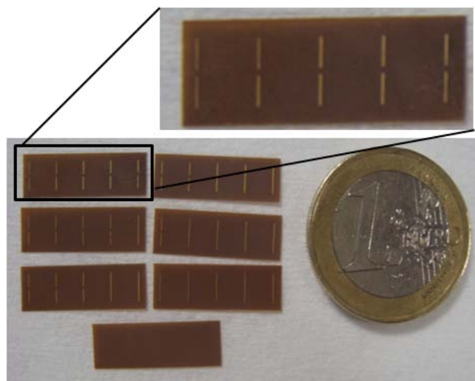
Figure III-7 : Réseau de dipôles réalisé sur kapton
