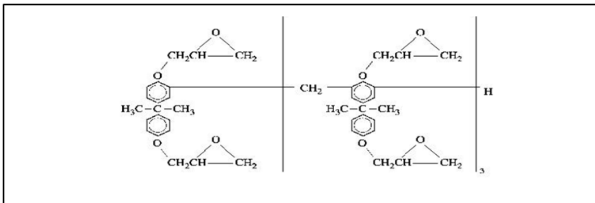
Figure II- 18: Structure chimique de la résine SU-8 (glycidyl-ether-bisphenol-A novolac).
