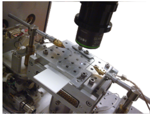
(c) Détails des doigts de la platine sous un système optique par réflexion.
