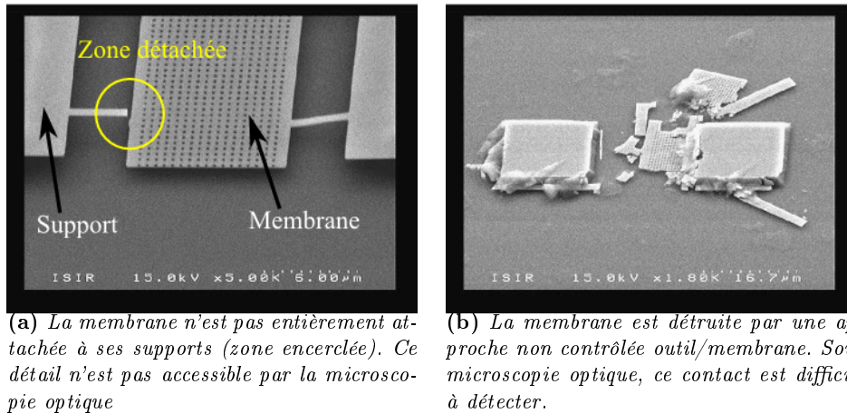
Figure 4.9 - Deux limites rencontrées lors de la caractérisation sous optique. Échantillons imagés au MEB.
