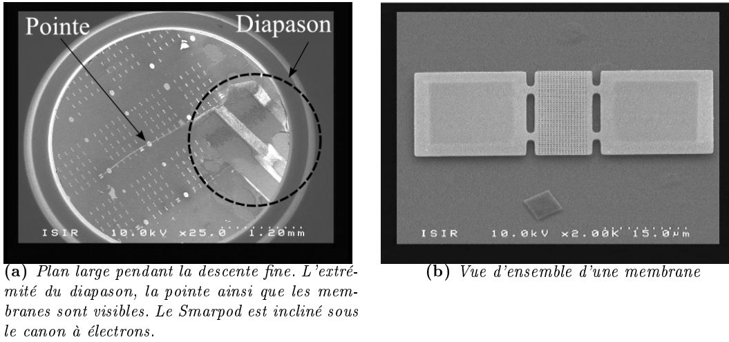
Figure 4.11 - Descente du capteur vers les échantillons
