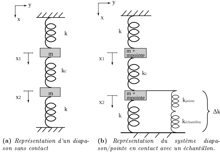
Figure 4.4 - Représentation de diapason par le modèle de [Castellanos-Gomez 09]. Les deux branches sont considérées de raideur ( k ) et de masse identiques ( m ou m + m_{\text{pointe}} ) avec une force de rappel ( k_c ) entre les deux masses.
