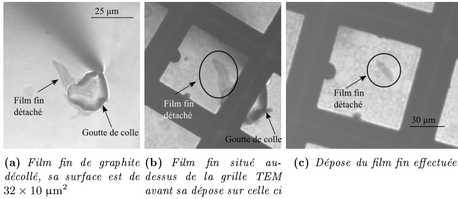
Figure 2.13 - Transfert de film fin sur une grille TEM. La surface du film fin déposé sur la grille est de 4.8 \times 11 \mu\text{m}^2 soit environ 15 % de la surface du film détaché.
