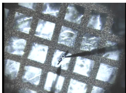
(b) Dépôt sur une seconde grille TEM du film détaché.
