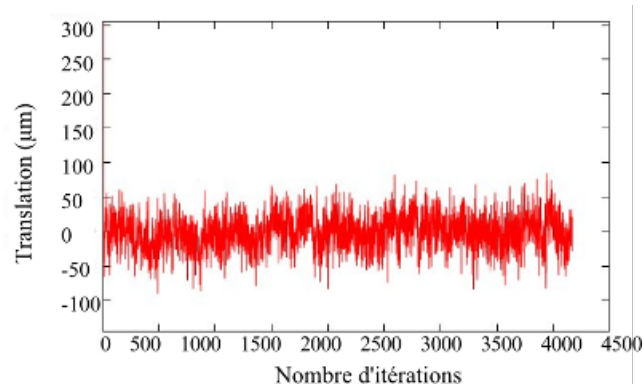
Figure 3.16 - Bruit statique de l'algorithme. L'algorithme fonctionne pendant 4000 itérations en statique à la position d'origine ( 0\text{ }\mu\text{m} ) de la platine. La résolution du système en statique est de 50\text{ }\mu\text{m} .
