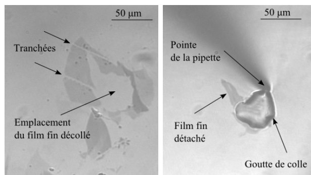
(a) Les tranchées ont été créées sur la membrane sectionnée, pour contrôler son déchirement (b) La pipette avec la membrane détachée.
