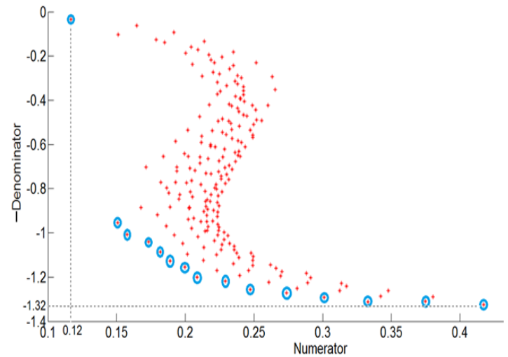
Fig. 22. Pareto front.
