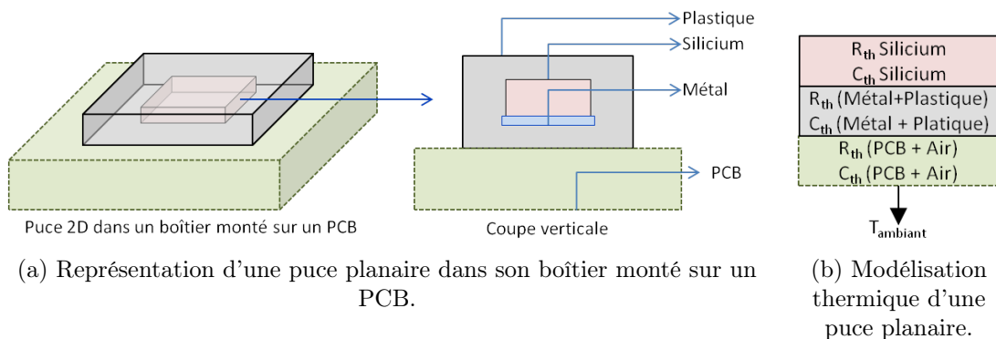
FIGURE 7.10 – Représentation et modélisation d'une puce planeaire.
