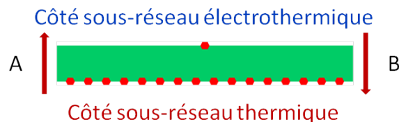
FIGURE 7.19 – Symbole d'une instance de couplage : distribution du flux de chaleur vers 16 nœuds du réseau thermique.
