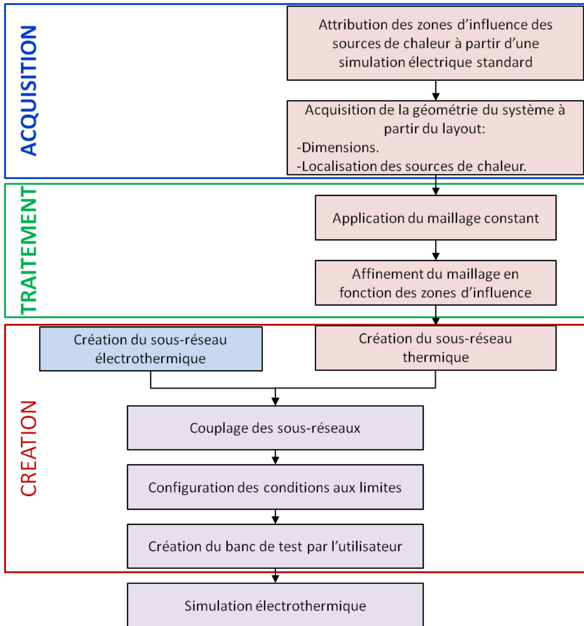
FIGURE 7.23 – Organigramme de la procédure complète nécessaire à la simulation électrothermique.
