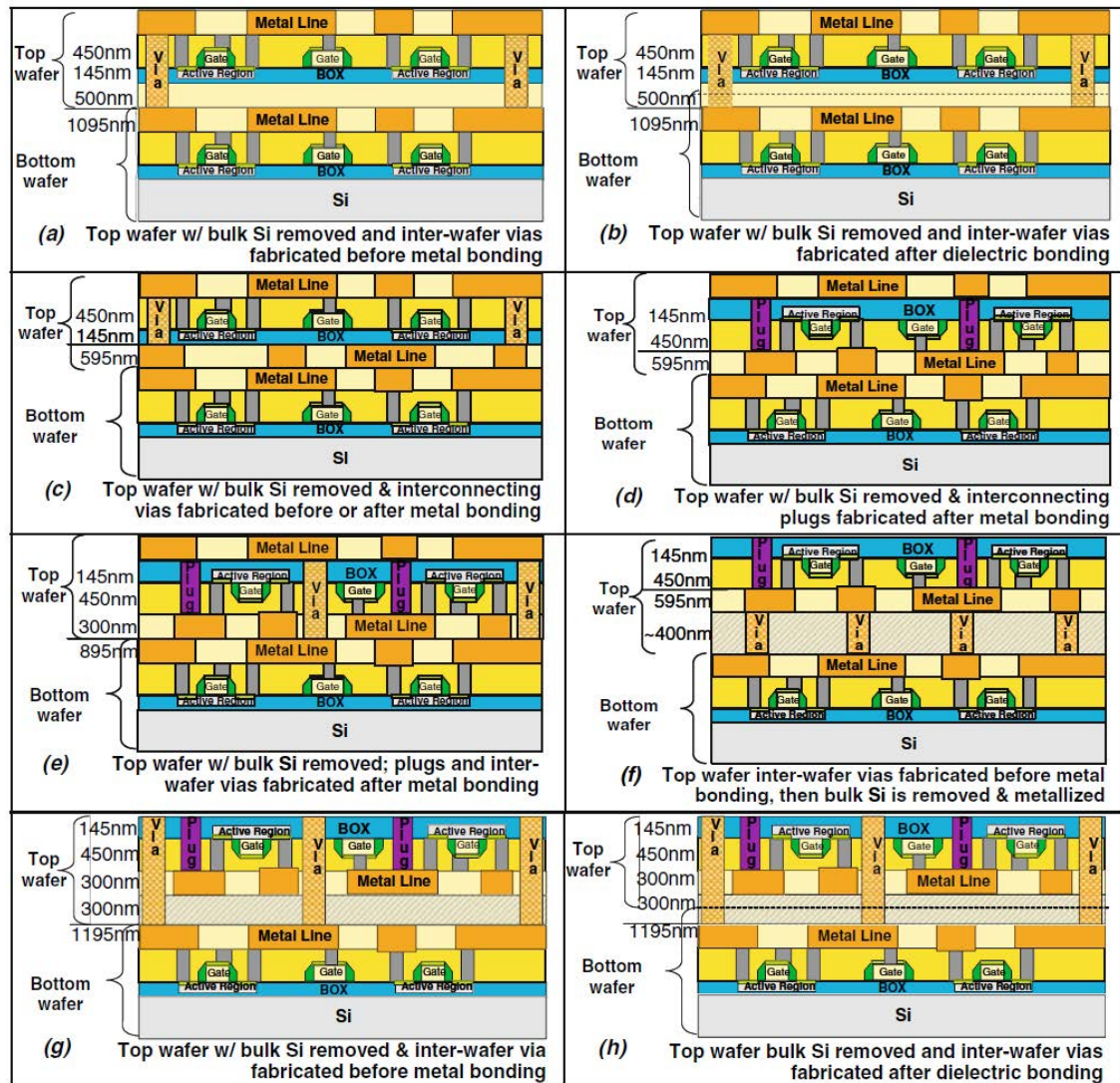
FIGURE 2.5 – Vue en coupe des différentes configurations d’intégrations possibles [8] (a)–(c) configuration “face-to-back”. (d)–(h) configuration “face-to-face”.
