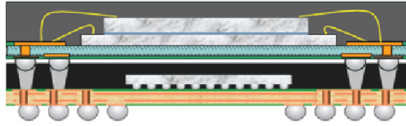
FIGURE 2.2 – Schéma en coupe d'un système PoP [2].
