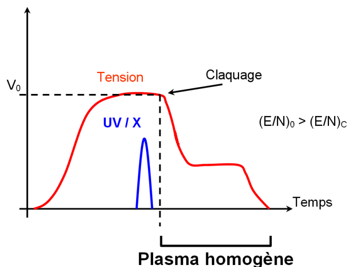
Figure 14 Principe du photo déclenchement
