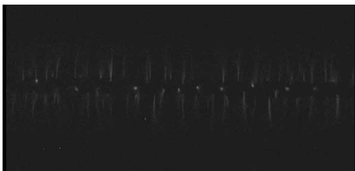
Figure 126 Visualisation d'une décharge produite par le réacteur tige-cylindre pour un débit de 500 cc/ min d'un mélange azote-oxygène à 20% d'oxygène (Flash Cam - objectif UV) avec une fréquence d'impulsion de 100 Hz
