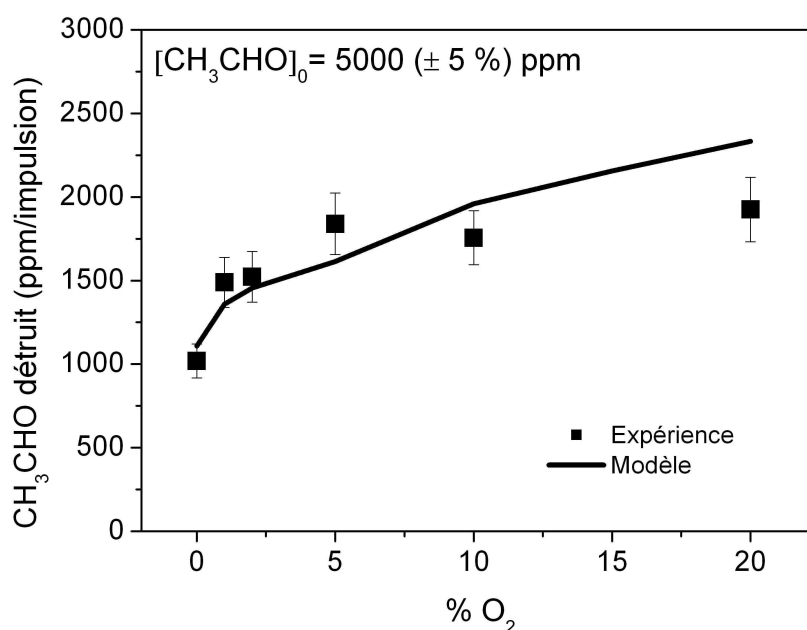
Figure 111 Destruction de l'acétaldéhyde dans le volume de décharge en fonction du pourcentage d'oxygène pour C_0 = 5000 ppm.
