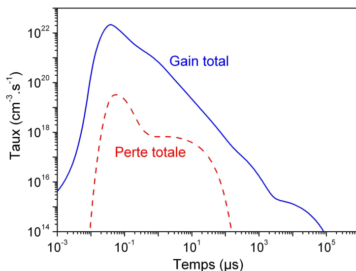
Figure 71 Perte totale et gain total d'hydrogène C_0 = 5000 ppm
