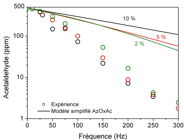
Figure 157 Concentration d'acétaldéhyde en sortie du réacteur pour des mélanges N_2/O_2/CH_3CHO 2 %, 5% et 10% d'oxygène et 480 ppm d'acétaldéhyde pour la DBD cylindrique
