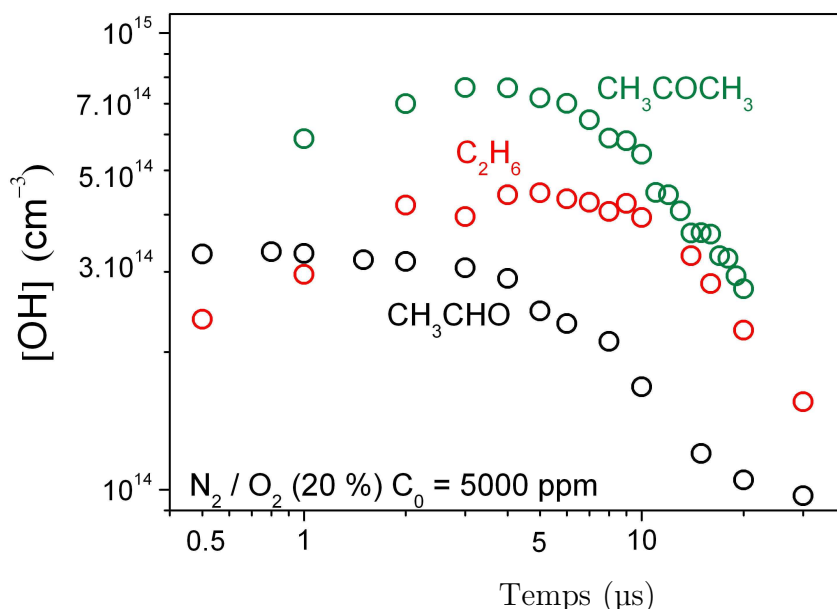
Figure 109 Comparaison de la concentration de radical hydroxyle à 5000 ppm et à 20 % d'oxygène pour l'éthane, l'acétone, et l'acétaldéhyde
