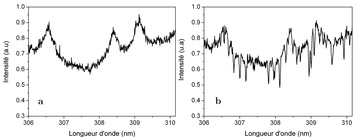
Figure 41 (a) Ligne de base (sans absorption) \text{N}_2 pur (b) Raies du radical OH observées dans un mélange \text{N}_2/\text{O}_2/\text{CH}_3\text{CHO} à 0.5 % d'acétaldéhyde et 20 % d'oxygène à 1 \mu\text{s} après l'impulsion de courant
