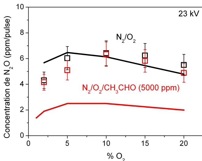
Figure 94 : Concentration de N_2O dans les mélanges N_2/O_2/CH_3CHO et N_2/O_2 à 23 kV (15 % barre d'erreur) et comparaison aux prédictions du modèle (trait plein)
