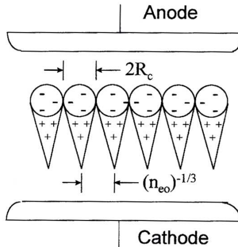
Figure 13 Densité minimale de pré-ionisation pour le développement homogène du plasma [59]
