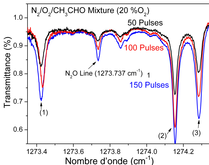
Figure 39 Spectre d'absorption après 50, 100, 150 impulsions - Pression dans la cellule : 100 Torr ( 1273.737\text{ cm}^{-1} ) N_2/O_2/CH_3CHO 10 % O_2 Température QCL : 14.6^\circ\text{C} (exsitu)
