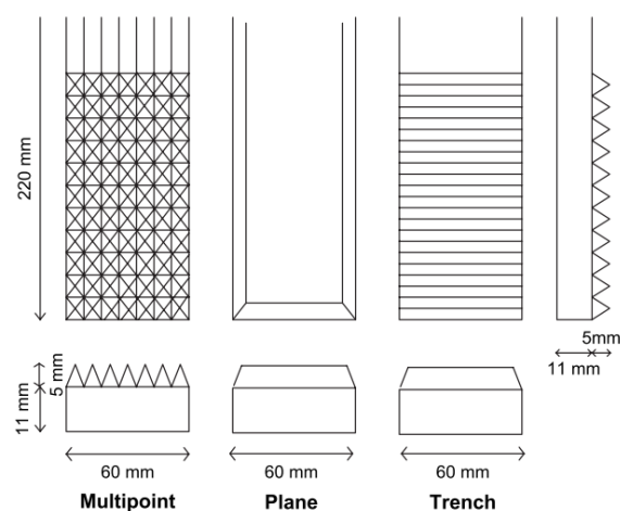
Figure 30 Différentes géométries d'électrodes utilisées par Takaki et al. [151]
