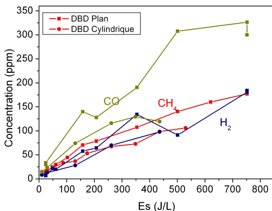
Figure 147 Concentrations de CO , CH_4 et H_2 en sortie des décharges DBD
