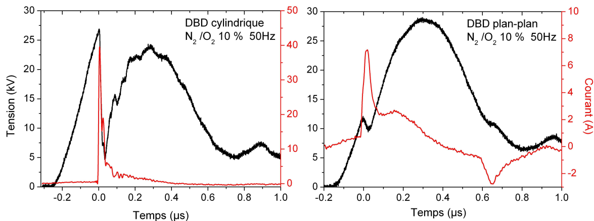
Figure 46 Signal de tension et de courant pour une décharge à 10% d'oxygène pour la DBD plan et la cylindrique (échantillonnage à 5 GS/s par canal, Fréquence = 50 Hz)
