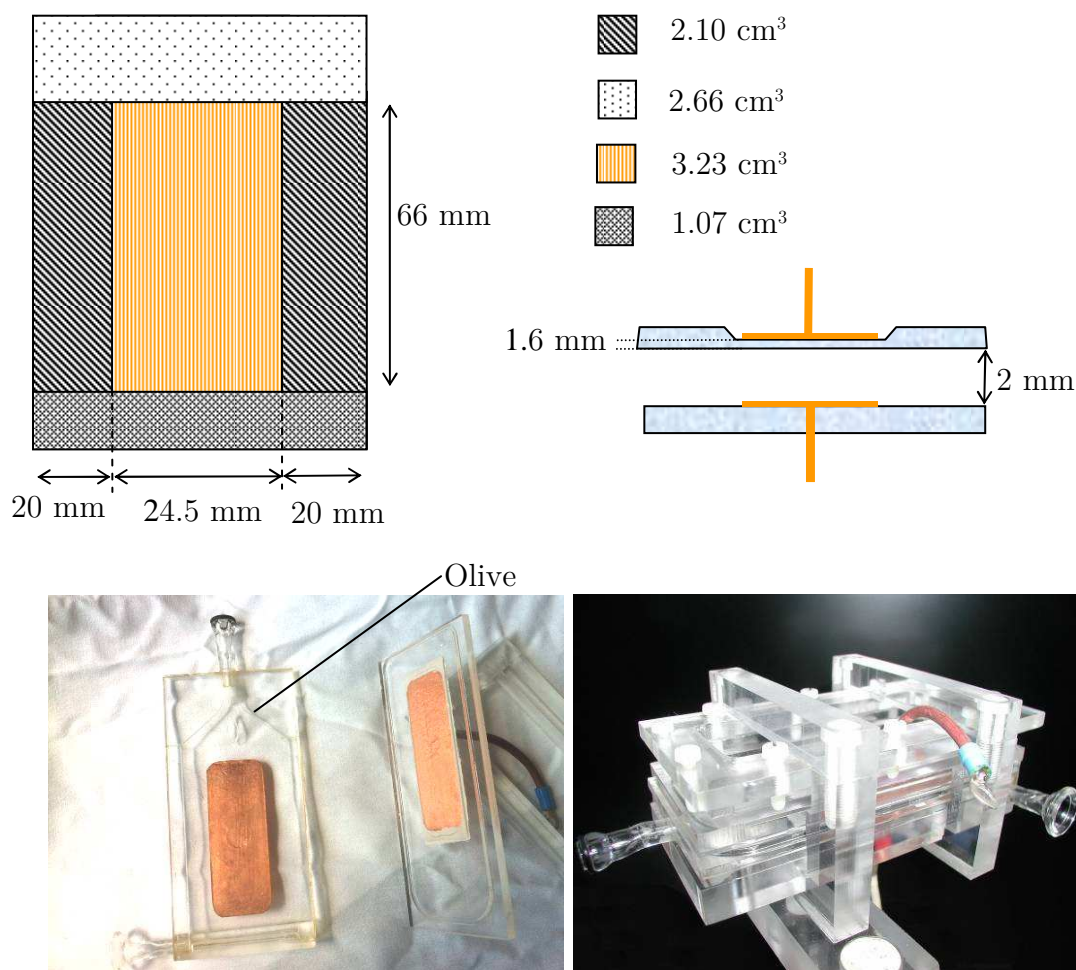
Figure 44 Schéma représentatif des longueurs remarquables dans la DBD Plan-plan – DBD plan-plan en images
