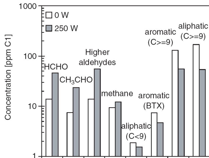
Figure 10 Sous-produits de conversion de fumée de véhicule diesel par décharges électriques impulsionnelles [45]
