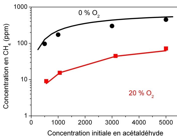
Figure 114 Concentration de méthane mesurée dans les mélanges à 0% et à 20 % d'oxygène pour différentes concentrations initiales en acétaldéhyde dans le volume de la décharge (Mesures : Points – Prédictions du modèle : traits)
