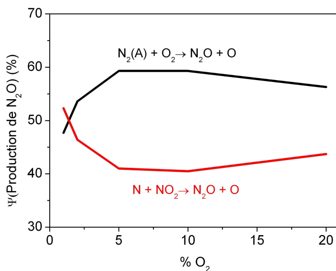
Figure 92 Parts de la production de N 2 O en fonction de la concentration d'oxygène
