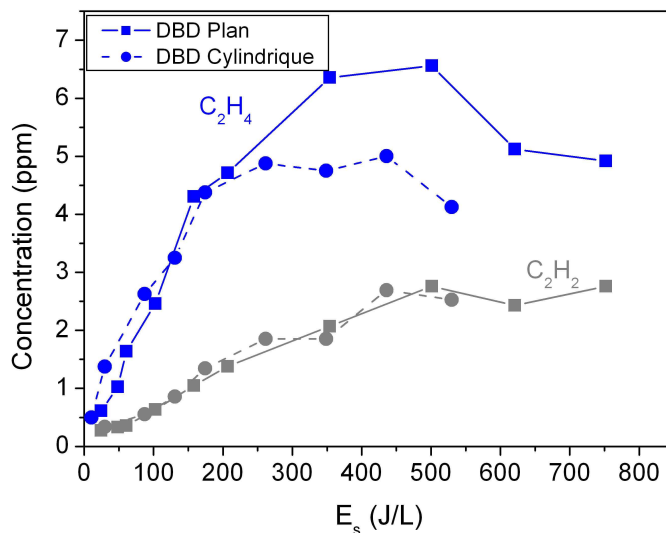
Figure 145 Evolution de la concentration d'éthène et d'acétylène en fonction de l'énergie déposée pour les réacteurs Plan et Cyindrique dans un mélange N_2/CH_3CHO C_0 = 480 ppm
