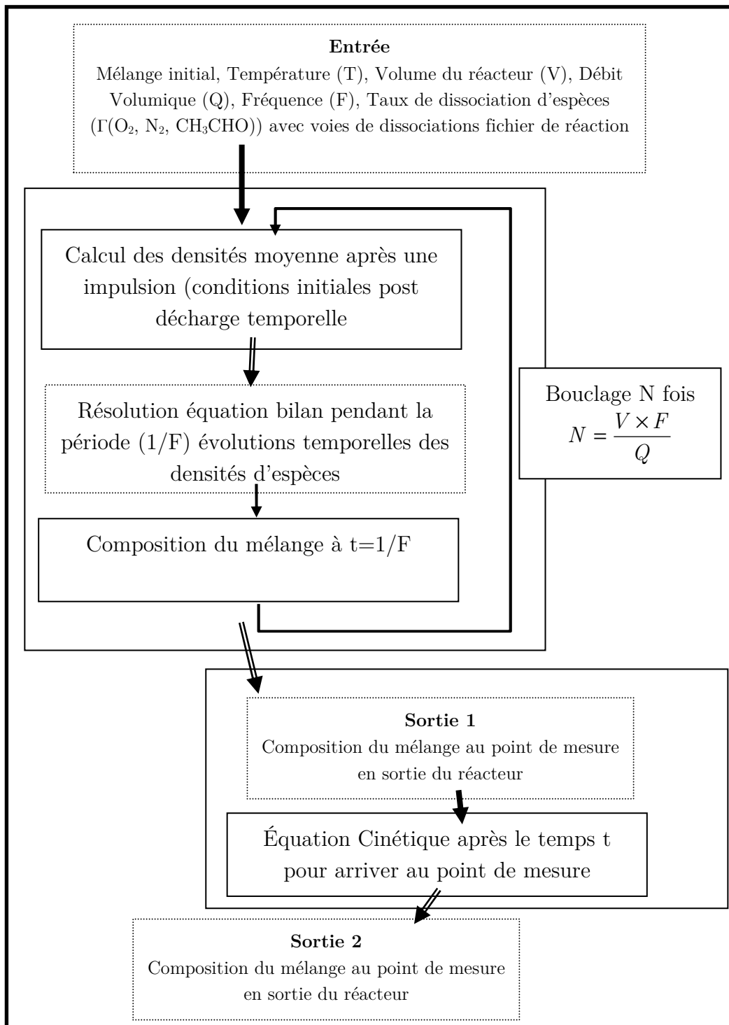
Figure 60 Schéma du modèle pour la simulation de la réactivité des DBD
