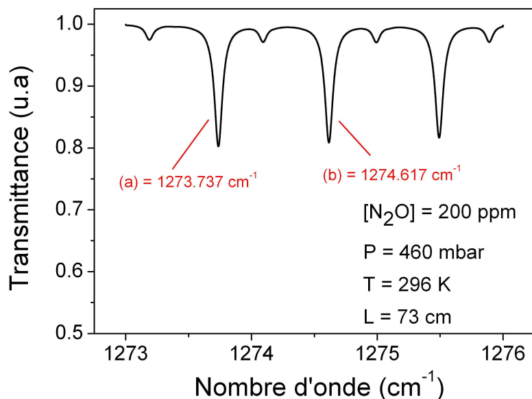
Figure 38 Simulation des raies de N_2O par le logiciel TDL Wintel utilisant la base de données HITRAN (200 ppm – Longueur d'absorption 73 cm – 460 mbar )
