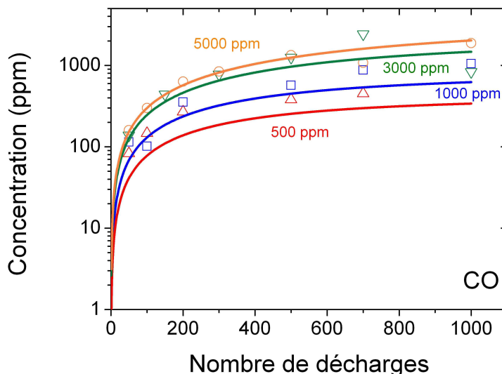
Figure 86 Evolution de la concentration du monoxyde de carbone dans le volume total du réacteur UV 510 et comparaison aux prédictions du modèle en boucle
