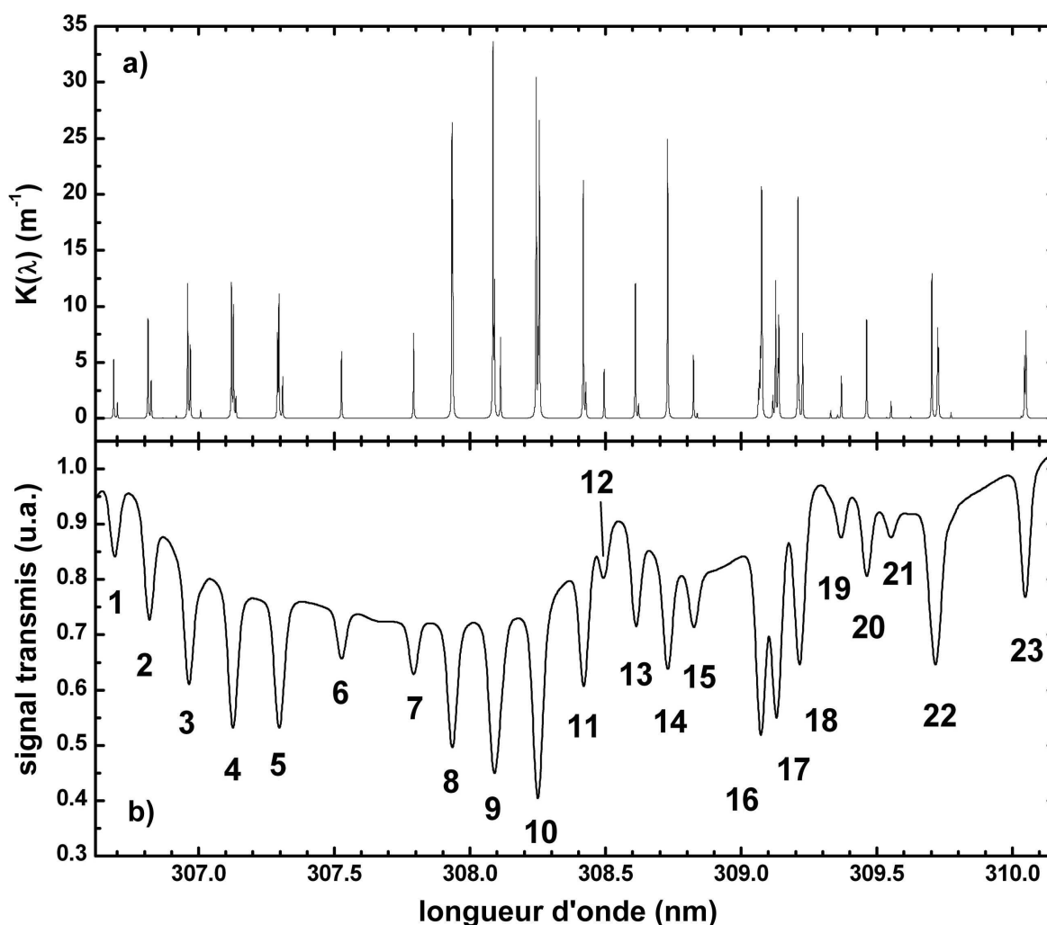
Figure 166 : Simulation de spectres. a) Coefficient d'absorption calculé en supposant une densité totale de OH de 1.0 \times 10^{15} \text{ cm}^{-3} et une température (rotation et translation) de 350 K. b) Spectre transmis calculé.
