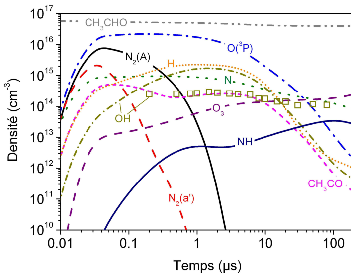
Figure 104 Prédictions du modèle pour quelques espèces au cours de la post décharges et densité de OH mesurée pour 5% d'oxygène, 5000 ppm d'acétaldéhyde, et 4.6 J par impulsion
