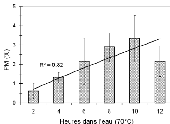
Fig.0.8. Pertes de masse (PM%) des échantillons soumis à des traitements à l'eau chaude (70 °C). N °: 5 pour chaque intervalle de temps: 5 \times 6 = 30 au total.
