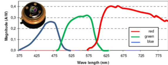
[Fig 2.8] sensibilité spectrale du MCS2AT
