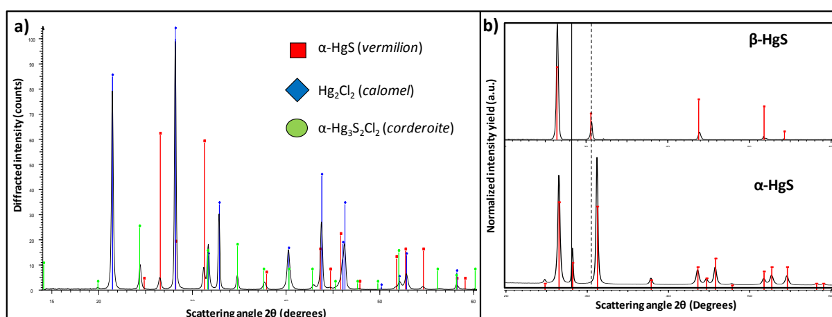
Figure 1.14.: a) Diffractogram showing different phases (vermilion \alpha\text{-HgS} –Prolabo-, calomel \text{Hg}_2\text{Cl}_2 –Aldrich- and corderoite \alpha\text{-Hg}_3\text{S}_2\text{Cl}_2 –Gallerie minéralogique de l’Ecole des Mines); b) Comparison of cinnabar ( \alpha\text{-HgS} , Gallerie minéralogique de l’Ecole des Mines) and metacinnabar ( \beta\text{-HgS} , Gallerie minéralogique de Jussieu) diffractograms.
