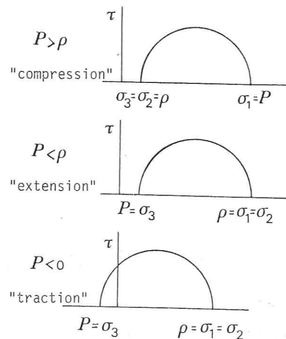
— Schema de principe de l'essai triaxial.
