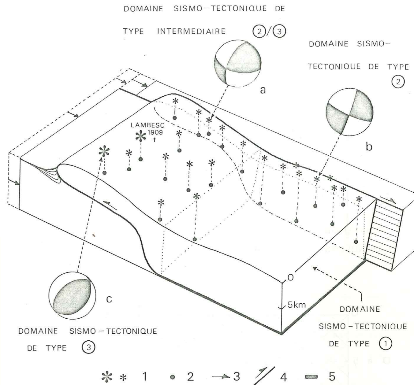
FIGURE 55 : Représentation schématique d'une déformation compressive décrochante (type D) et relation avec la sismicité. 1-Epicentre. 2-Hypocentre. 3-Direction de raccourcissement. 4-Accident tectonique. 5-Surface de décollement. a-Mécanisme au foyer décrochant-chevauchant. b-Mécanisme au foyer décrochant. c-Mécanisme au foyer inverse.
