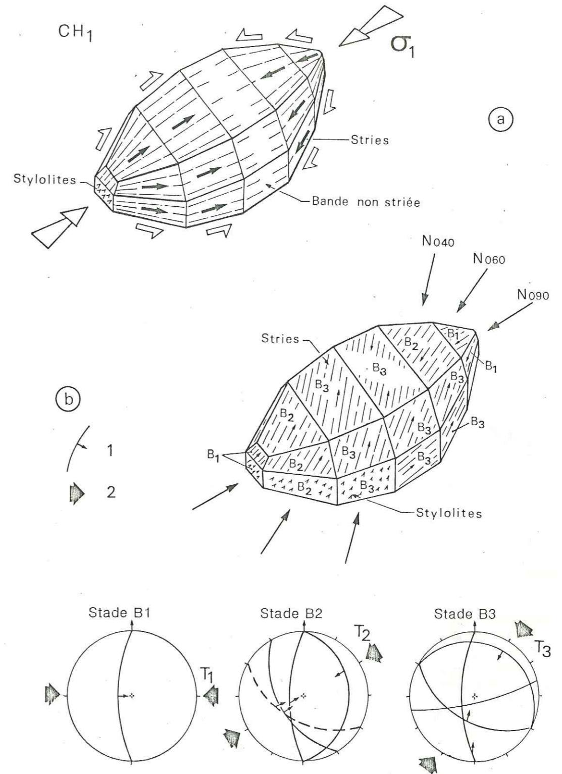
FIGURE 19 : a-Déformation d'un galet par striation (une seule direction de raccourcissement) b-Déformations successives d'un galet par striation (3 directions de raccourcissement) et représentation stéréographique de ces microdéformations. 1-Microplan de faille et sa strie. 2-Composante horizontale maximale \sigma_1 du tenseur de contraintes.
