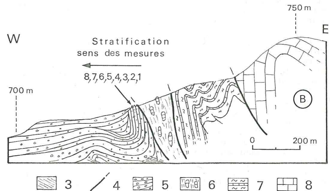
FIGURE 15 : Rotation de la stratification au cours du plissement synsédimentaire dans le flanc inverse du synclinal de St Jurs. A- Représentation stéréographique hémisphère inférieure. 1-Plan de stratification. 2-Pôles des plans. 3-Plans de schistosité. B-Coupe du front subalpin à St Jurs : localisation figure 16 (station 22). 4-Contact anormal. 5-Conglomérats mio-pliocène du Valensole. 6-Trias gypseux. 7-Calcaires et marnes Valanginiennes 8-Calcaires massifs Portlandien.
