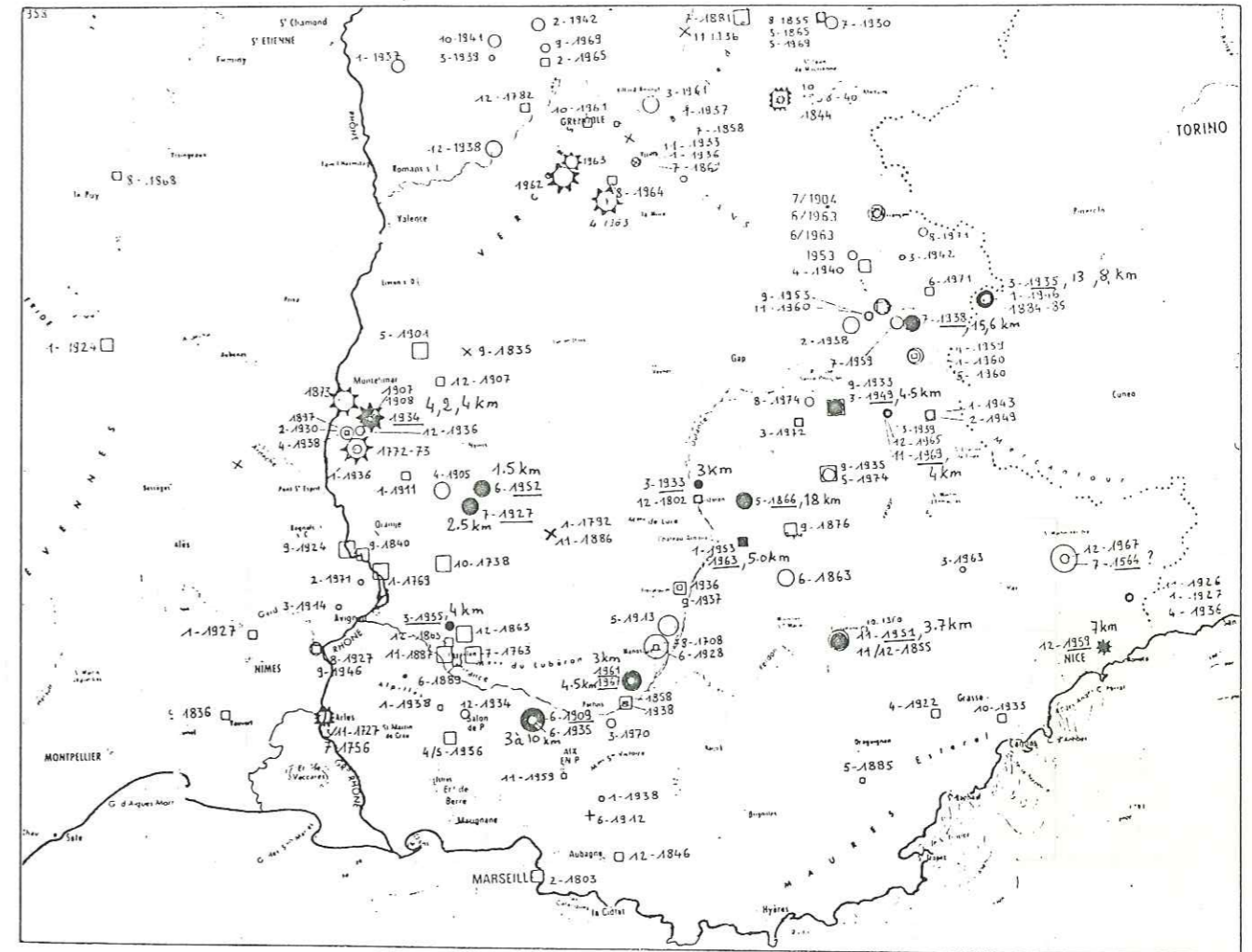
FIG : 40 CARTE D'EPICENTRES 0 10 20 30 40 50 60 70 80 90 100 D'après B.R.G.M. SGN/GTC Janvier 1978 D.S.N./B.E.R.S.S.I.N. M.REVERDY Juillet 1978
