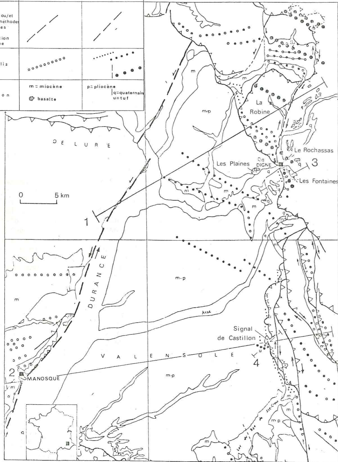
FIGURE 9a : Répartition et chronologie des déformations MIO-PLIO-PLÉISTOCENE le long du front subalpin occidental.
