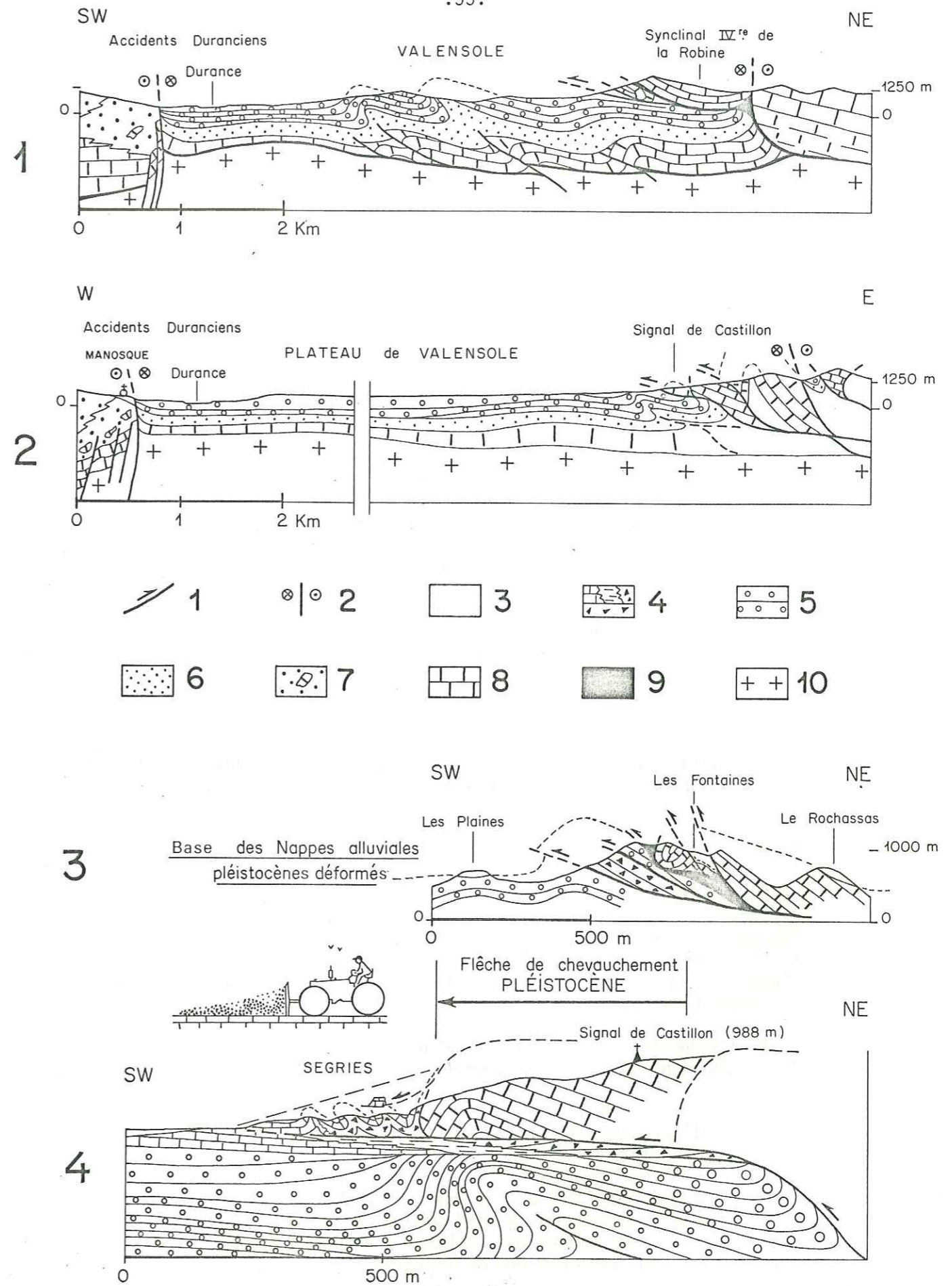
FIGURE 9b : Coupes générales (1et2) et détaillées (3et4) du front subalpin. 1-Chevauchement. 2-Décrochement. 3-Nappes alluviales pléistocène. 4-Passage latéral : calcaires lacustres, argiles et brèches d'âge pliocène terminal - pléistocène ancien (1.9 million d'années). 5-Conglomérats du Valensole mio-pliocène. 6-Formations miocène. 7-Formations oligocène. 8-Formations carbonatées mésozoïque. 9-Trias gypseux. 10-Socle paléozoïque.
