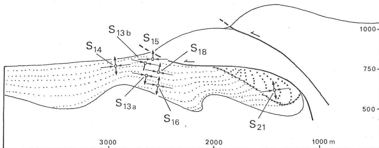
FIGURE 25 : Coupes schématiques figurant divers stades de chevauchement et leurs relations avec les axes principaux des tenseurs de contraintes.
