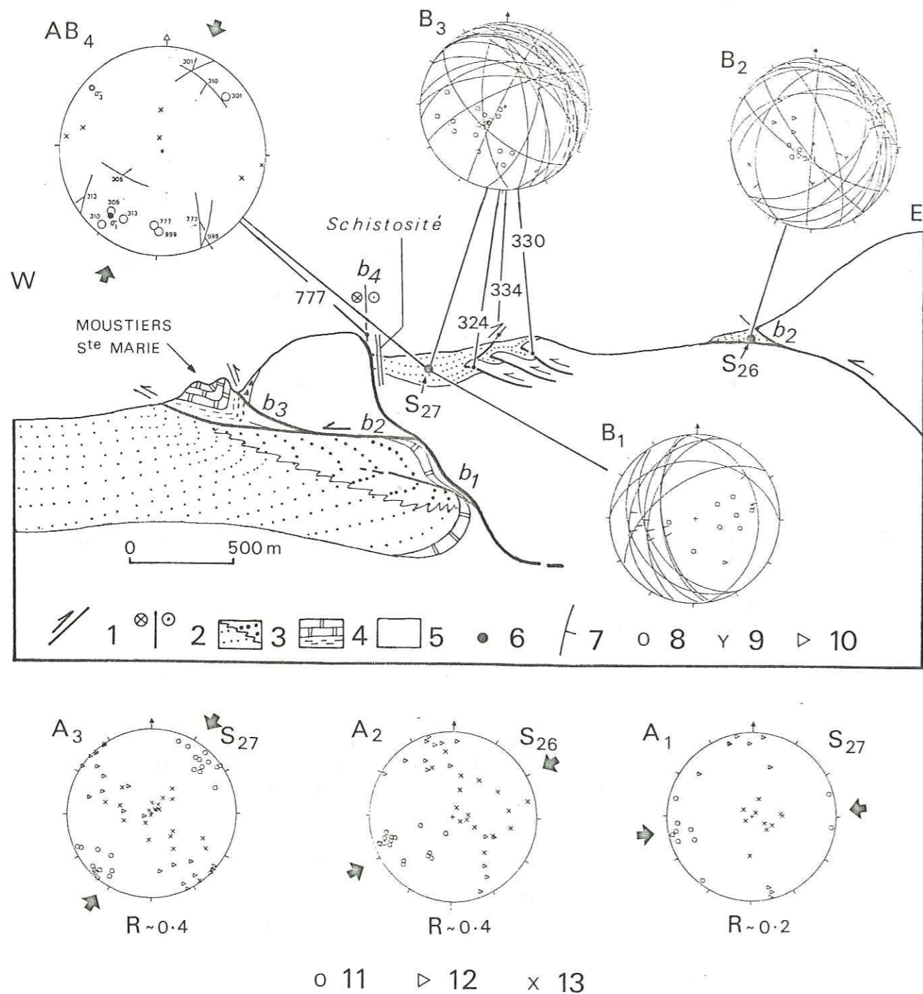
FIGURE 26 : Les rapports contraintes-déformations au cours du changement d'épisode tectonique MIO-PLIOCENE/PLEISTOCENE : exemple du front subalpin dans la région de Moustiers Ste Marie. 1-Faille chevauchante. 2-Décrochement. 3-Conglomérat du Valensole d'âge mio-pliocène. 4-Calcaires et marnes miocène. 5-Calcaires mésozoïque. 6-Station microtectonique. B-Représentation stéréographique des microstructures. 7-Plan de microfaille et sa strie. 8-Pôle de plan Inverse. 9-Séneestre. 10-Dextre. A-Représentation stéréographique des tenseurs de contraintes relatifs à chaque strie. 11-Contrainte maximale \sigma_1 . 12-Contrainte intermédiaire \sigma_2 . 13-Contrainte minimale \sigma_3 .
