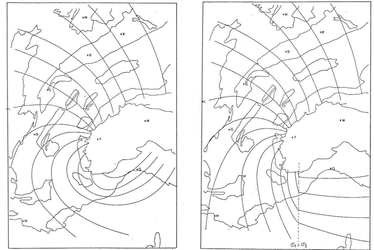
FIG.23c: Interprétation 1; lignes de direction de compression maximale. Interprétation 2
