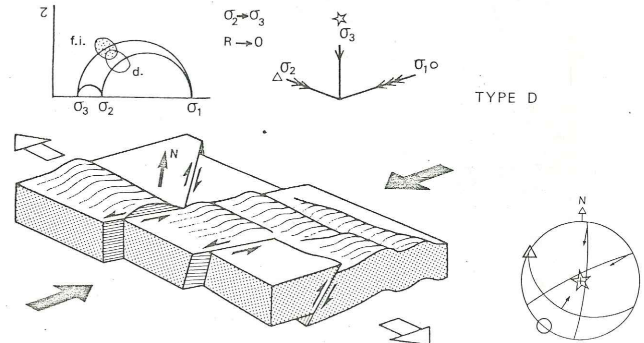
Déformation décrochante compressive
