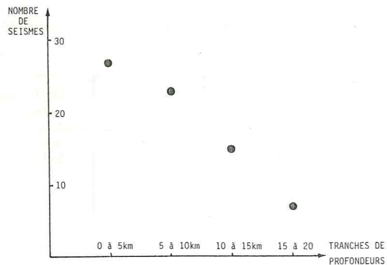
FIG. 41 : Nombre de séismes dont on connaît la profondeur, par tranches de profondeurs (séismes de 1971 à 1978, profondeurs données par l'I.S.C., le B.C.I.S. ou le S.E.D.).
