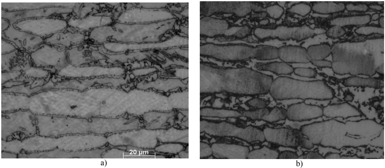
Figure III.31. Micrographies optiques du métal de base vieilli à 850 °C pendant a) 15', b) 5h Suite à une hypotrempe à 1150 °C
