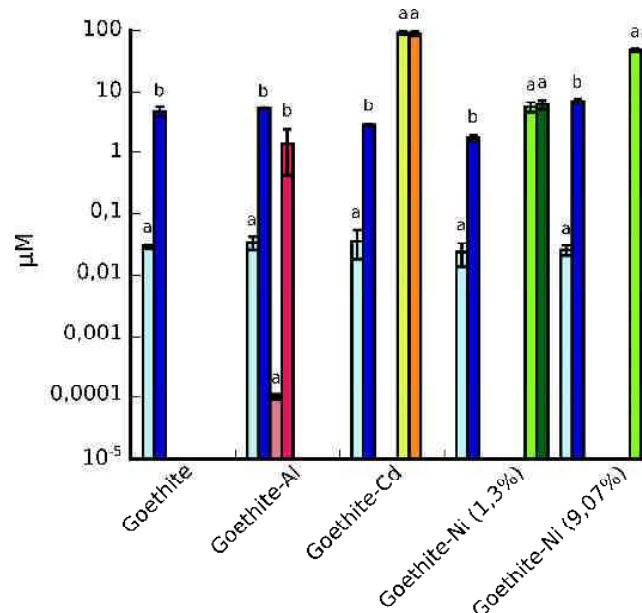
Figure 49 : Solubilisation des métaux présents dans les goethites par la pyoverdine. Les différentes goethites 1 \text{ g.L}^{-1} sont incubées en absence ou en présence de pyoverdine à 50 \text{ } \mu\text{M} en milieu \text{MES-Ca}(\text{NO}_3)_2 . Après 24 h d'incubation, les échantillons sont centrifugés et les teneurs en métaux présents dans la solution sont mesurées par ICP-AES. Sont représentés en bleu, les teneurs en fer, en rose, celles en aluminium, en jaune-orange, les quantités de cadmium et en vert, celles de nickel. Les histogrammes clairs correspondent aux échantillons sans ajout de pyoverdine tandis que les couleurs foncées, aux teneurs mesurées en présence de pyoverdine. Les valeurs représentent les moyennes \pm les déviations standards des 5 répétitions et les lettres indiquent les différences significatives (ANOVA, P < 0,001 ; test de Tukey P < 0,05 ).
