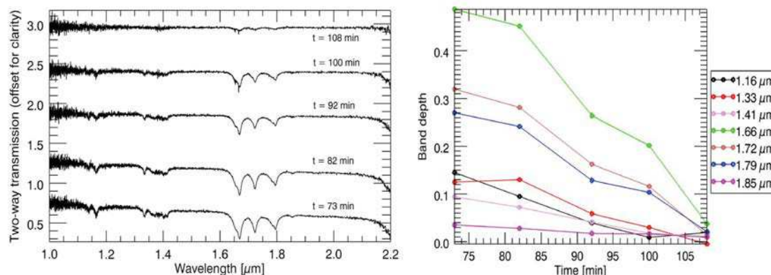
FIGURE 11.17 – Exemple d’une séquence temporelle spectrale d’évaporation de méthane liquide et calcul de profondeurs de bandes associés. Les températures lors de cette expérience test ont été augmentées de 100 à 140 K pour accélérer l’évaporation du méthane. Images : Wasiak et al. (2012a) , modifiées.
