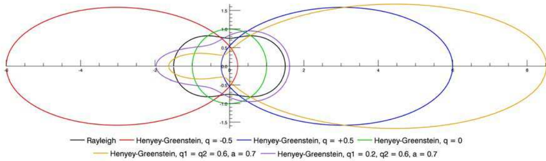
FIGURE 5.8 – Diffusion produite par une particule ayant une fonction de phase P(g) de type Rayleigh (courbe noire) et de type Henye-Greenstein à 1 paramètre (courbes bleue, rouge et verte), à 2 paramètres (courbe jaune) et à 3 paramètres (courbe violette).
