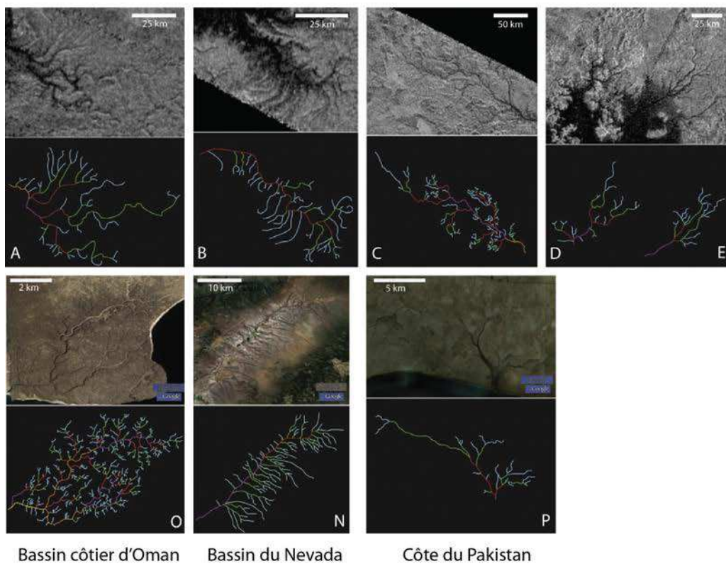
FIGURE 3.16 – Réseaux fluviaux et analogues terrestres (climat aride). Images issues de : Lorenz et al. (2008a) ; Cartwright et al. (2011) ; Langhans et al. (2012) .
