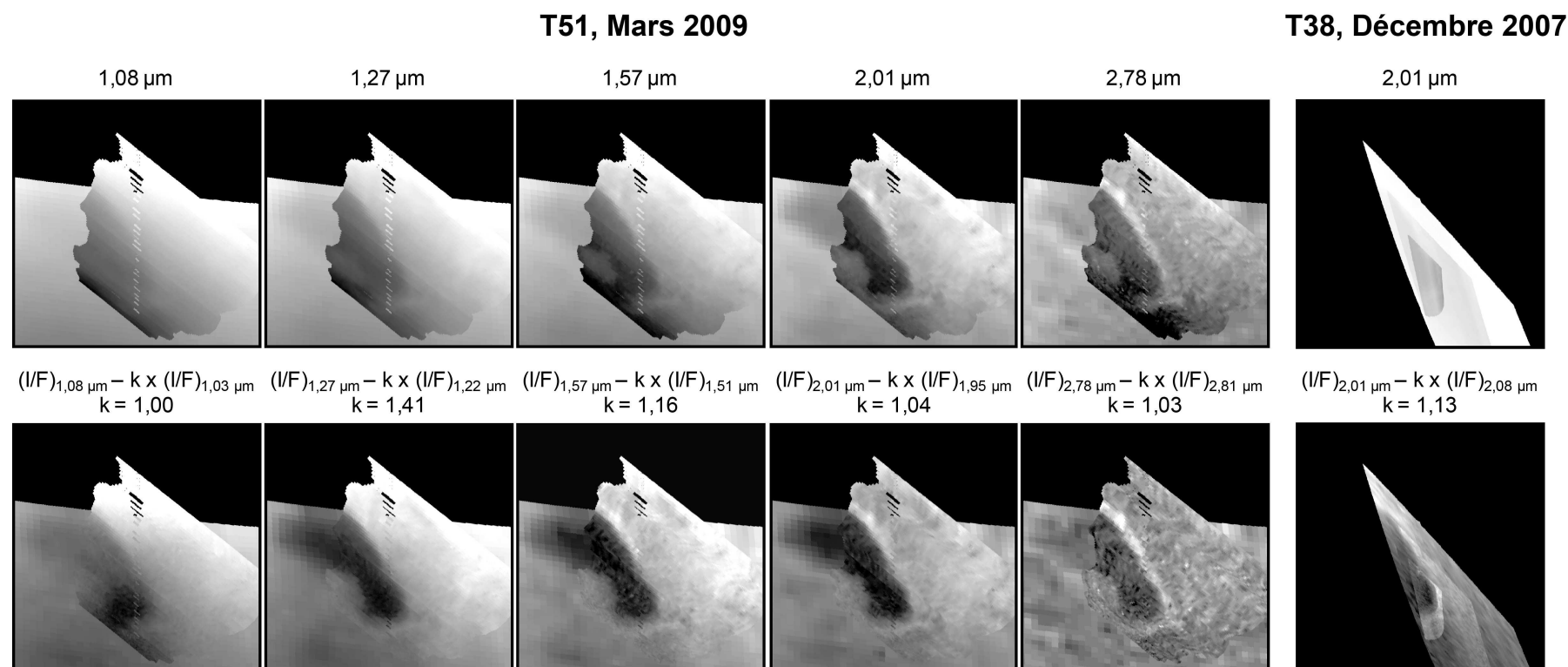
FIGURE 5.21 – Mosaïques VIMS acquises au-dessus d'Ontario Lacus ( 72^\circ\text{S} , 180^\circ\text{E} ) lors des survols T38 (Décembre 2007) et T51 (Mars 2009) brutes puis corrigées de la diffusion atmosphérique.
