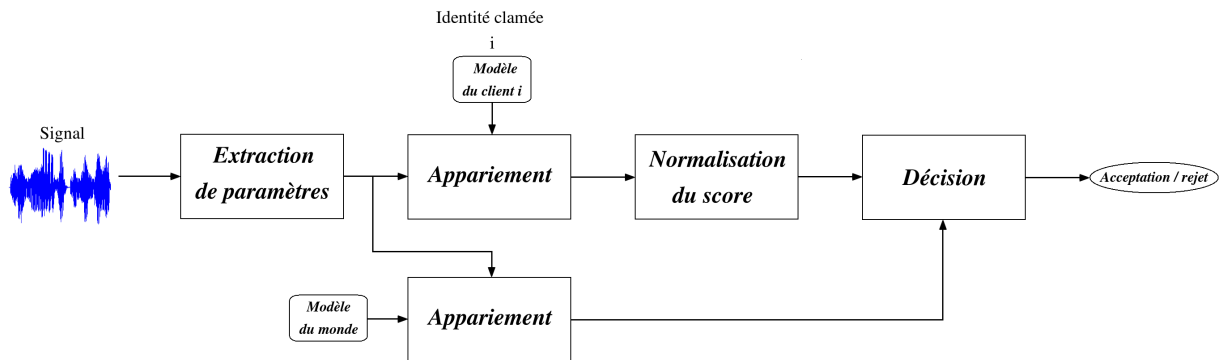
FIG. 2.2: Architecture d'un système de vérification du locuteur.
