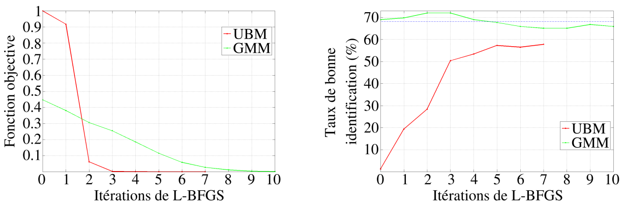
FIG. 4.3: Variation de la fonction objective et du taux de bonne identification, des modèles LM-GMM à 32 gaussiennes : Apprentissage GMM vs Apprentissage UBM.
