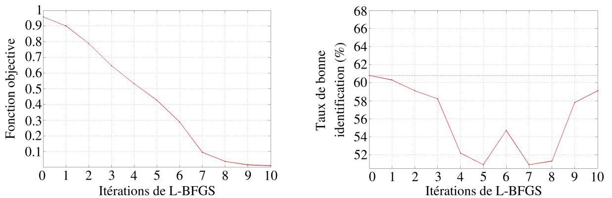
FIG. 3.5: Variation de la fonction objective et du taux de bonne identification, des modèles LM-GMM à 16 gaussiennes.
