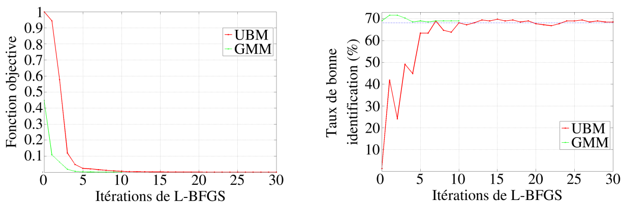
FIG. 4.4: Variation de la fonction objective et du taux de bonne identification, des modèles LM-dGMM à 32 gaussiennes : Apprentissage GMM vs Apprentissage UBM.
