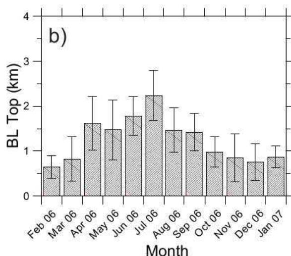
FIGURE 3.9 - Moyennes mensuelles du maximum journalier de hauteur de couche limite mesuré par un lidar Raman automatisé au-dessus de la ville de Leipzig entre février 2006 et janvier 2007. Les barres d'erreur représentent l'écart-type. D'après Baars et al. (2008).
