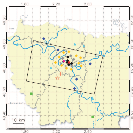
FIGURE 2.4 - Mesure des \text{NO}_x par AIRPARIF : station de fond urbain (losanges), péri-urbaines (triangles cyans) et rurales (carrés verts). Les stations utilisées pour calculer la moyenne intra muros (« couronne ») sont en noir (jaune). La Tour Eiffel est en rose et les stations trafic ne sont pas représentées. La station Qualair et le Sirta sont représentés par une étoile rouge pleine / vide. La croix rouge indique le centre de la maille du modèle ECMWF la plus proche de Paris. Le rectangle noir représente l'empreinte au sol d'un pixel de SCIAMACHY.
