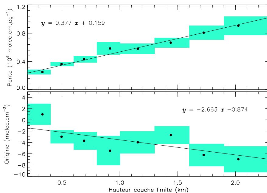
FIGURE 4.13 - Pente (en haut) et ordonnée à l'origine (en bas) de la régression linéaire ( Y|X ) de \Omega_{\text{SZ}} \times 10^{-15} = f(C_{\text{im}}) pour les différentes classes de h_{\text{lid}} . La largeur des boîtes représente la taille des classes et leur hauteur, l'incertitude sur la pente ou l'ordonnée à l'origine.
