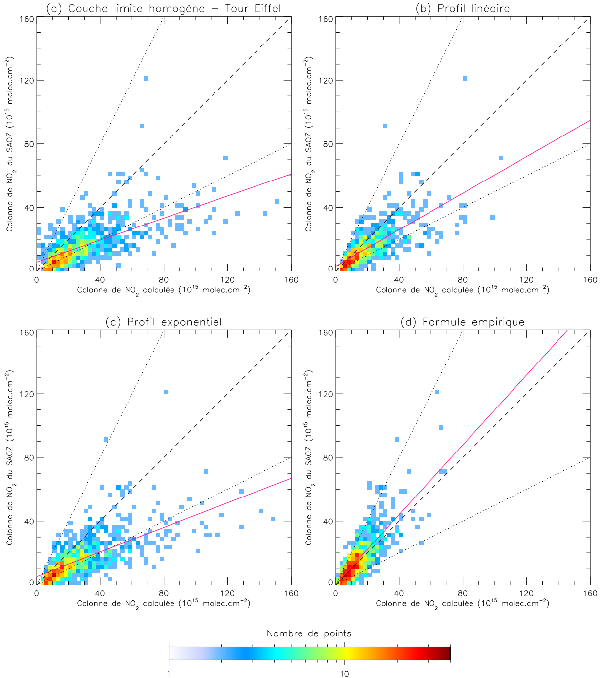
FIGURE 4.14 - Colonnes de \text{NO}_2 observées par le SAOZ en fonction de la colonne calculée selon plusieurs méthodes : intégration d'un profil de concentration (a) homogène au sommet de la Tour Eiffel, (b) linéaire, (c) exponentiel et (d) calcul avec l'équation 4.3. Les points sont répartis dans des classes de taille (2,5 \times 2,5) \cdot 10^{15} \text{ cm}^{-2} et on représente le nombre de points, plus un à cause de l'échelle logarithmique. Les trois droites noires représentent la première bissectrice (tirets) et les droites y = 2x et y = x/2 (pointillés). La droite rose représente la régression linéaire (Y|X).
