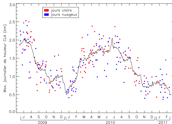
FIGURE 3.5 - Série temporelle du maximum journalier de hauteur de couche limite observé par le lidar de la station Qualair, avec les jours clairs/nuageux en rouge/bleu. La ligne noire représente la moyenne glissante sur 30 jours.
