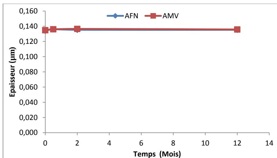
Figure IV–17 : Evolution de l'épaisseur en fonction du temps d'immersion dans une solution de Cr (VI) 0,5 \text{mol L}^{-1} .
