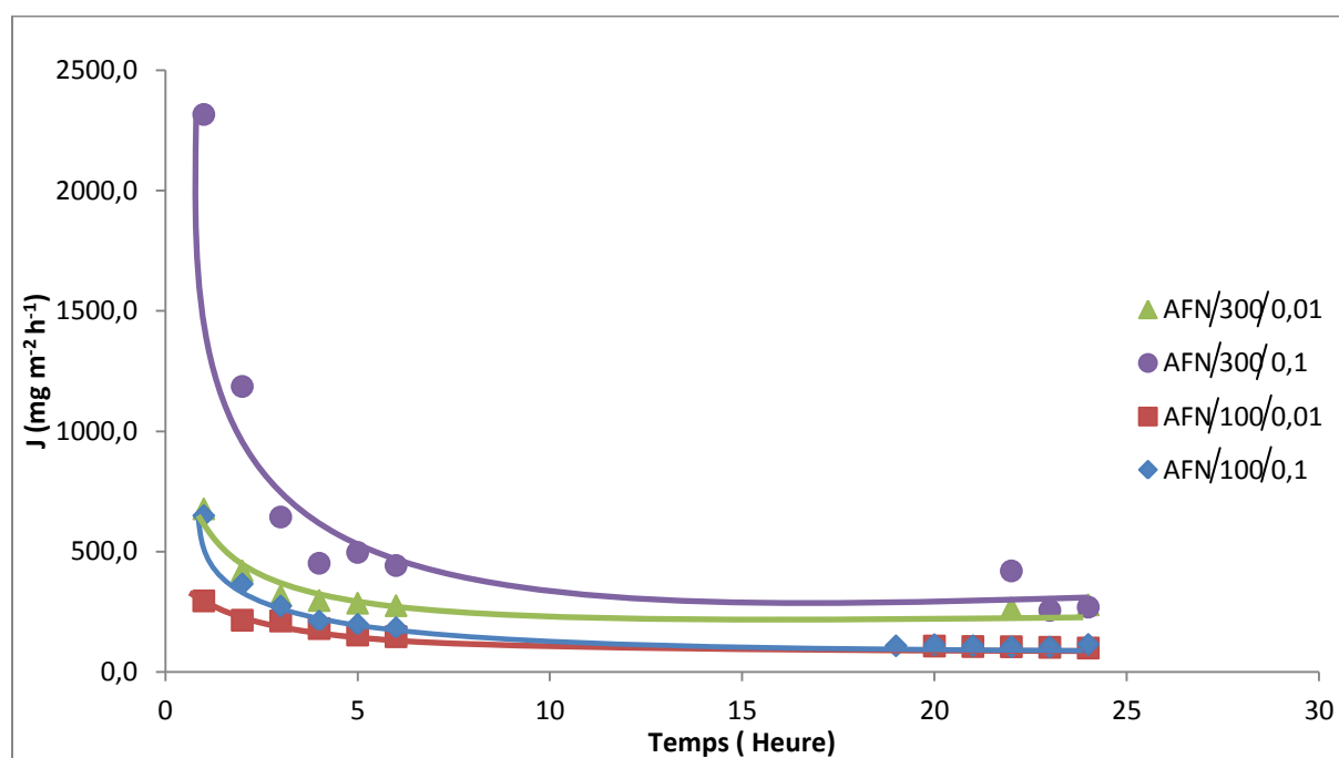
Figure IV- 11 : Evolution du flux moyen dans le compartiment receveur pour la membrane AFN.
