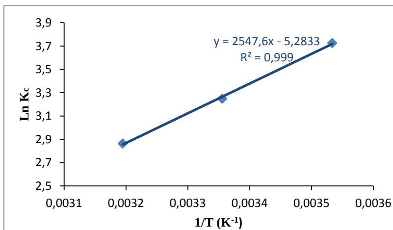
Figure III- 16 : Détermination des paramètres thermodynamiques.
