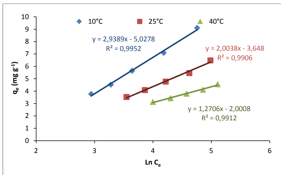
Figure III-12 : Isothermes d'adsorption du chrome sur l'alumine activée selon le modèle de Temkin
