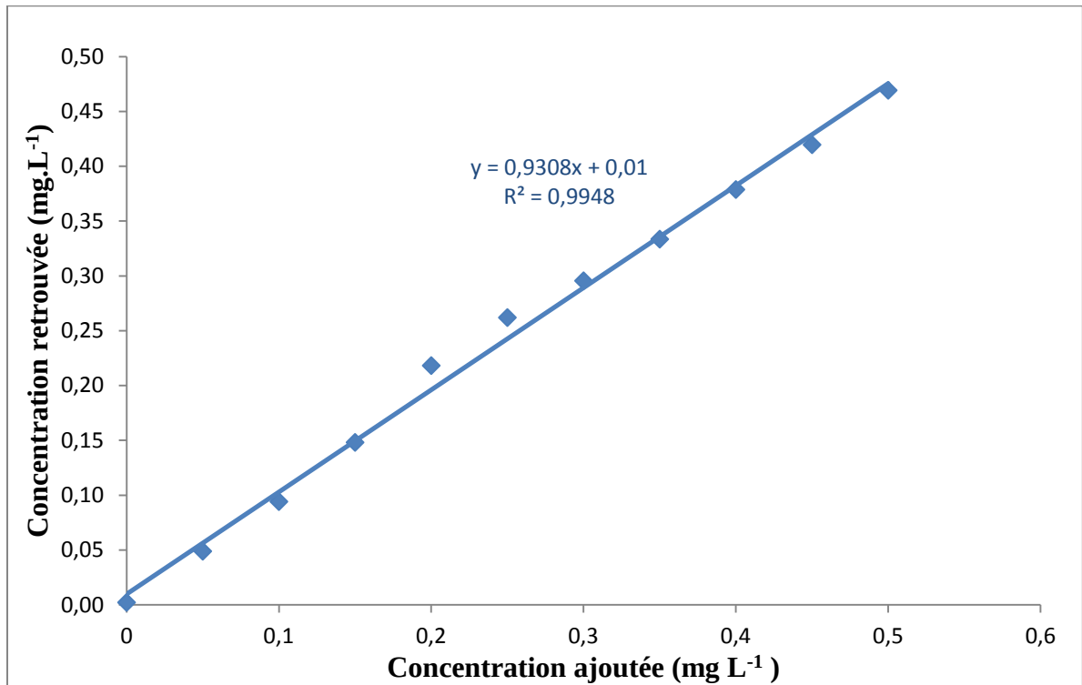
Figure II-3 : Courbe de recouvrement.
