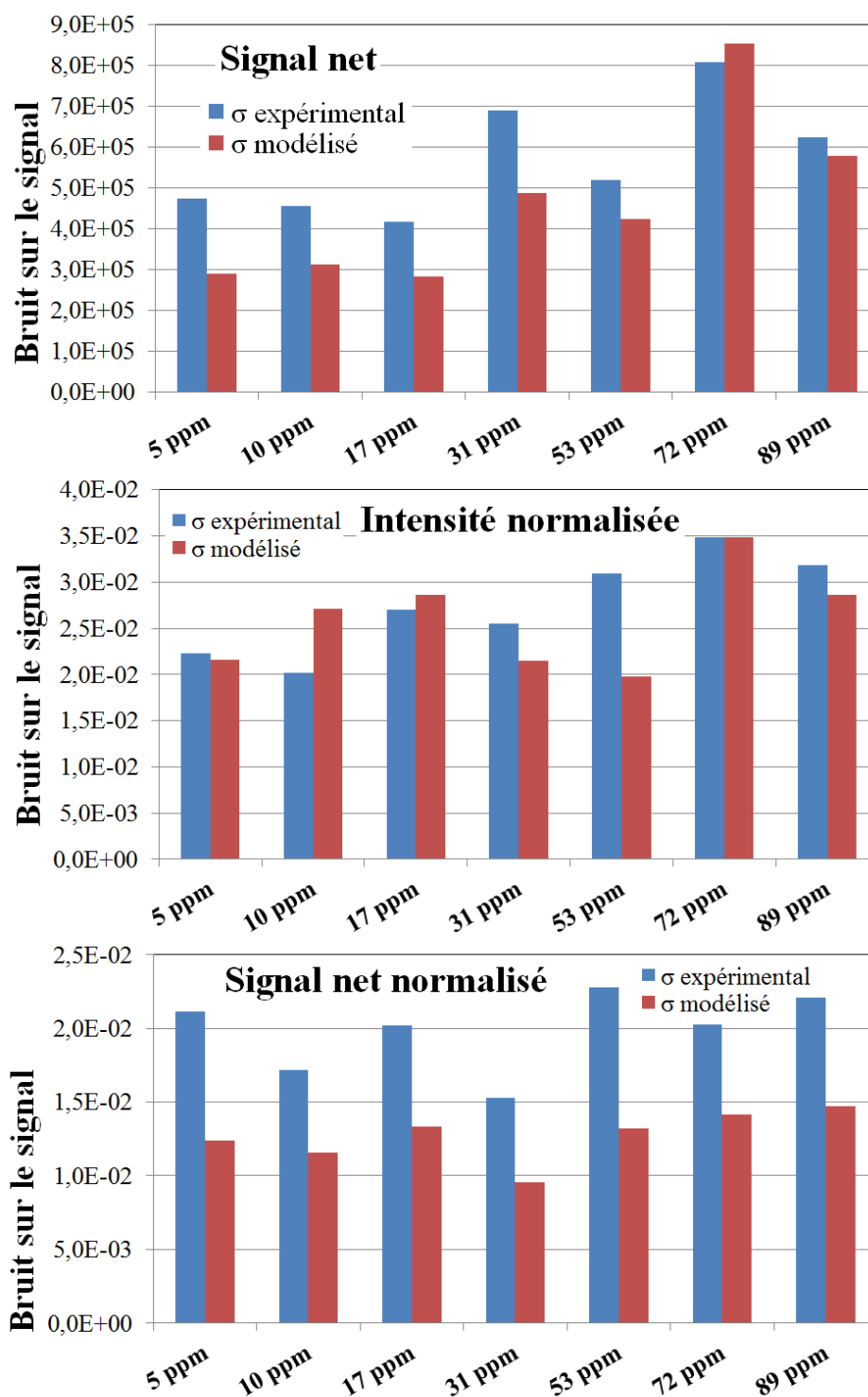
FIGURE 4.13 – Comparaison pour différentes concentrations en plomb entre les bruits totaux sur le signal net, l'intensité brute normalisée et le signal net normalisé, calculés expérimentalement et en appliquant le modèle aux données expérimentales.
