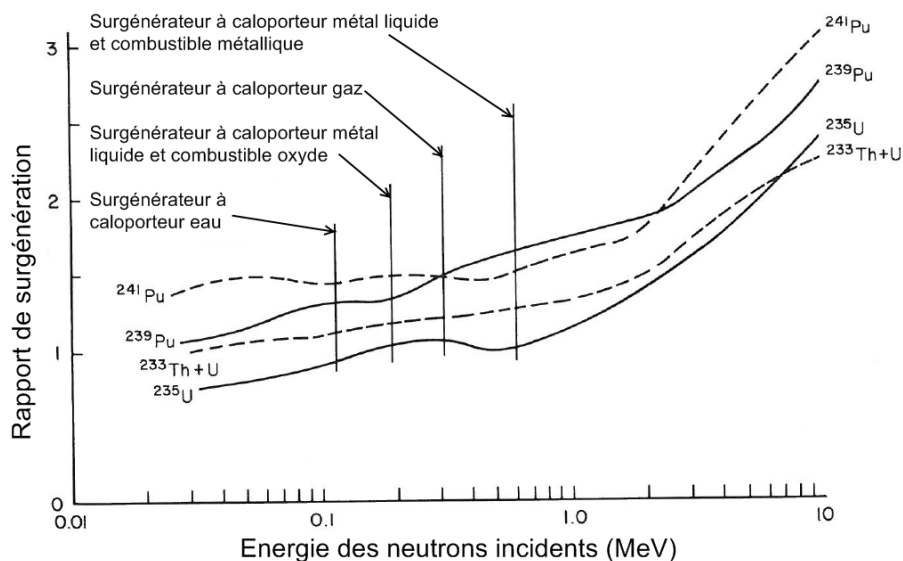
FIGURE 1.2 – Evolution de la capacité du réacteur à produire de la matière fissile à partir de la matière fertile (Rapport de surgénération) en fonction du type de réacteur, du noyau fissile obtenu et de l'énergie cinétique des neutrons incidents [2].
