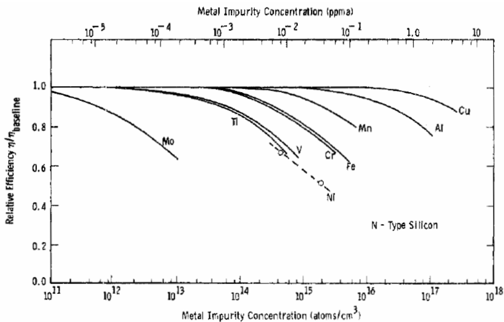
Figure 19 : Evolution du rendement de conversion normalisé en fonction de la concentration en impuretés métalliques pour différentes impuretés [10]. Silicium de type n de 1.5 \Omega .cm.
