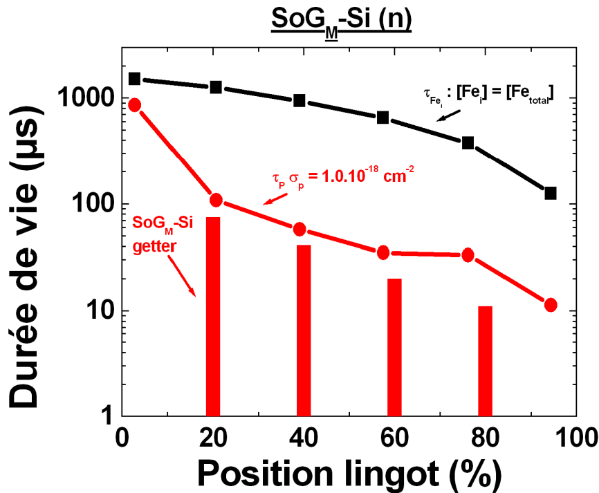
Figure 75 : Evolution de la durée de vie des porteurs de charge mesurée sur le lingot SoG_M-Si (n) (histogrammes), limitée par le fer (carrés), limitée par les recombinaisons SRH liées au phosphore (cercles).
