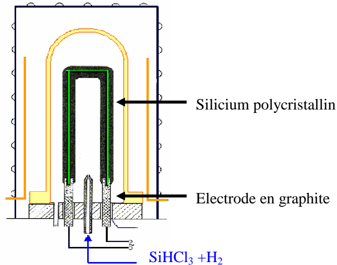
Figure 6 : Réacteur Siemens .
