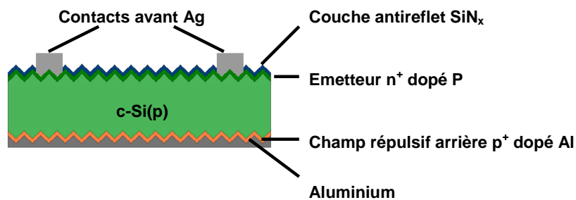
Figure 35 : Schéma de la structure standard.
