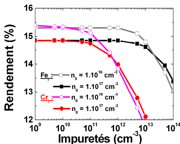
Figure 99 : Evolution du rendement de conversion en fonction de la concentration en Cr i et Fe i .
