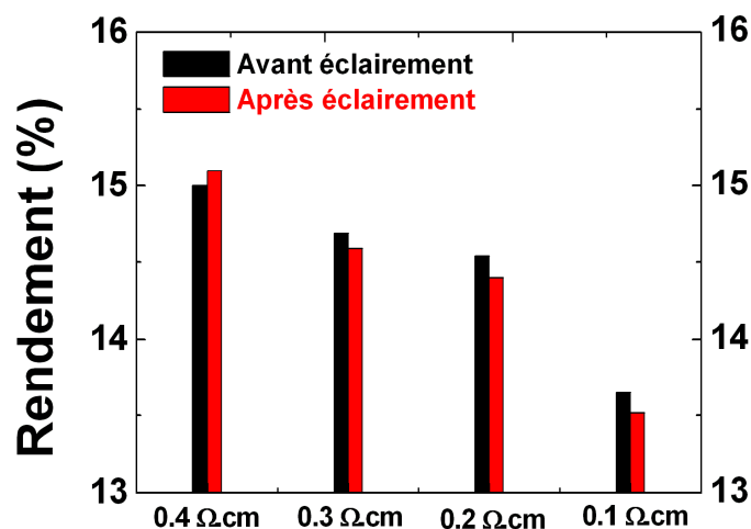
Figure 127 : Evolution du rendement de conversion de cellules PV issues du lingot SoG_M-Si (n) ( \rho = 0.1, 0.2, 0.3 et 0.4 \text{ } \Omega\text{cm} ) avant et après illumination.
