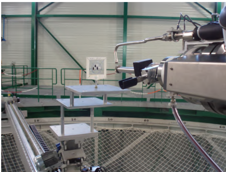
Figure E 5- Irradiations des CR-39 aux basses énergies auprès de l'installation Amande. Le support des détecteurs, la plaque en plexiglas et les CR-39 apparaissent sur la figure.
