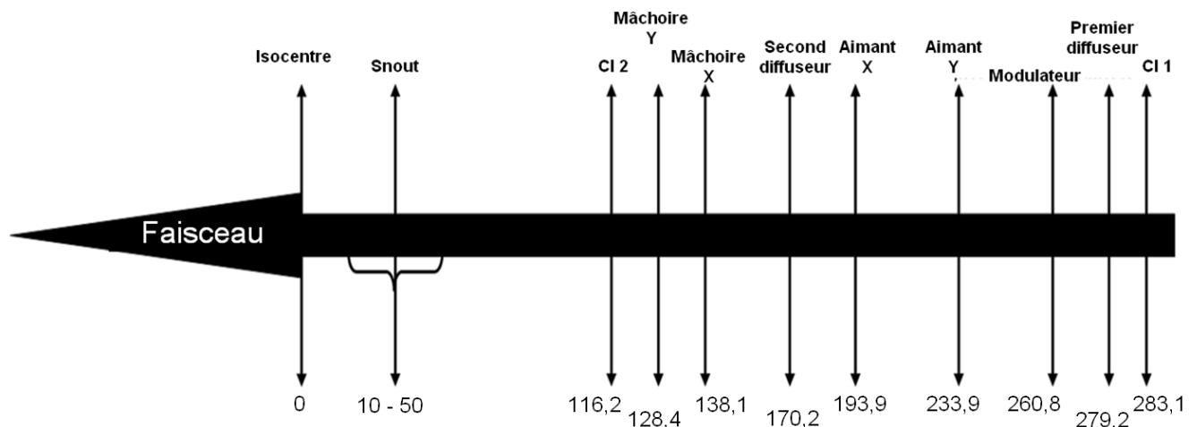
Figure II.2- Dispositifs présents dans la ligne IBA. La flèche indique la direction du faisceau de protons et les distances (en cm) séparant chaque élément de l'isocentre sont donnés en bas (CI : chambre d'ionisation).
