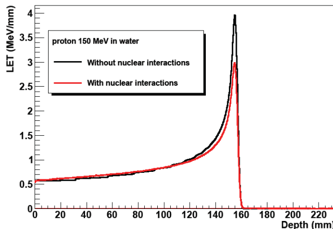
Figure I.10- Variation de l'énergie déposée en profondeur avec (courbe rouge) ou sans (courbe noire) prise en compte des interactions nucléaires (adaptée de Cussol, 2011).
