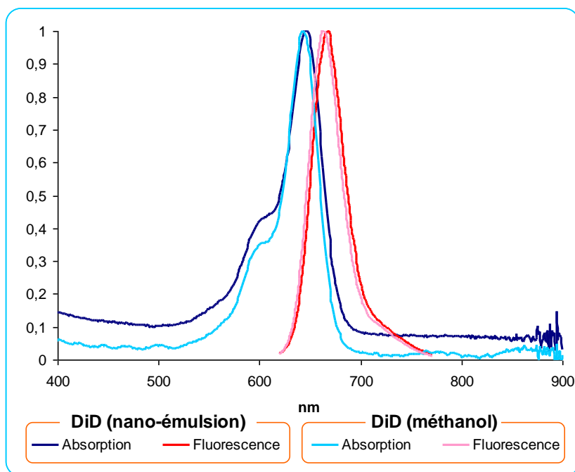
Figure IV-12 : Comparaison des spectres d'absorption et d'émission de nano-émulsions dopées DiD avec ceux du DiD en solution dans le méthanol.
