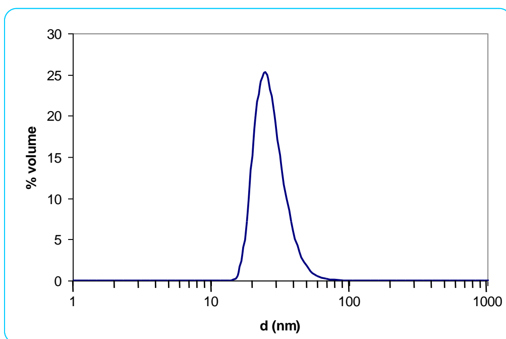
Figure III-6 : Distribution en taille (pondération en volume) d'une solution de nano-émulsions issues de la formulation dite de « référence » à température ambiante après fabrication.
