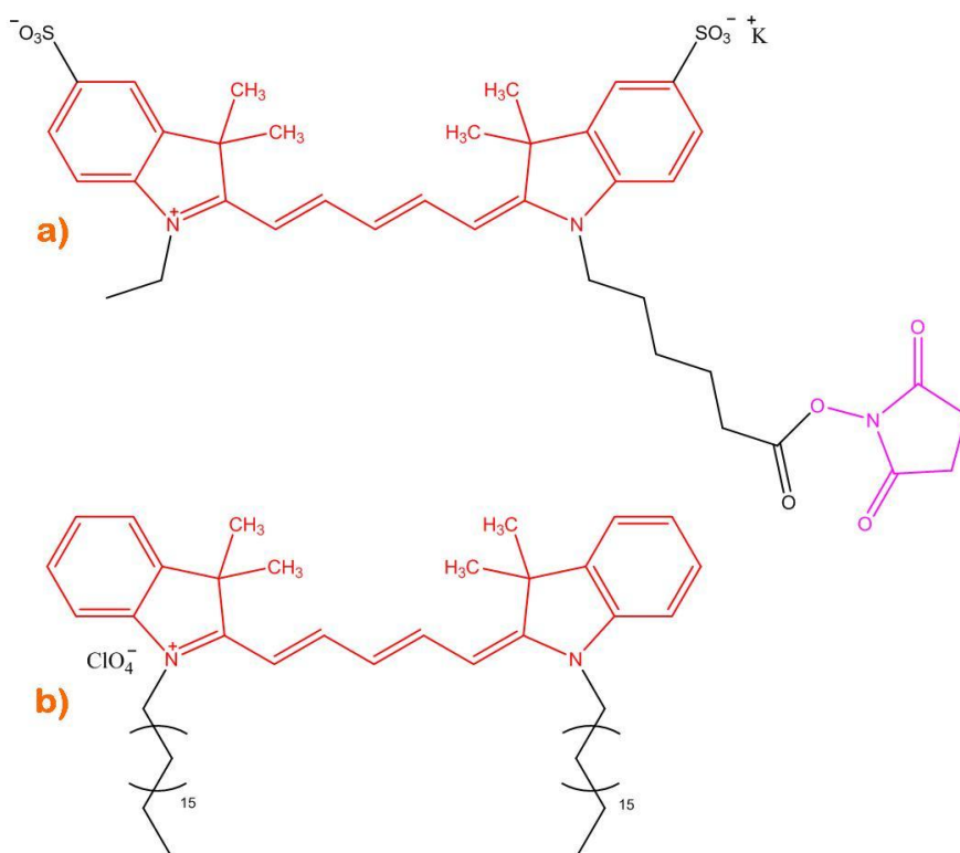
Figure IV-4 : Structure des molécules fluorescentes a) Cyanine 5 (Cy5) ; b) DiD. Les sous-structures représentées en rouge font ressortir l'analogie structurale entre les deux fluorophores en ce qui concerne la partie aromatique responsable des propriétés optiques. La sous-structure du fluorophore hydrophile représentée en violet correspond aux groupes de greffage, ici des esters activés par un groupement N-hydroxysuccinimide capable de former une liaison amide avec des amines.
