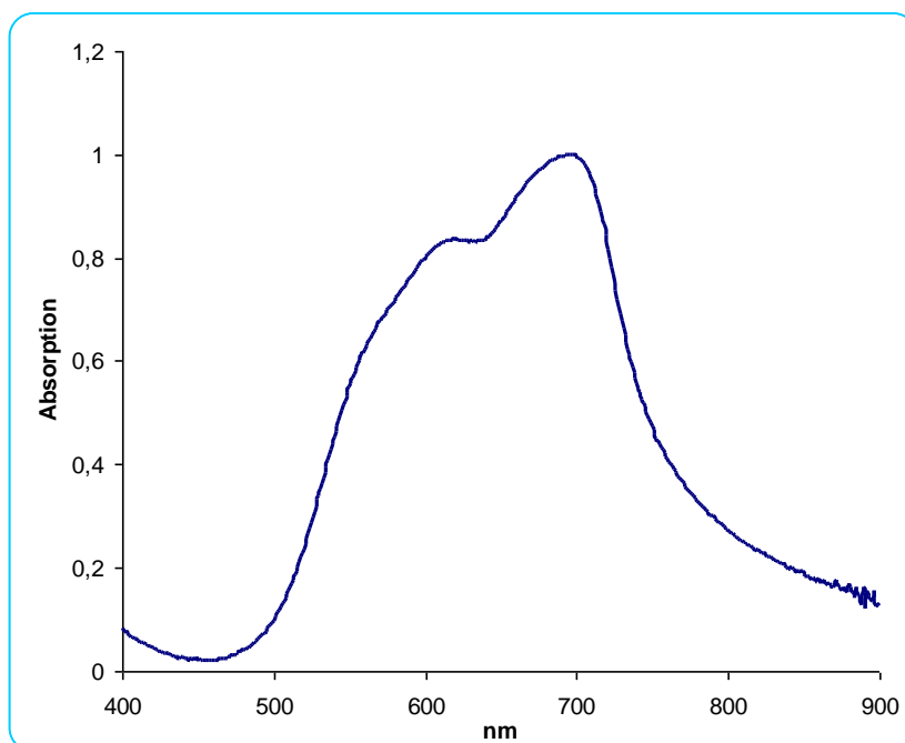
Figure IV-11 : Spectre d'absorption du DiD en solution aqueuse.
