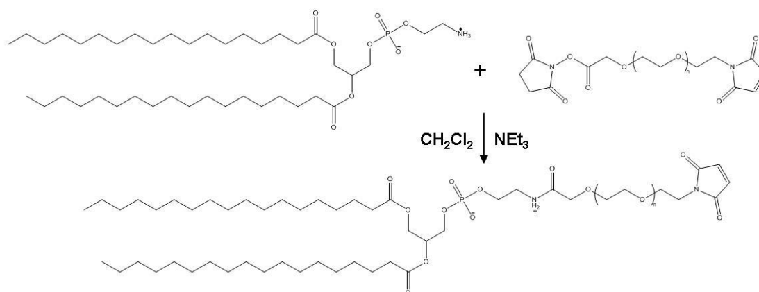
Figure A-1 : Schéma de synthèse du PE-PEG5000-MAL.
