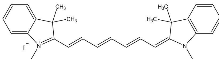
Figure IV-14 : Structure du HITC.
