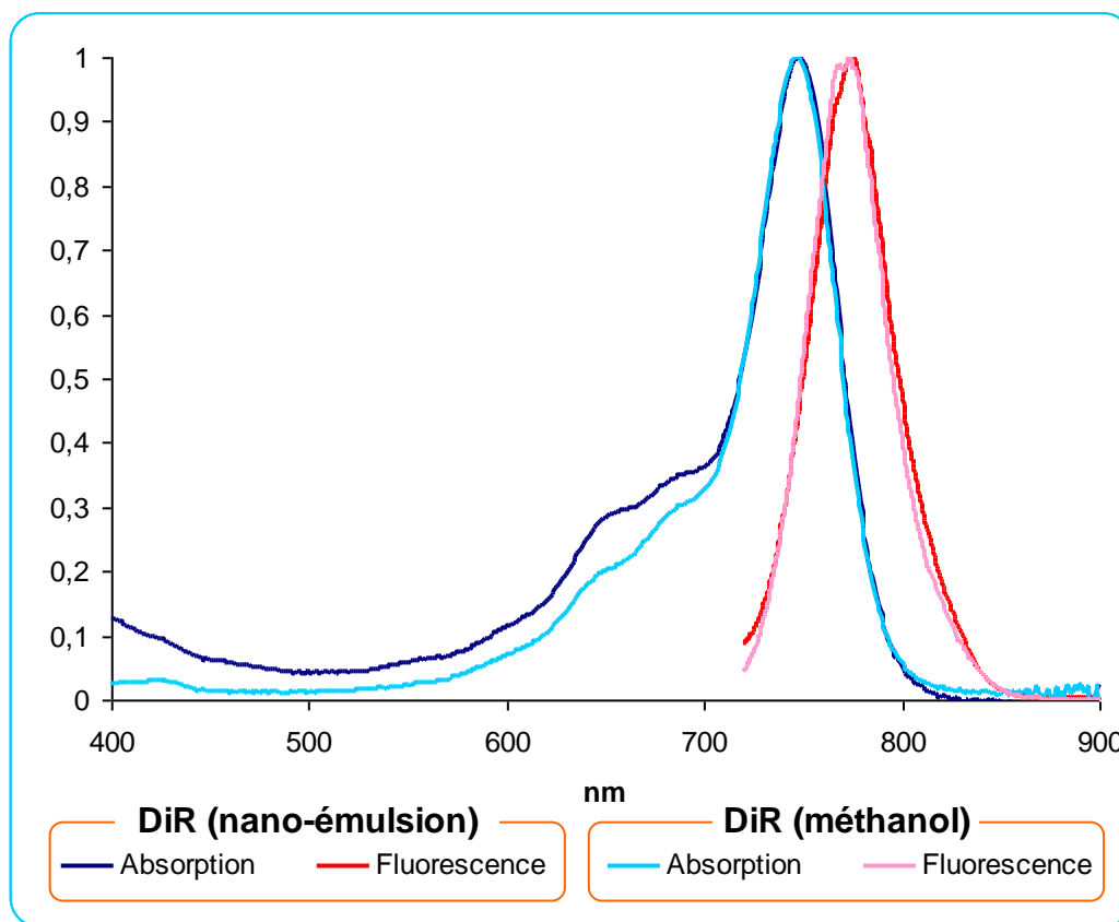
Figure IV-13 : Comparaison des spectres d'absorption et d'émission de nano-émulsions dopées DiR avec ceux du DiR en solution dans le méthanol.
