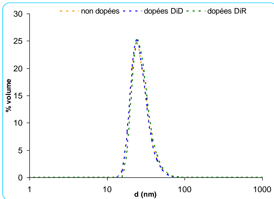
Figure IV-7 : Comparaison de la distribution en taille de nano-émulsions en fonction du dopage
