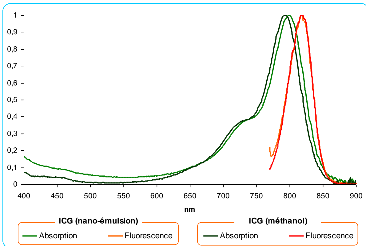
Figure C-1 : Comparaison des spectres d'absorption et d'émission de nano-émulsions dopées ICG avec ceux de l'ICG en solution dans le méthanol.
