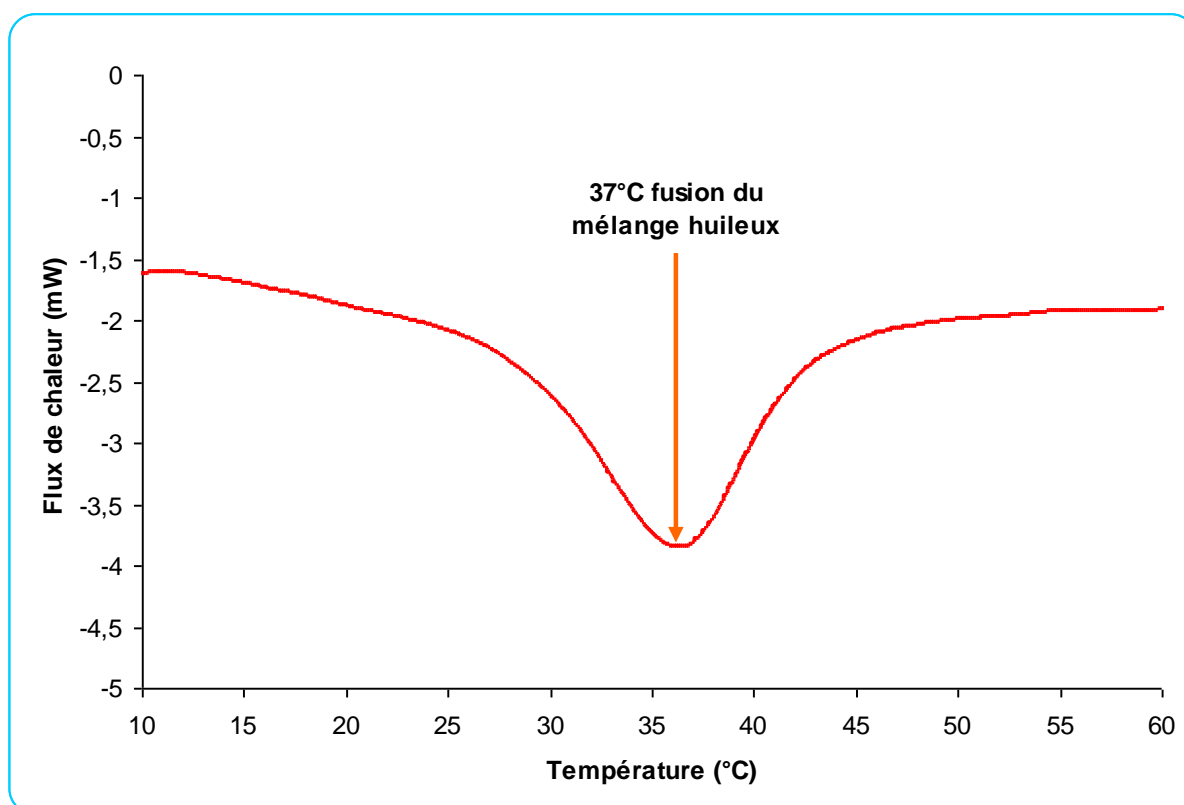
Figure III-9 : Thermogramme du mélange huileux entrant dans la composition des nano-émulsions.
