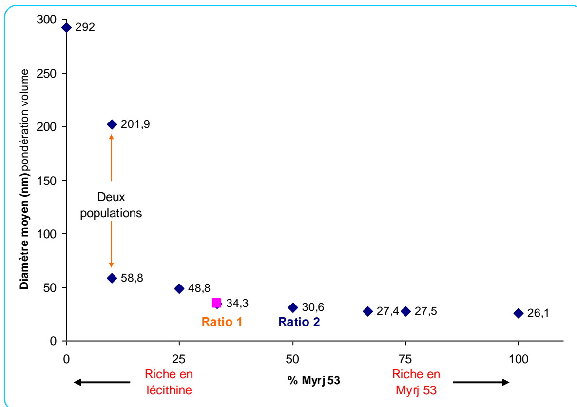
Figure III–16 : Evolution du diamètre moyen des globules en fonction du pourcentage molaire de surfactant pegylé. La formulation de référence est représentée par le carré rose. Les ratios molaires 1 et 2 correspondent respectivement à 66,7 % lécithine / 33,3 % Myrj 53 et 50 % lécithine / 50 % Myrj 53.
