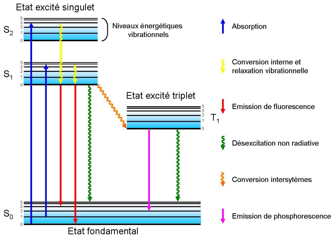
Figure II-3 : Diagramme de Jabłoński.
