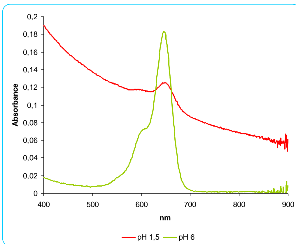
Figure IV-21 : Comparaison des spectres d'absorption de solutions dont le pH est acide et neutre.
