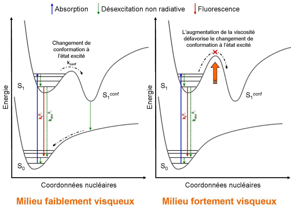
Figure IV-24 : Schéma simplifié des états électroniques fondamentaux et excités d'une molécule fluorescente pouvant changer de configuration à l'état excité en fonction de la viscosité du milieu.
