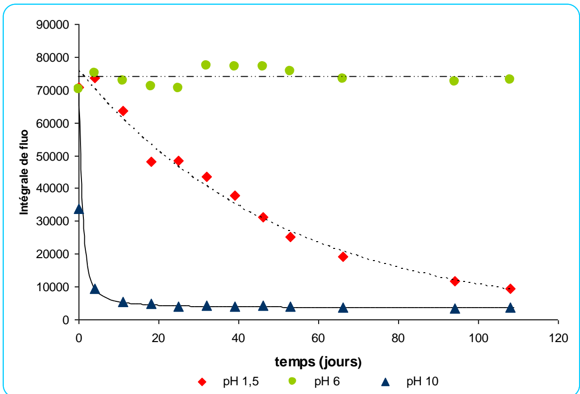
Figure IV-19 : Evolution de la fluorescence en fonction du temps pour trois solutions de pH différents.
