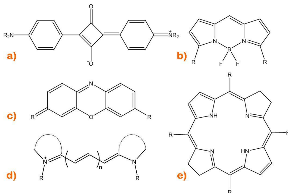
Figure IV-2 : Structures générales de fluorophores pouvant émettre et absorber dans le proche infrarouge : a) squaraines ; b) borondipyrométhènes ; c) oxazines ; d) cyanines ; e) bactériochlorines.
