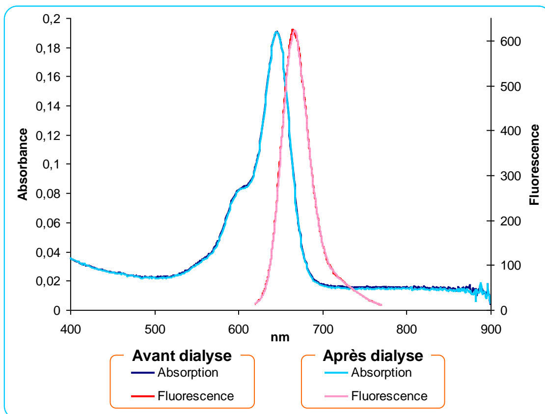
Figure IV-17 : Spectres d'absorption et d'émission d'une nano-émulsion dopée à 400 µM en DiD avant et après dialyse (15 jours à 37°C contre de l'eau déionisée ; seuil de coupure de la membrane : 12-14000 kDa). L'unité de fluorescence est une unité arbitraire.
