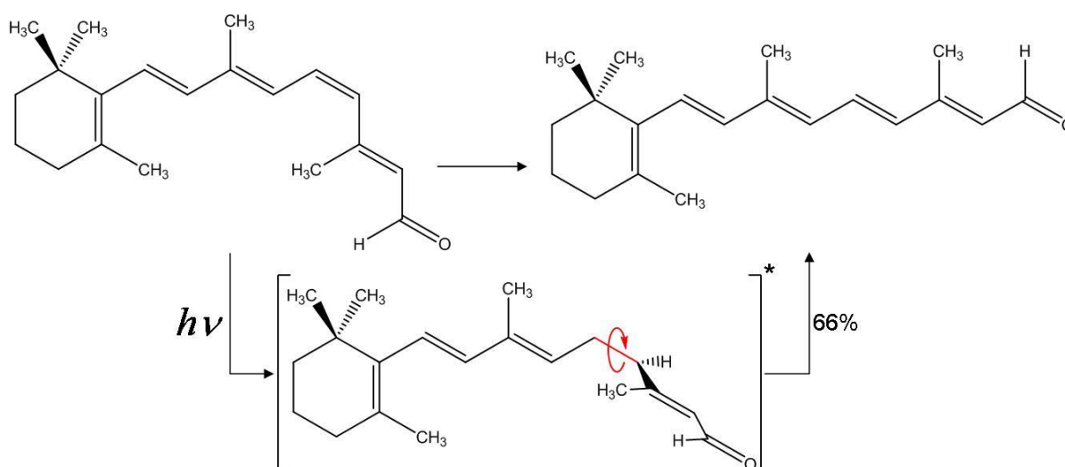
Figure IV-23 : Photo-isomérisation du 11-cis rétinol en tout trans rétinol.
