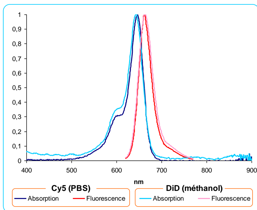
Figure IV-10 : Spectres d'absorption et d'émission de la Cyanine 5 en solution dans une solution tampon PBS (Phosphine Buffer Saline) et du DiD en solution dans le méthanol.
