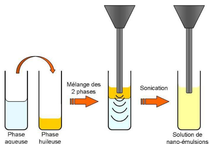
Figure III-4 : Schéma du protocole de préparation d'une solution de nano-émulsions.
