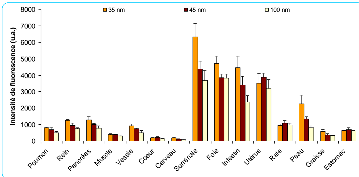
Figure V-16 : Intensité de fluorescence émise par différents organes en fonction de la taille des nanoparticules, 24 h après l'injection dans la queue de l'animal de 200µL de nano-émulsion fluorescente contenant 10 nmol de fluorophores.
