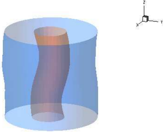
FIG. 2.5 – Iso-surfaces de vorticit  du tourbillon   la fin du r gime faiblement non-lin aire. On remarque que la d formation axiale du c ur du tourbillon est invers e par rapport   sa d formation   la p riph rie.
