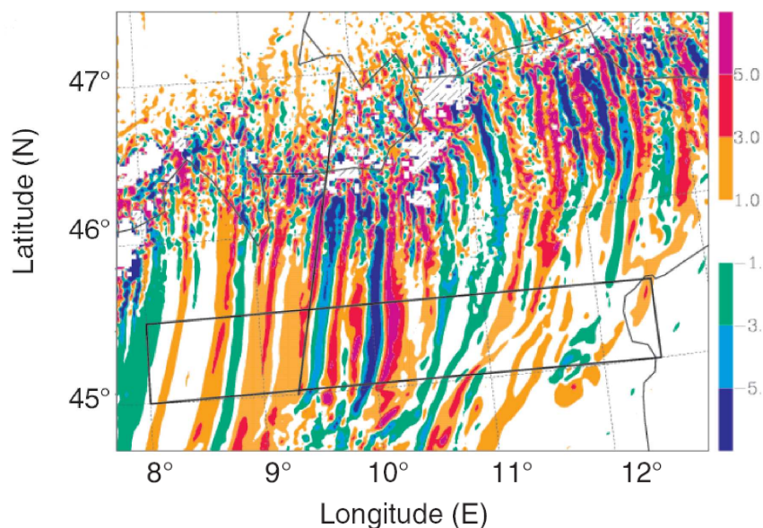
FIG. 1.8 – Champ de vorticit  potentielle   2700 m d'altitude (unit  : 1 PVU= 10^{-6} K.m 2 .kg -1 .s -1 ),   14h00 UTC le 8 Novembre 1999, simul  par MESO-NH (r solution 2km). Les zones hachur es repr sentent la section de l'orographie, et le rectangle noir les trajectoires de l'avion utilis  (Flammant et al 2004).
