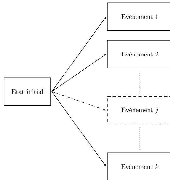
FIG. 3.2 – Représentation schématique d'une situation de risques compétitifs
