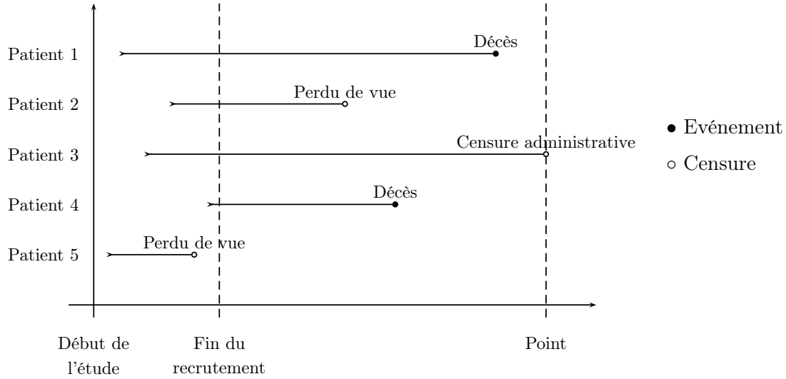
FIG. 3.1 – Représentation schématisée de 5 données de survie
