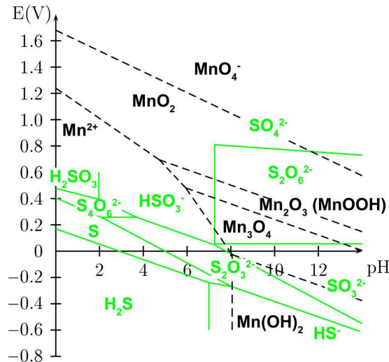
FIG. 6.5 – Diagrammes de Pourbaix simplifiés à 25 °C pour le manganèse et le soufre.[91] E^{\circ}(S_2O_8^{2-} / SO_4^{2-}) = 1,96 V. La courbe n'est pas présentée sur le diagramme E-pH pour plus de clarté.
