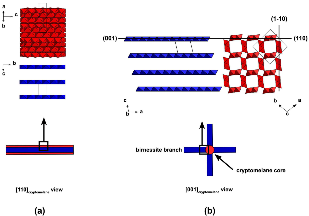
FIG. 4.6 – Schéma représentant les relations épitaxiales lors de la nucléation de la phase birnessite sur une baguette de cryptomélan. Vues dans les directions [110] (a) et [001] (b) du cryptomélan.
