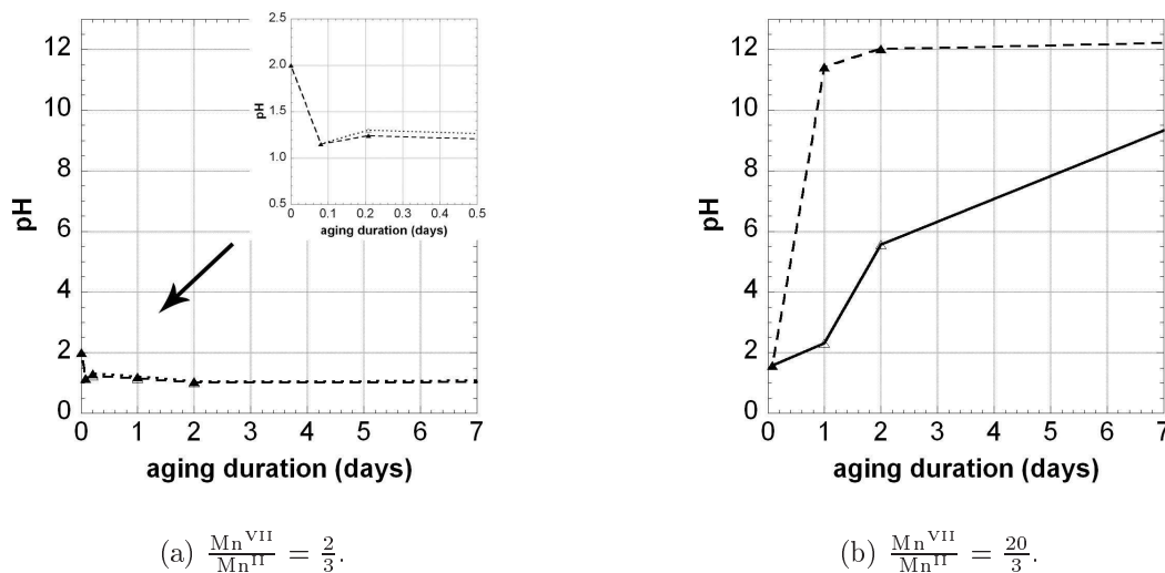
FIG. 2.18 – Evolution du pH du milieu d'évolution à 95 °C, dans le cas de la synthèse par médiamutation pour un pH initial 2,0, évolution à 60 °C (---) ou 95 °C (—): \frac{Mn^{VII}}{Mn^{II}} = \frac{2}{3} (a); \frac{Mn^{VII}}{Mn^{II}} = \frac{20}{3} (b).
