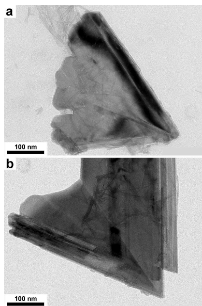
FIG. 4.2 – Clichés TEM de particules de feitknechtite \beta - MnOOH obtenues après réduction du permanganate par le thiosulfate, ( \frac{Mn}{S} = \frac{1}{6} , pH initial 11, après 4 j d'évolution à 60 °C).
