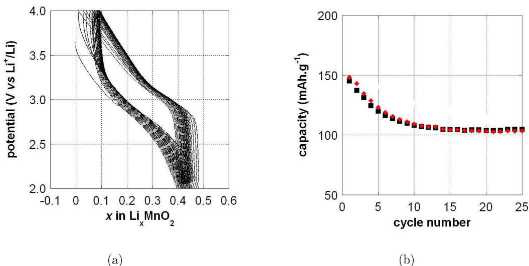
FIG. 7.8 – Courbe potentiel-composition en mode galvanostatique (a) et tenue en cyclage (b) (régime C/10 ) pour la birnessite obtenue par médiamutation, \frac{Mn^{VII}}{Mn^{III}} = \frac{20}{3} , pH initial 2,0, 95^\circ C , 7 jours.
