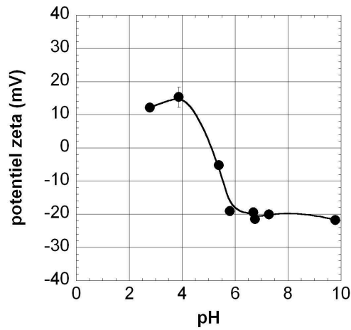
(a) Hausmannite, \text{Mn}_3\text{O}_4 .
