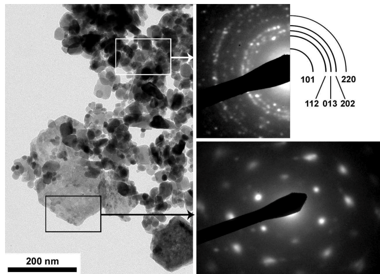
FIG. 2.6 – Clichés TEM et SAED obtenus immédiatement après mélange des réactifs lors de la médiamutation ( \frac{Mn^{VII}}{Mn^{II}} = \frac{2}{30} ) en milieu initial basique (pH 11, pH_f = 12 ). Indexation du diagramme des particules isotropes selon la maille de l'hausmannite.
