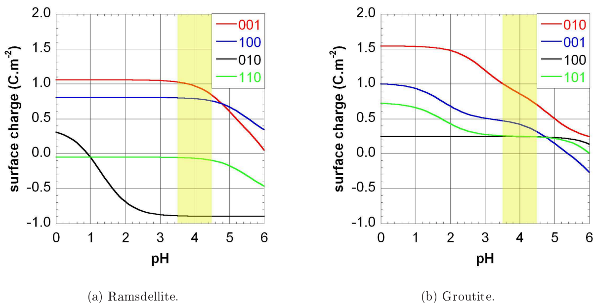
FIG. 5.16 – Charges de surface maximales calculées par les modèles de Brown et Altermatt et MUSIC pour les différentes faces des baguettes de groutite et des cônes, dont la structure est assimilée à celle de la ramsdellite.
