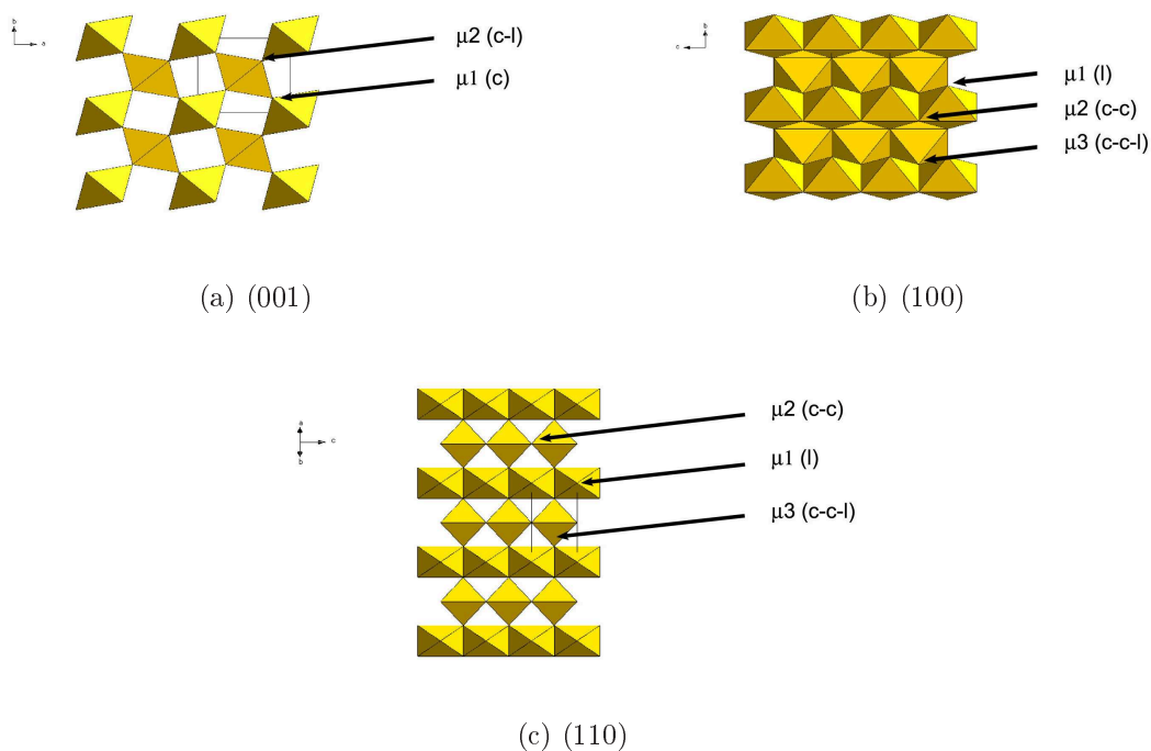
FIG. 1.6 – Faces de la pyrolusite étudiées dans le cadre du modèle MUSIC.
