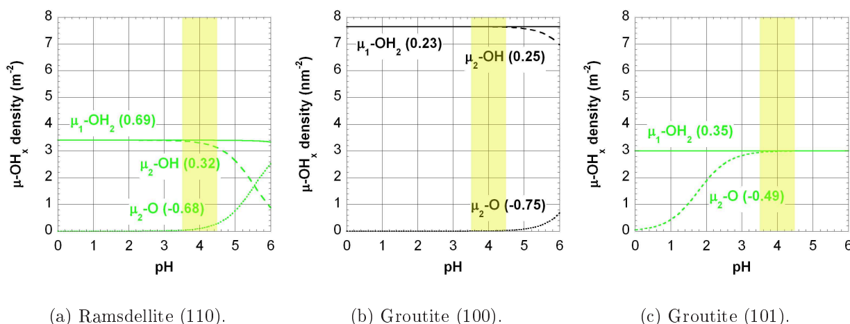
FIG. 5.17 – Répartition des groupes \mu_1 et \mu_2 sur les faces latérales des baguettes de groutite dans les conditions d'acidité correspondant à l'obtention des cônes. Les chiffres entre parenthèses correspondent à la charge portée par le groupe.
