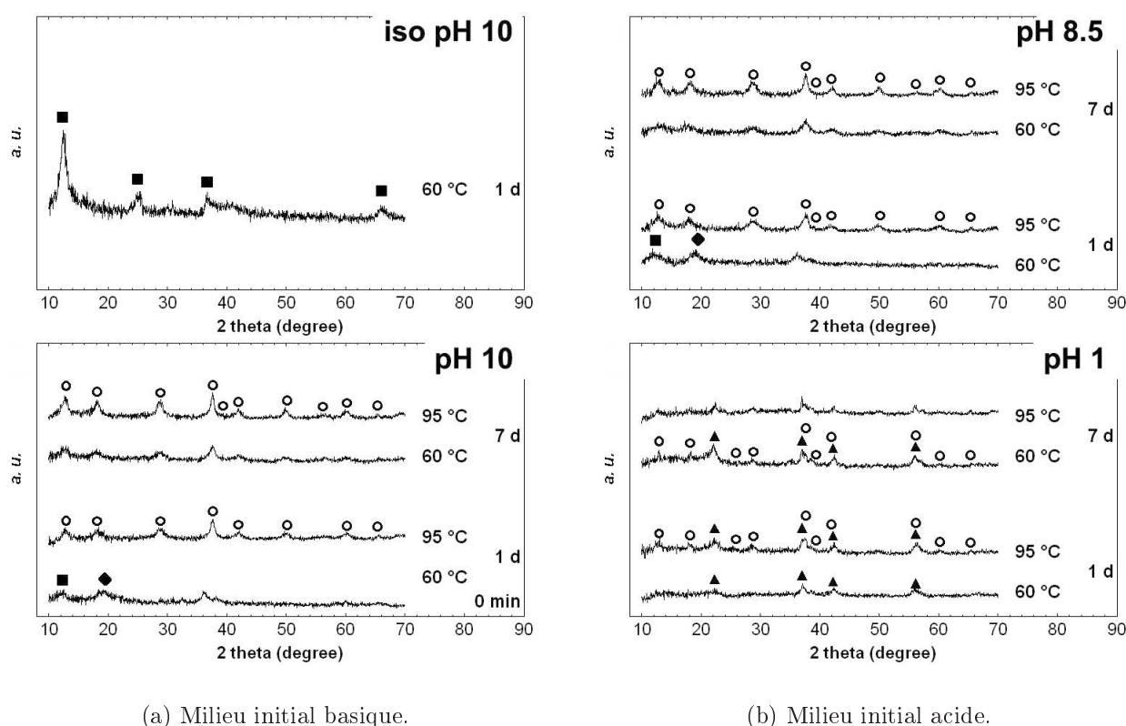
FIG. 5.1 – Diagrammes de DRX décrivant l'évolution structurale lors de la synthèse par oxydation de \text{Mn}^{\text{II}} par du persulfate à différents pH initiaux et températures d'évolution. ◆ : feitknechtite. La signification des autres symboles est donnée sur la fiche insert.
