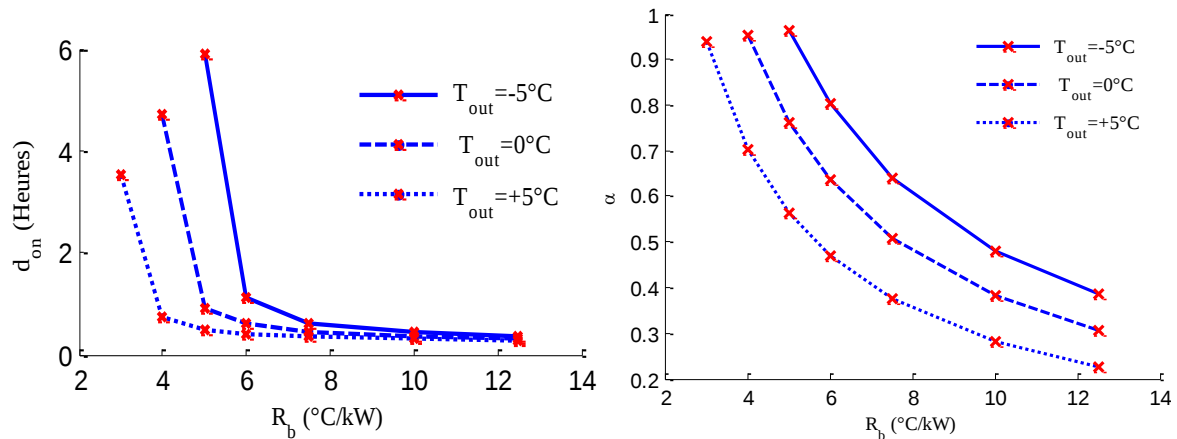
Figure 3-7 La relation entre la durée de chauffe, d_{on} et la résistance thermique équivalente du bâtiment, R_b pour différentes valeurs de T_{out} .
