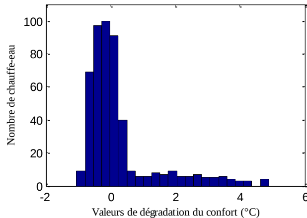
Figure 4-11 Le nombre de chauffe-eau correspondant à chaque valeur de dégradation de confort.
