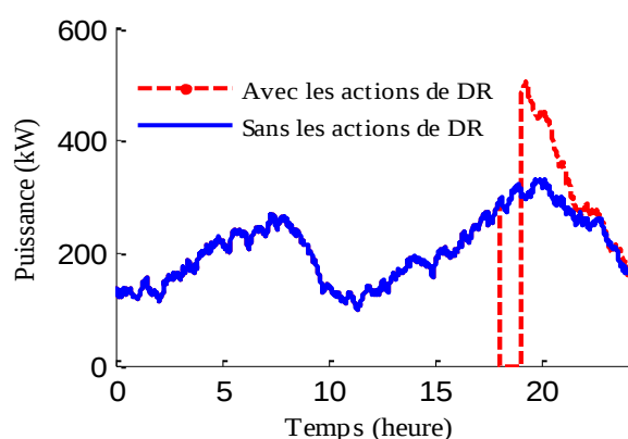
Figure 4-9 Le CLPU généré par la coupure brutale appliquée sur 500 chauffe-eau de 18h à 19h.
