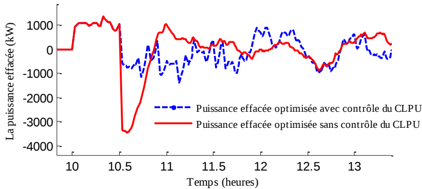
Figure 6-13 Le bloc optimisé d'effacement d'1 MW sans et avec l'optimisation du contrôle du CLPU.
