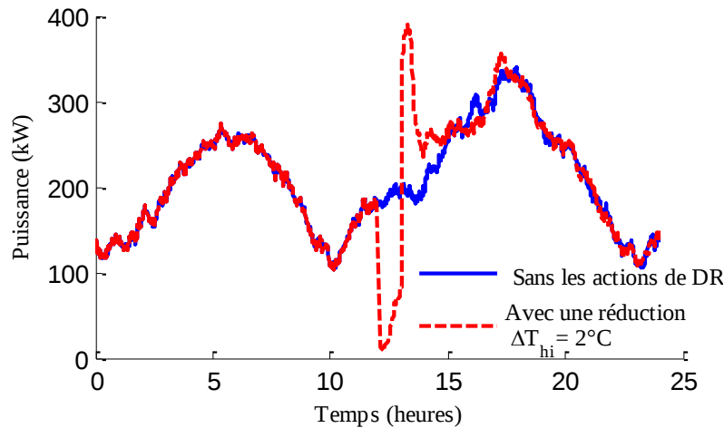
Figure 5-18 La puissance totale consommée par le parc de 500 chauffe-eau sans et avec la réduction de midi à 13h.
