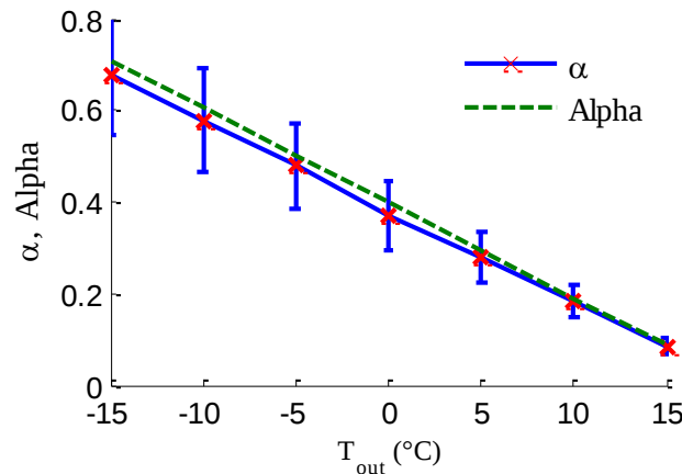
Figure 3-12 La relation entre Alpha, \alpha et la température extérieure du logement, T_{out} , pour une valeur de \Delta T=0.55^{\circ}\text{C} et une valeur moyenne de la température T_{int} égale à 19.22^{\circ}\text{C} .
