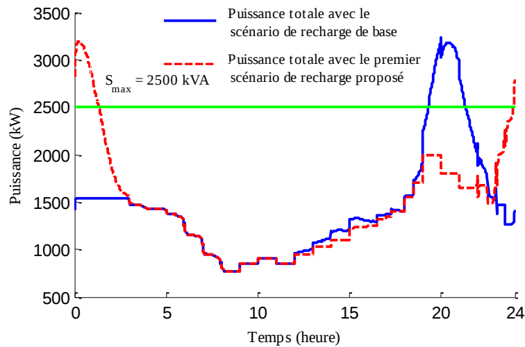
Figure 7-5 les profils de consommation journaliers des 780 logements avec la demande des 500 VEs premièrement en appliquant le scénario de recharge de base et deuxièmement en appliquant le premier scénario de recharge proposé.
