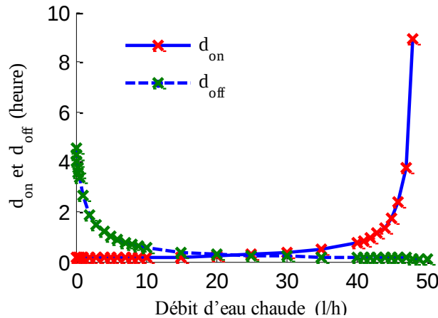
Figure 3-15 Evolution des durées de chauffe ( d_{on} ) et refroidissement ( d_{off} ) en fonction du débit d'eau chaude à T_{ref} , la consommation est maintenu pendant tout le cycle.
