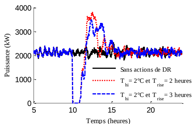
Figure 5-22 La puissance totale consommée par les 500 convecteurs sans et avec la réduction des consignes du thermostat de 10h à 11h pour 2 heures et 3 heures de durée de restitution des consignes et ceci est pour T_{out} = -5^{\circ}\text{C} .
