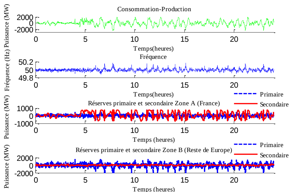
Figure 7-25 Le déséquilibre final entre la production et la consommation, l'évolution temporelle de la fréquence et les réserves primaires et secondaires libérées pour l'ajustement et pour un \Delta P = 1400 MW.
