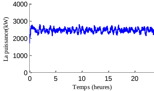
Figure 3-11 La consommation électrique d'un parc de 500 chauffages pour T_{out} = -5^{\circ}C
