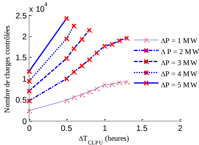
Figure 6-12 La relation entre \Delta T_{CLPU} et le nombre de charges contrôlées et pour différentes valeurs de \Delta P .
