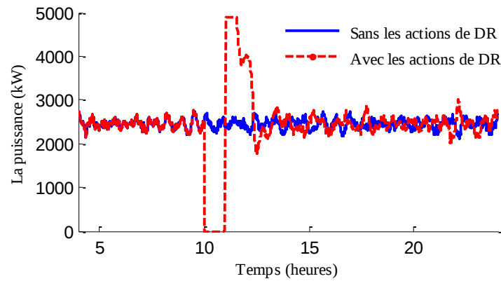
Figure 5-13 Le CLPU obtenu suite à la réduction des consignes des thermostats des 500 convecteurs électriques de 2^{\circ}\text{C} et de 10h à 11h pour T_{out} = -5^{\circ}\text{C} .
