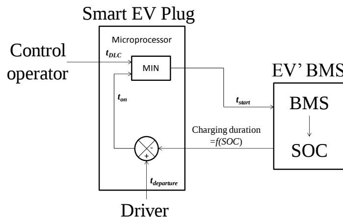
Figure 7-11 L'infrastructure requise pour l'application des actions de DR sur le parc des VE.
