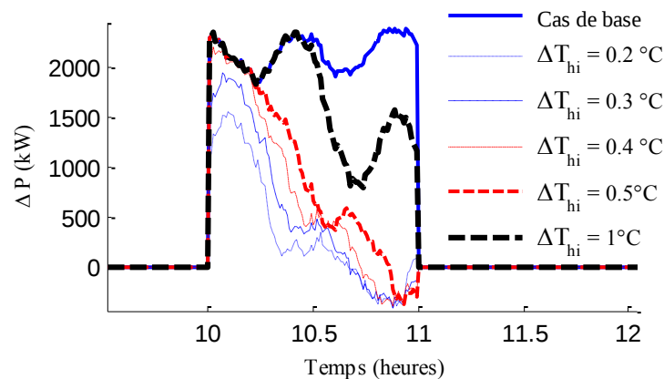
Figure 5-15 Les profils de \Delta P en cas d'application de différentes valeurs de \Delta T_{hi} entre 10h et 11h et pour un \Delta T=0.55^\circ\text{C} , un N=500 et une température T_{out} = -5^\circ\text{C} comparée avec l'application du cas de base et en cachant l'effet du CLPU.
