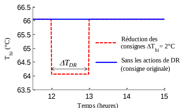
Figure 5-17 La réduction de la consigne T_{hi} de 2^{\circ}\text{C} pendant \Delta T_{DR} .
