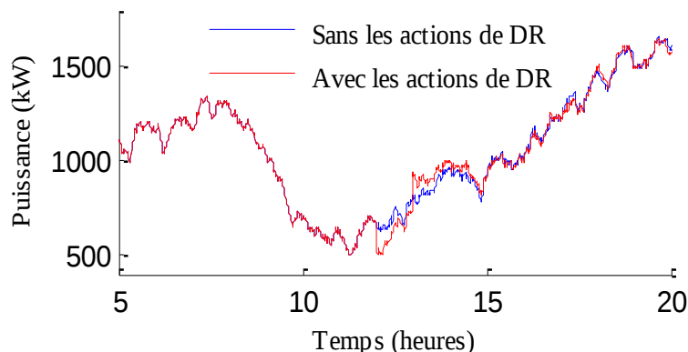
Figure 5-6 La puissance contrôlée et non contrôlée en cas d'application du cas dispatché sur les chauffe-eau et pour la valeur initiale de N_1 , N_2 , N_3 , N_4 et N_5 .
