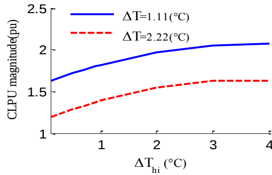
Figure 5-20 Les magnitudes du CLPU pour différentes valeurs de \Delta T_{hi} , et pour deux valeurs de la bande morte des thermostats.
