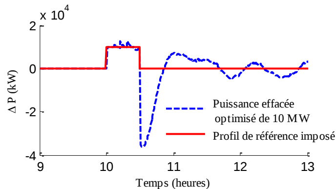
Figure 6-7 Puissance de référence imposée dans l'optimisation et puissance effacée optimisée de 10 MW.
