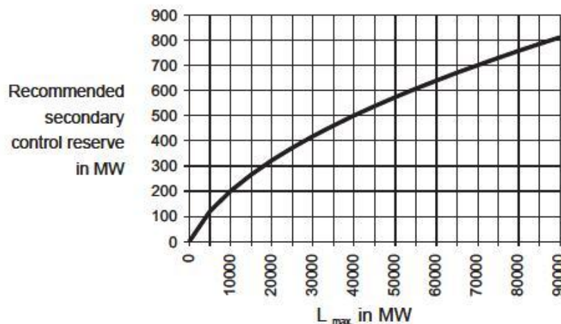
Figure 2-5 La valeur de la réserve secondaire recommandée par l'UCTE en fonction de la demande des charges. [UCTE, 2004]
