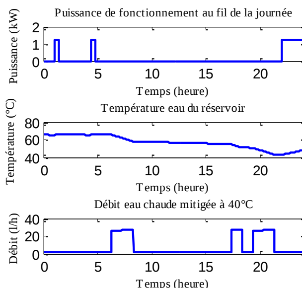
Figure 3-22 La puissance individuelle contrôlée par un chauffe-eau, la température de l'eau à l'intérieur du réservoir et la quantité de chaleur nécessaire pour préparer l'eau chaude.
