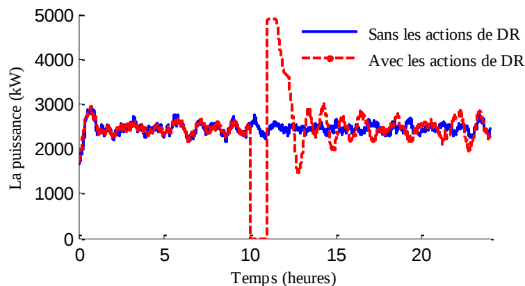
Figure 4-4 Les puissance non contrôlée et contrôlée par une coupure brutale d'une heure (de 10h à 11h) appliquée sur un parc de radiateurs et pour une température extérieure, T_{out} , égale à -5^{\circ}\text{C} .
