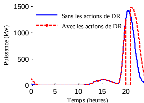
Figure 4-12 Le profil de recharge de 500 VEs sans et avec l'application d'un effacement d'une heure
