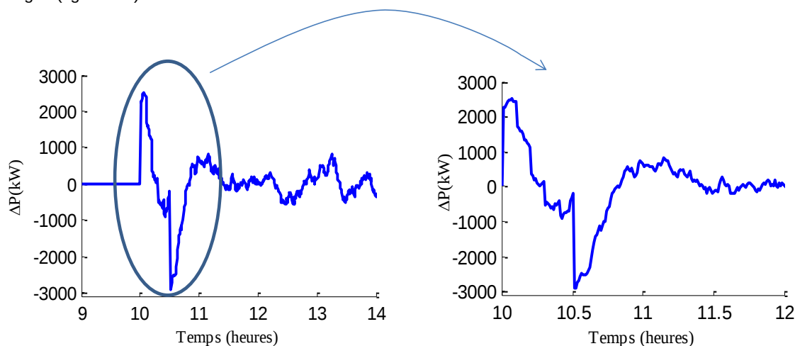
Figure 5-3 La puissance effacée par le cas dispatché.
