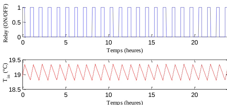
Figure 3-4 La puissance consommée d'un chauffage électrique avec un convecteur et l'évolution de la température à l'intérieur de la pièce, T_{in} pour une température T_{out} = -5^\circ\text{C} .
