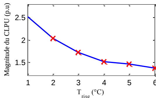
Figure 5-25 La magnitude du CLPU pour différentes valeur de T_{rise} .
