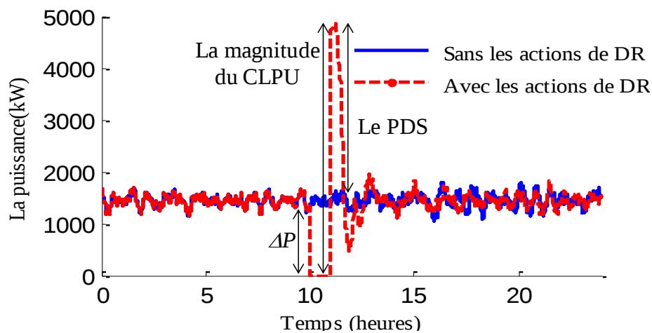
Figure 4-2 Les caractéristiques du CLPU qui résulte d'une coupure brutale d'une heure (de 10h à 11h) pour une température extérieure, T_{out} , égale à 5°C.
