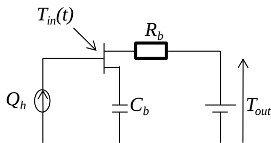
Figure 3-2 Le modèle de bâtiment (1 pièce) adopté dans l'étude.
