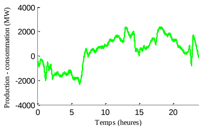
Figure 7-13 Le déficit de production et la surproduction créés au cours de la journée du 02/09/2012
