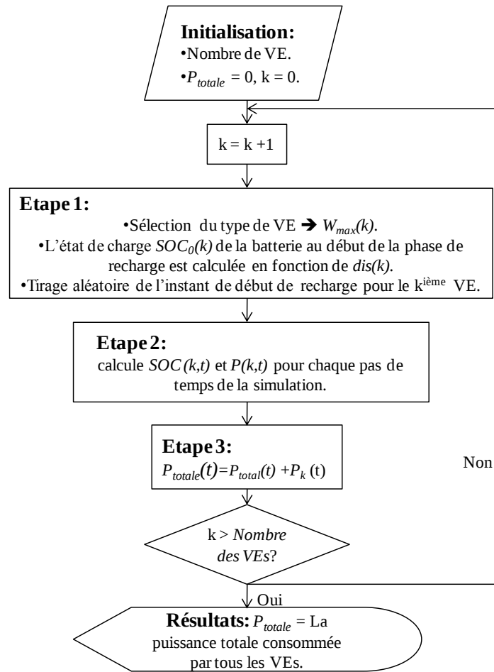
Figure 3-25 L'organigramme avec les différentes étapes de la simulation réalisées pour obtenir un profil de recharge du parc de VEs.
