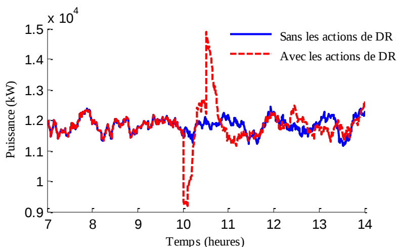
Figure 5-2 Puissance contrôlée et non contrôlée en cas d'application du cas dispatché sur la valeur initiale de N_1 , N_2 , N_3 , N_4 et N_5 .
