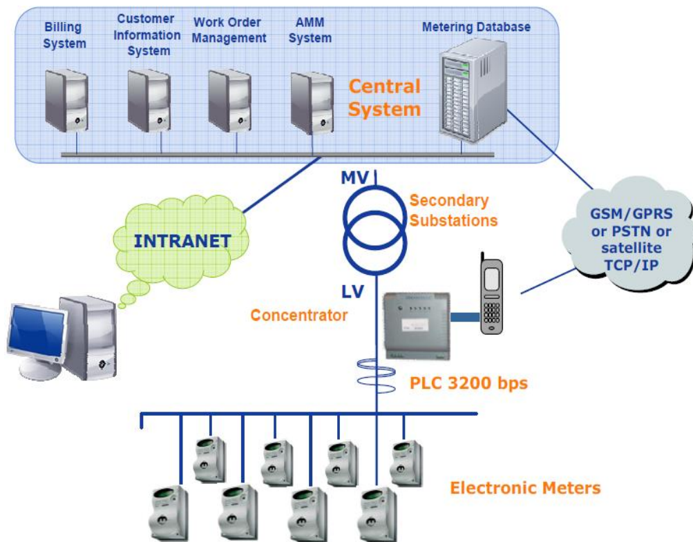
Figure 2-16 Infrastructure du projet Telegestore d'ENEL.
