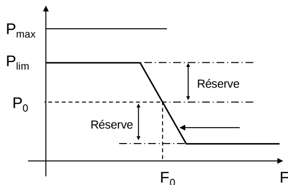
Figure 2-2 : courbe fréquence-puissance pour le réglage primaire
