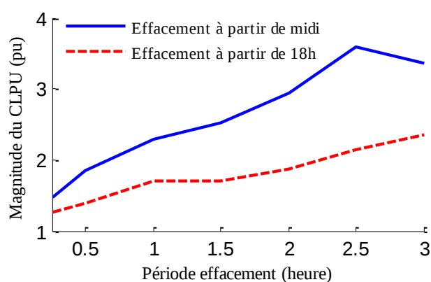
Figure 4-10 La relation entre la magnitude du CLPU et la durée de contrôle pour la première stratégie de contrôle (qui représente une coupure brutale de la consommation) appliquée sur un parc de 500 chauffages.
