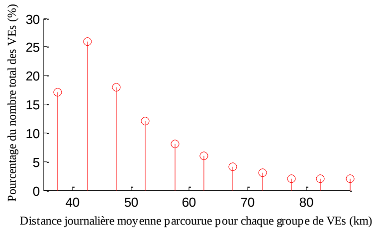
Figure 3-24 Les distances moyennes journalières parcourues pour chaque proportion de véhicules électriques du parc (500 VEs).
