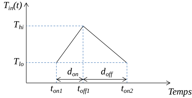
Figure 3-6 L'évolution de la température intérieure de la pièce, T_{in} , pendant un cycle de chauffe
