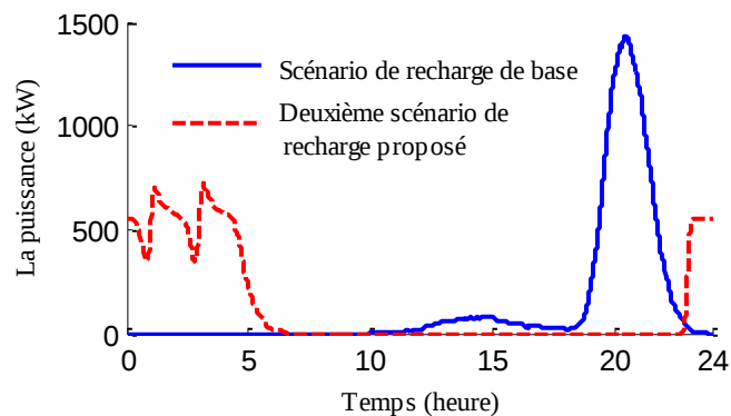
Figure 7-6 Comparaison entre le profil de recharge globale des 500 VEs selon le scénario de recharge de base et le profil de recharge selon le deuxième scénario de recharge.
