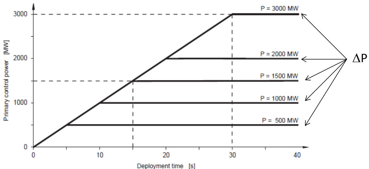
Figure 2-3 Le déploiement minimum de la réserve primaire de fréquence en fonction de la durée de la perturbation. [UCTE, 2004]
