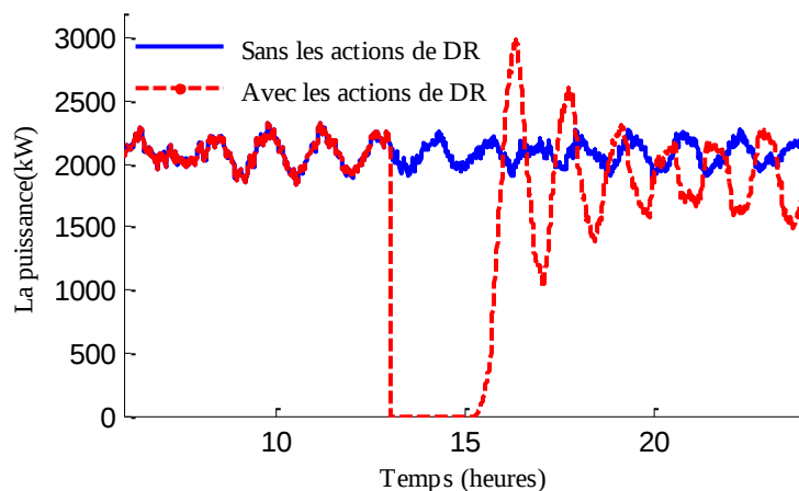
Figure 5-16 Oscillations observées après le CLPU pour 500 maisons bien isolées chauffées avec des convecteurs.
