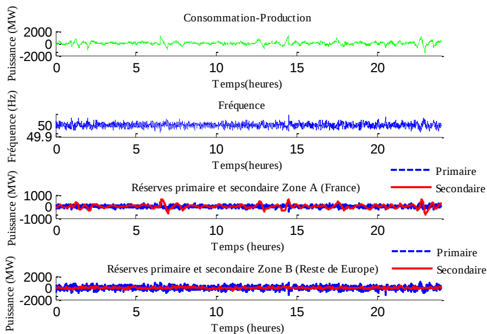
Figure 7-22 Le déséquilibre final entre la production et la consommation, l'évolution temporelle de la fréquence et les réserves primaires et secondaires libérées pour l'ajustement et pour un \Delta P = 200 MW dont le CLPU est contrôlé.
