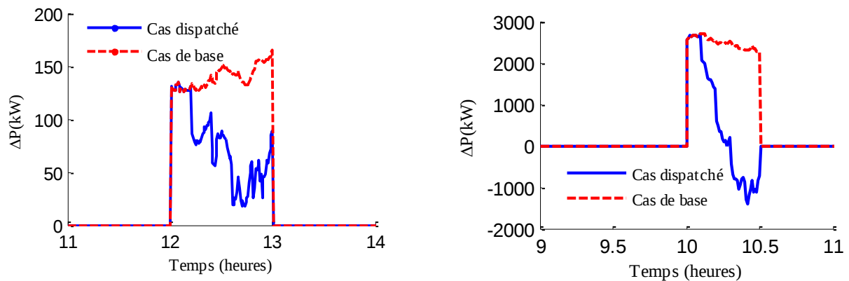
Figure 5-9 Comparaison entre la quantité effacée par le cas de base et par le cas dispatché en cachant l'effet du CLPU. Chauffe-eau (à gauche) et convecteur (à droite)
