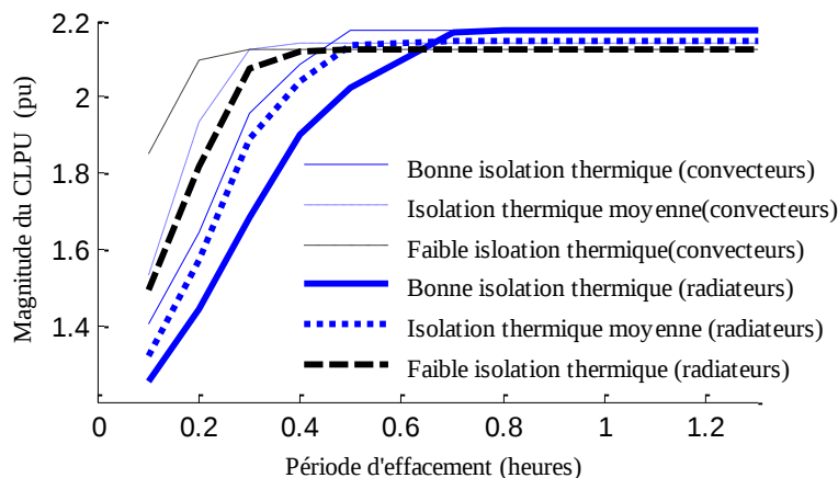
Figure 4-5 Les magnitudes du CLPU pour différentes périodes d'effacement et pour différents niveau d'isolation (pour une température extérieure, T_{out} égale à -5^{\circ}\text{C} ). Pour \Delta T_{DR} = 1 heure.
