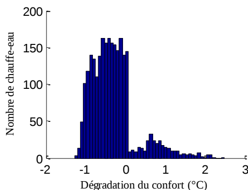
Figure 5-8 Les valeurs de dégradation de confort des 2500 chauffe-eau qui en résultent du cas dispatché.
