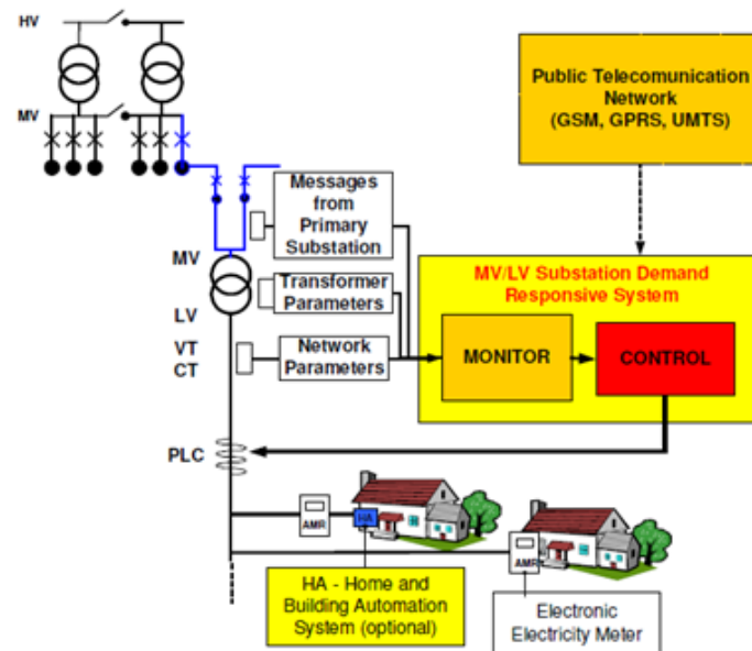
Figure 2-12 La structure d'un système de DR pour les réseaux de distribution.
