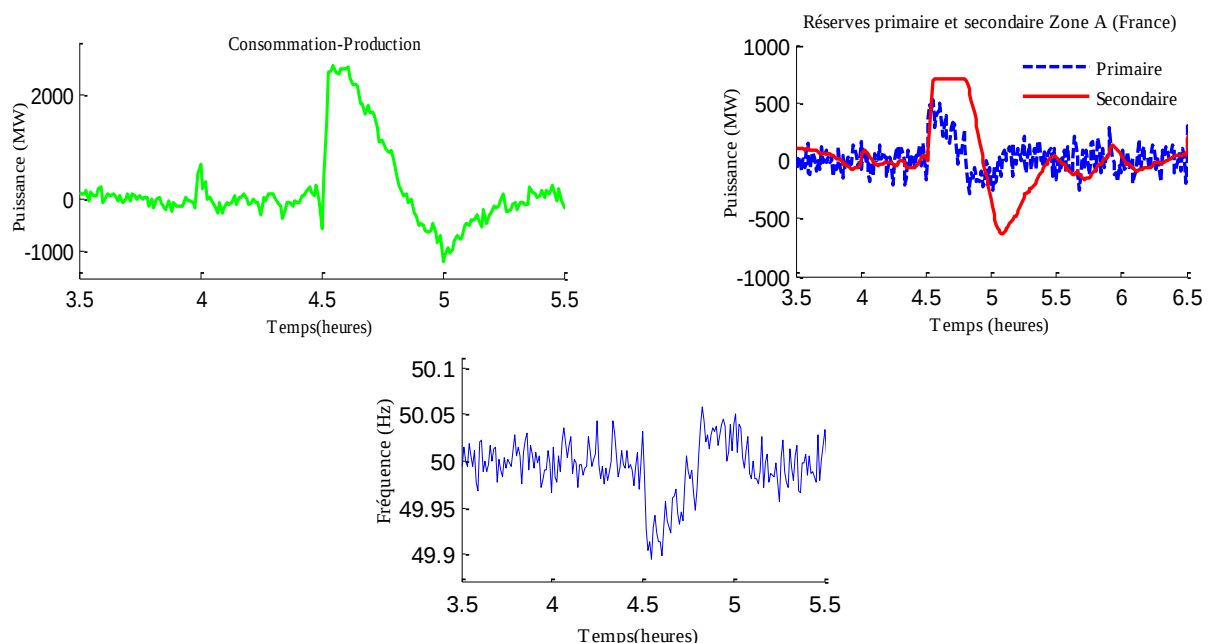
Figure 7-19 Le déséquilibre créé avec et participation de l'effacement de 4h à 4h30 (en haut à gauche) et la réserve secondaire mobilisée pour compenser le CLPU (en haut à droite) et l'évolution de la fréquence pendant l'heure qui suit l'effacement (en-dessous).
