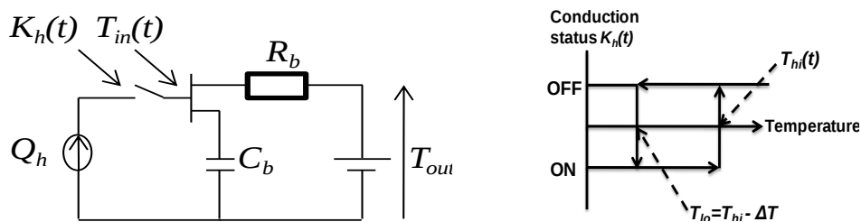
Figure 3-3 L'ensemble du modèle du bâtiment + élément de chauffage par convecteur, et logique de commande du relais
