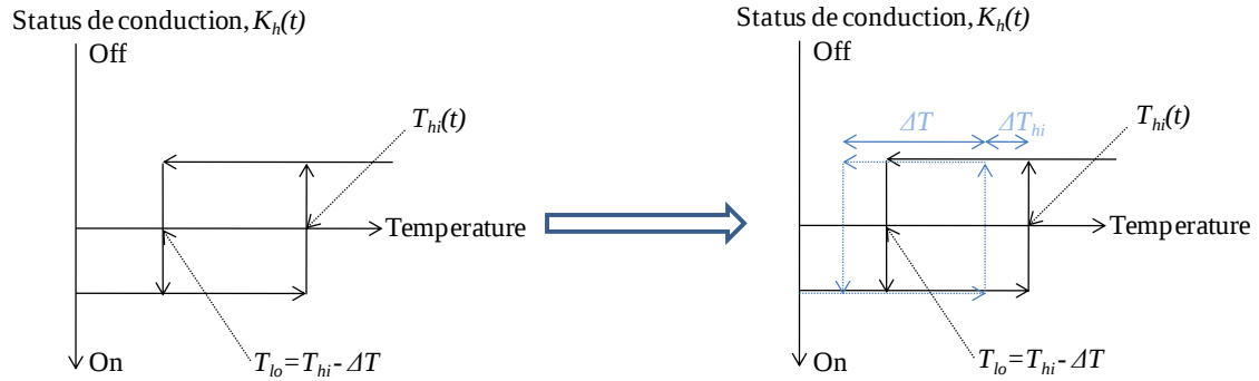
Figure 5-12 Variation de la consigne élevée du thermostat T_{hi} pendant l'application de la deuxième action de DR.
