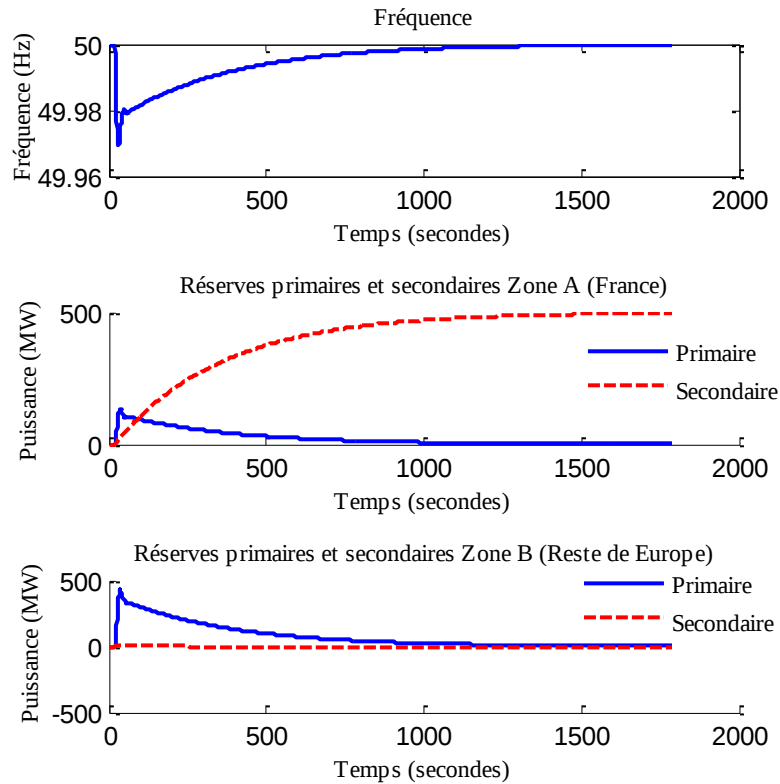
Figure 3-28 L'évolution temporelle de la fréquence ainsi que les réserves primaires et secondaires libérées de chaque zone.
