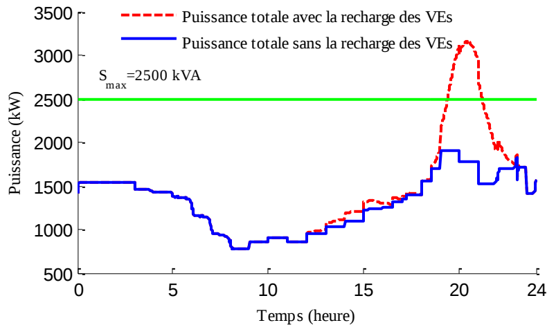
Figure 7-3 Le profil de consommation journalier des 780 maisons sans et avec la recharge des 500 véhicules électriques et en appliquant des actions de DR sur les 624 chauffe-eau.
