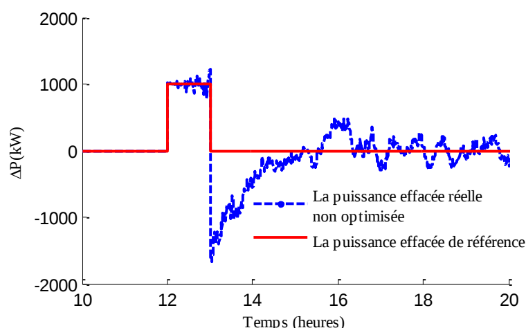
Figure 6-8 La puissance effacée réelle sans optimisation et la puissance de référence imposée dans l'optimisation.
