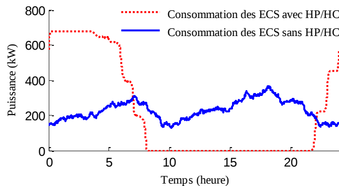
Figure 3-23 La consommation de 500 ECS sans et avec l'application de l'option HP/HC
