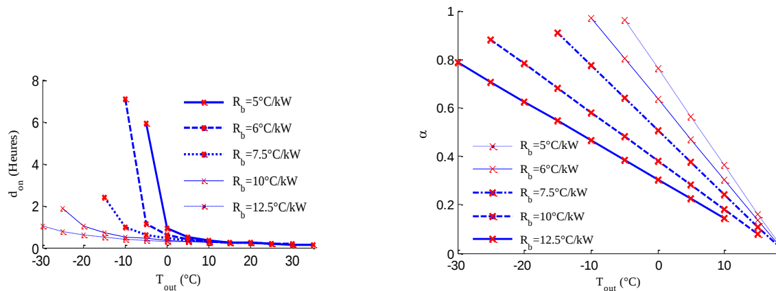
Figure 3-8 La relation entre la durée de chauffe, d_{on} , et la température extérieure du logement, T_{out} pour différentes valeurs de R_b .
