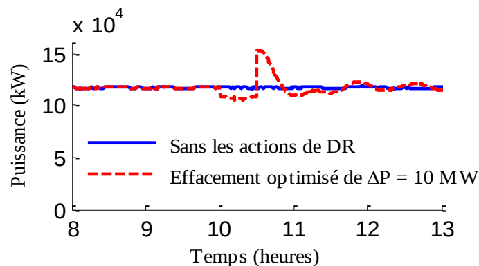
Figure 6-6 Le CLPU généré d'un effacement optimisé de 10 MW.
