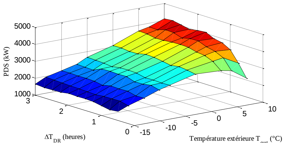
Figure 4-6 La relation entre le pic de surconsommation, la température extérieure T_{out} , et la durée d'effacement.
