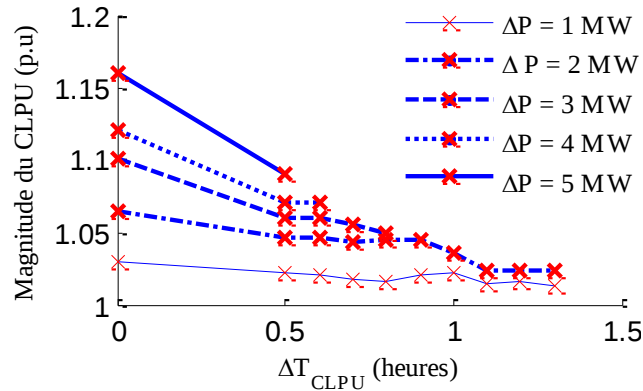
Figure 6-11 La magnitude du CLPU en fonction de \Delta T_{CLPU} pour différentes valeurs de \Delta P . T_{out} = -5^\circ\text{C} .
