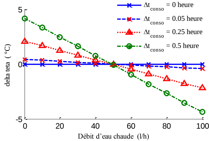
Figure 3-16 La relation entre le débit d'eau et le delta teta en phase de chauffe.
