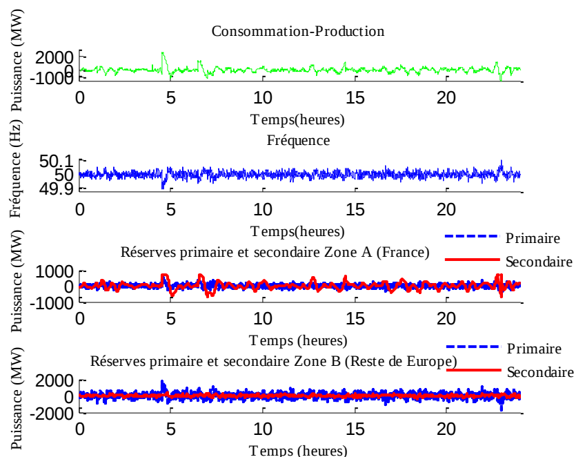
Figure 7-18 Le déséquilibre final entre la production et la consommation, l'évolution temporelle de la fréquence et les réserves primaires et secondaires libérées pour l'ajustement avec un bloc d'effacement \Delta P = 700 MW.
