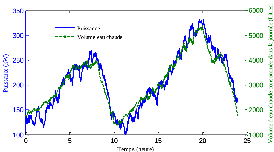
Figure 3-21 La demande de base journalière du chauffe-eau et le volume d'eau chaude utilisé pour 500 logements.
