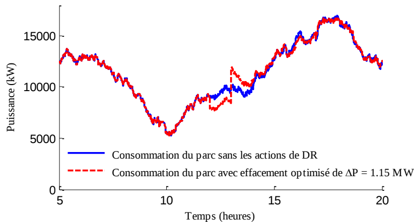
Figure 6-9 La consommation du parc des 25000 chauffe-eau sans et avec un effacement optimisée de midi à 13h.
