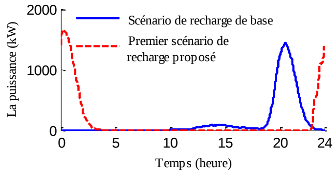
Figure 7-4 Comparaison entre le profil de recharge global des 500 VEs selon le scénario de recharge de base et le profil de recharge de ces VEs selon le premier scénario de recharge proposé.
