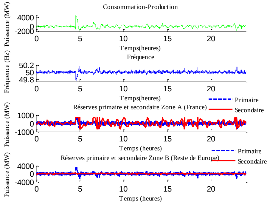
Figure 7-20 Le déséquilibre final entre la production et la consommation, l'évolution temporelle de la fréquence et les réserves primaires et secondaires libérées pour l'ajustement et pour un \Delta P égal à 1400 MW
