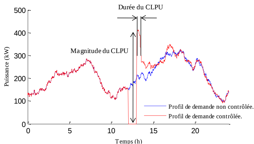
Figure 4-8 Caractéristiques du CLPU qui apparaît suite à une heure de coupure brutale d'un parc de 500 chauffe-eau.
