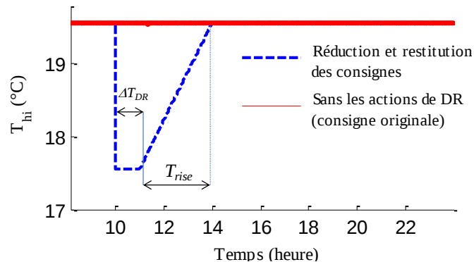
Figure 5-21 La variation des consignes du thermostat avec une restitution des consignes initiales en pente.
