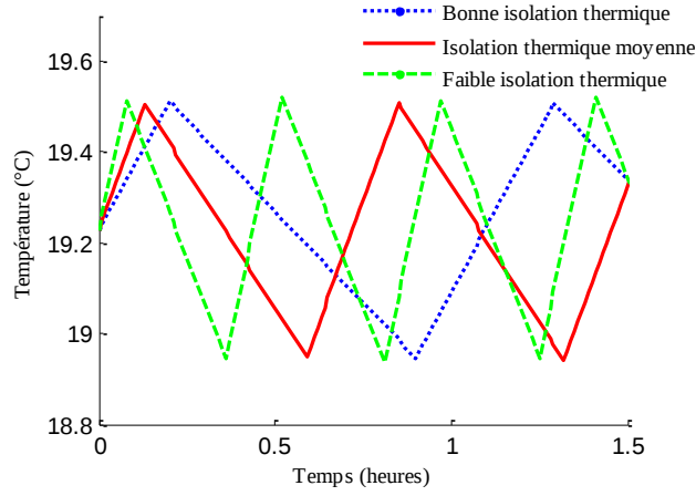
Figure 3-5 Evolution de la température intérieure de la pièce à chauffer pour chaque niveau d'isolation.
