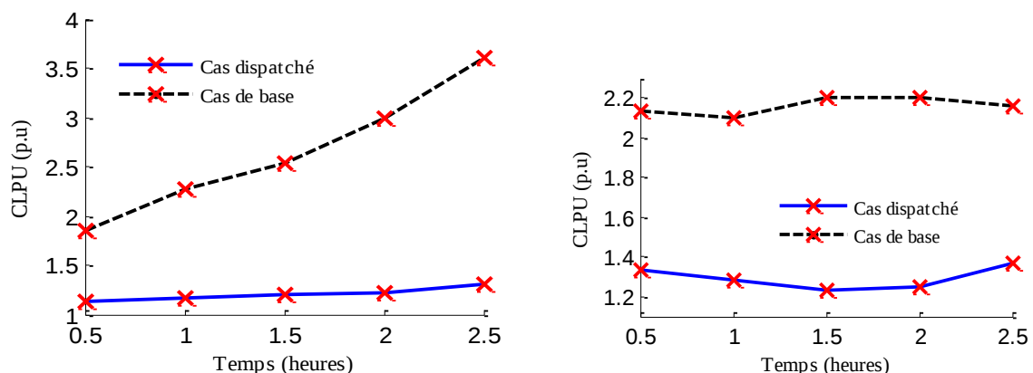
Figure 5-10 Magnitudes de CLPU obtenues pour les deux scenarios de coupure et pour différentes périodes de coupures ( \Delta T_{DR} ). Pour les convecteurs (à droite) et pour les chauffe-eau (à gauche).
