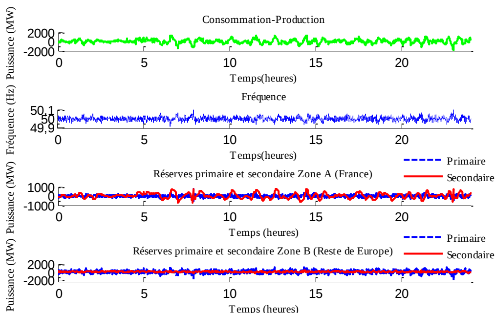
Figure 7-23 Le déséquilibre final entre la production et la consommation, l'évolution temporelle de la fréquence et les réserves primaires et secondaires libérées pour l'ajustement et pour un \Delta P = 700 MW dont le CLPU est contrôlé.
