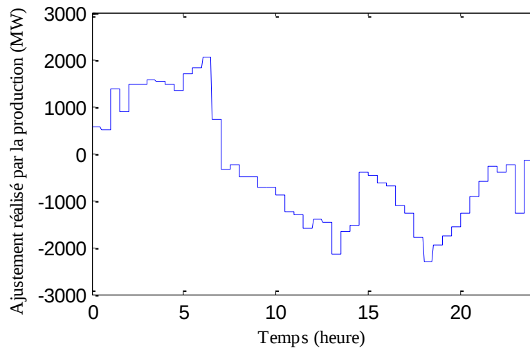
Figure 7-14 L'ajustement fourni par la production conventionnelle, en forme de marches d'escaliers de 30 minutes.
