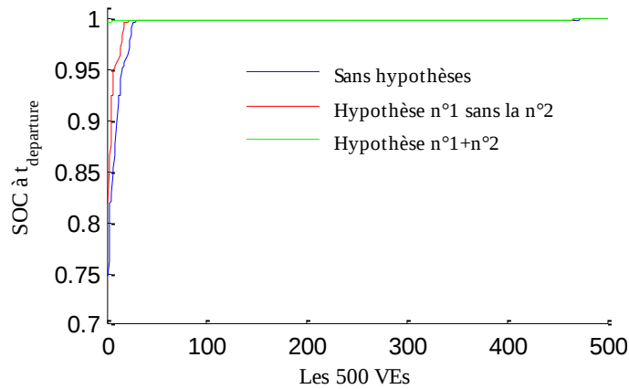
Figure 7-8 Les états de charges, SOC des 500 VEs à l'instant t_{departure} sans et avec l'application des hypothèses.
