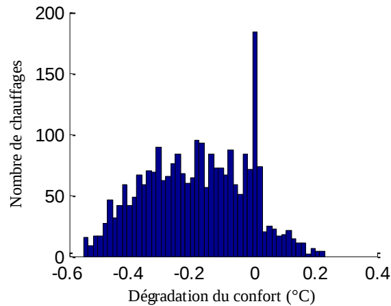
Figure 5-4 Valeurs de dégradation du confort thermique des 2500 chauffages contrôlés.
