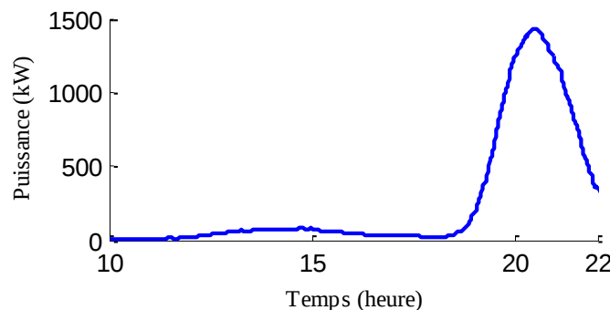
Figure 7-2 Le profil de recharge de base de 500 VEs.
