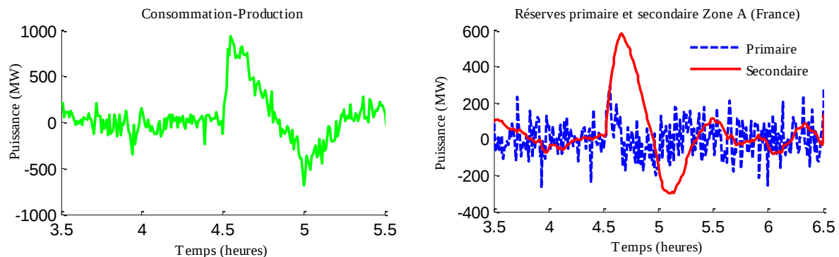
Figure 7-17 Le déséquilibre créé avec la participation de l'effacement de 4h à 4h30 (à gauche) et la réserve secondaire mobilisée pour compenser le CLPU (à droite).
