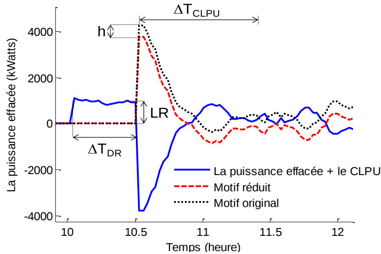
Figure 6-10 Le profil réel de la puissance effacée et le profil de référence de l'optimisation en rouge.
