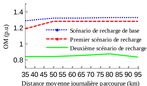
Figure 7-9 Le rapport de surcharge en fonction de la distance moyenne journalière parcourue.
