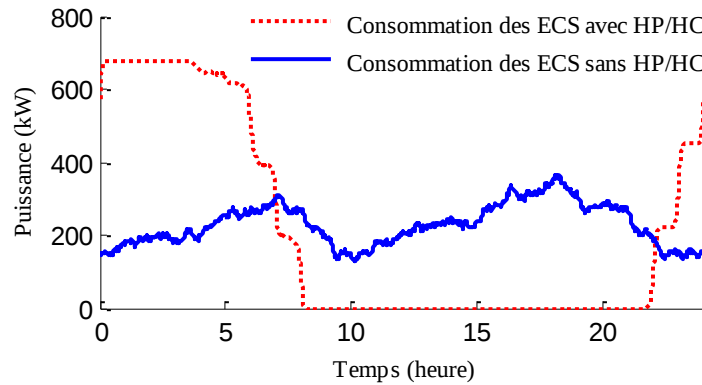
Figure 7-1 La demande des 624 chauffe-eau sans et avec l'application de actions de DR.
