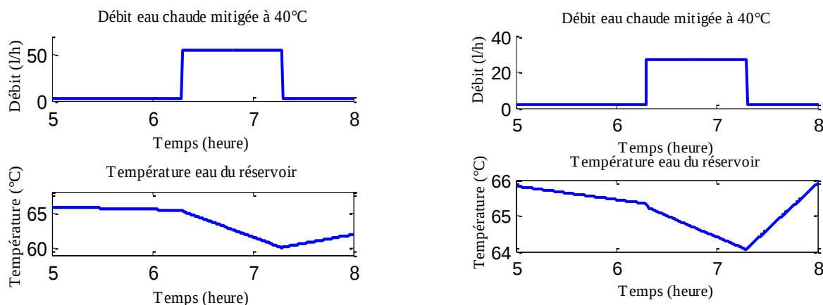
Figure 3-20 L'évolution de la température d'eau chaude pour deux valeurs de débit.
