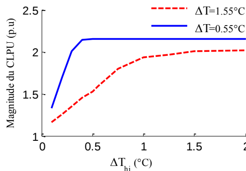
Figure 5-14 La magnitude du CLPU qui résulte de l'application de différentes valeurs de \Delta T_{hi} et pour deux valeurs de la bande morte du thermostat ( \Delta T ) pour \Delta T_{DR}=1 heure et pour T_{out} = -5^{\circ}\text{C} .
