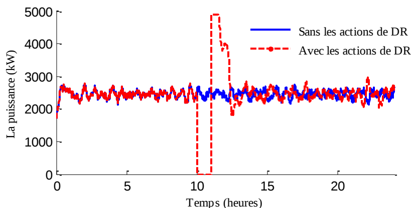
Figure 4-3 Le phénomène du CLPU qui résulte d'une coupure brutale d'une heure (de 10h à 11h) pour une température extérieure, T_{out} , égale à -5^{\circ}\text{C} .
