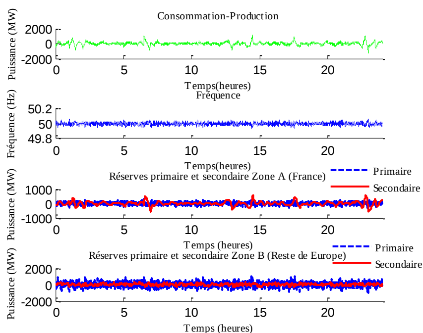
Figure 7-15 L'évolution temporelle de la fréquence, et les réserves primaires et secondaires libérées pour rééquilibrer la demande et la production.
