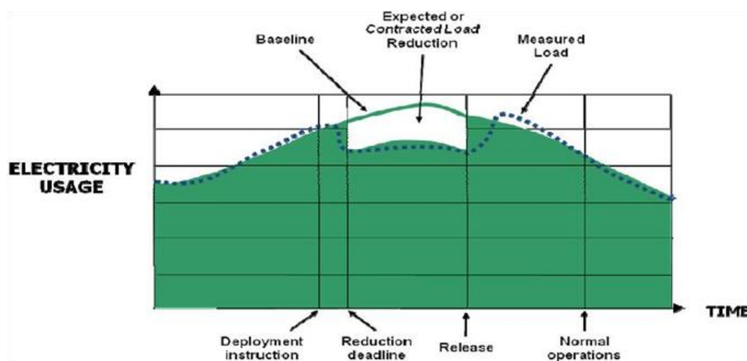
Figure 2-11 Un exemple sur la Baseline. [AEIC, 2009].
