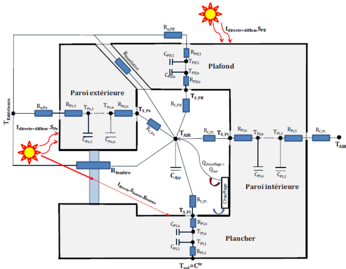
Figure 3-1 Schéma du modèle électrothermique du bâtiment utilisé par [Da_Silva, 2011]
