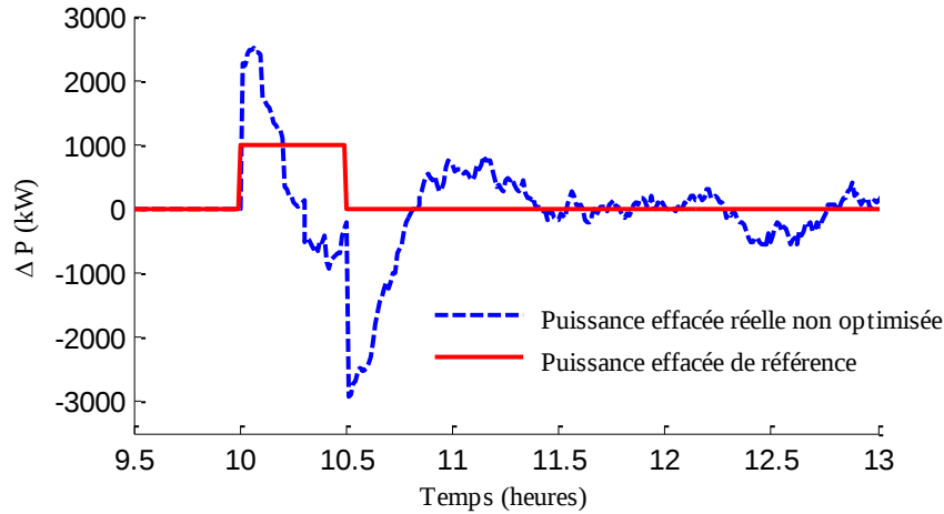
Figure 6-3 Le profil de puissance de référence et le profil de puissance effacée non optimisé à optimiser (qui résulte du contrôle ON/OFF de 500 charges dans chaque groupe). T_{out} = -5^{\circ}\text{C}
