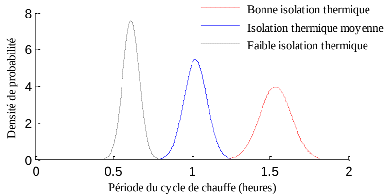
Figure 3-13 Distribution of des périodes de cycle de chauffe d'un parc de logement avec convecteurs.
