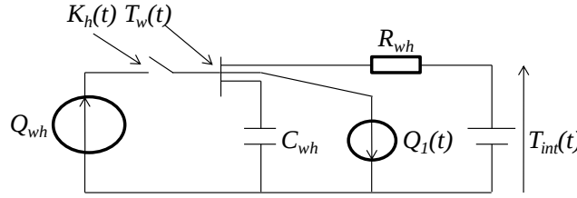
Figure 3-14 Modèle physique d'un chauffe-eau.
