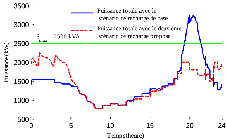
Figure 7-7 Les profils de consommation journaliers des 780 logements avec la demande des 500 VEs premièrement en les rechargeant avec le scénario de recharge de base et deuxièmement en les rechargeant avec le deuxième scénario de recharge.
