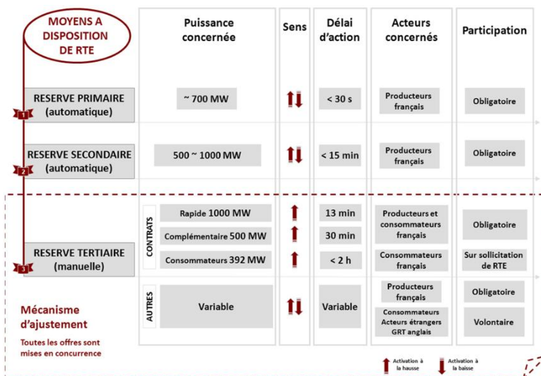
Figure 2-7 Récapitulatif des réserves de puissance pour le réglage de fréquence.
