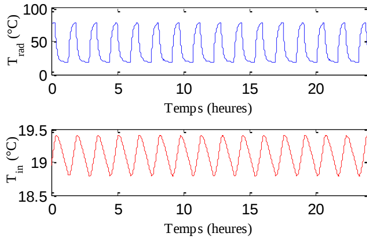
Figure 3-10 L'évolution de la température du cœur de chauffe, T_{rad} ainsi que celle à l'intérieur de la pièce à chauffer, T_{in} .
