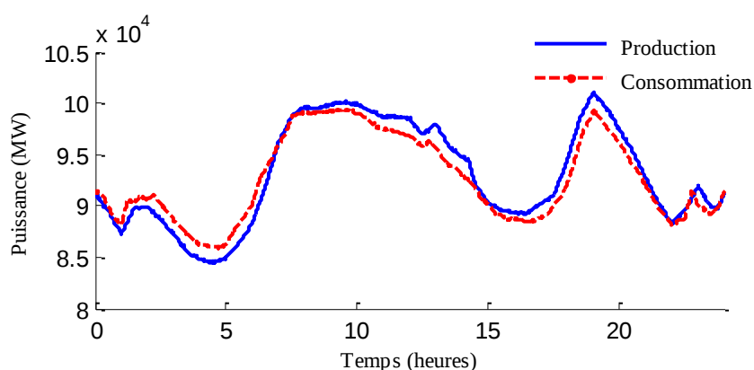
Figure 7-12 Le profil sous-échantillonné de la puissance en France dans la journée du 09/02/2012
