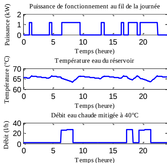
Figure 3-19 La vitesse de baisse de la température d'eau chaude dans le réservoir en cas de fonctionnement au fil de la journée.
