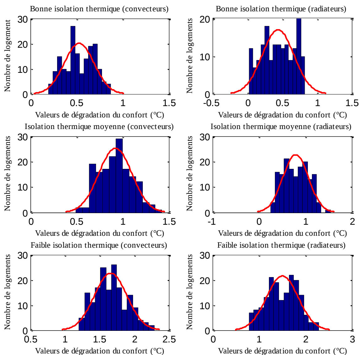
Figure 4-7 Distribution des valeurs de dégradation de confort thermique dans les 500 logements pour les deux cas d'étude, pour les différents niveaux d'isolation et pour T_{out} = -5^{\circ}\text{C} .
