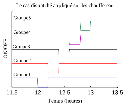
Figure 5-5 Le cas dispatché appliqué sur les chauffe-eau.
