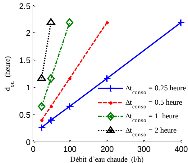
Figure 3-17 La durée d_{on} en fonction du débit d'eau chaude pour un volume d'eau soutiré de 100l.
