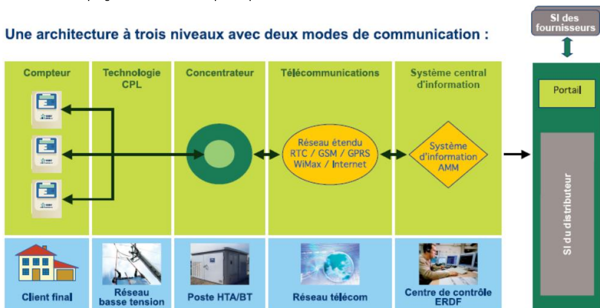
Figure 2-17 Architecture du projet de pilotage ERDF (SI=Systeme d'Information).
