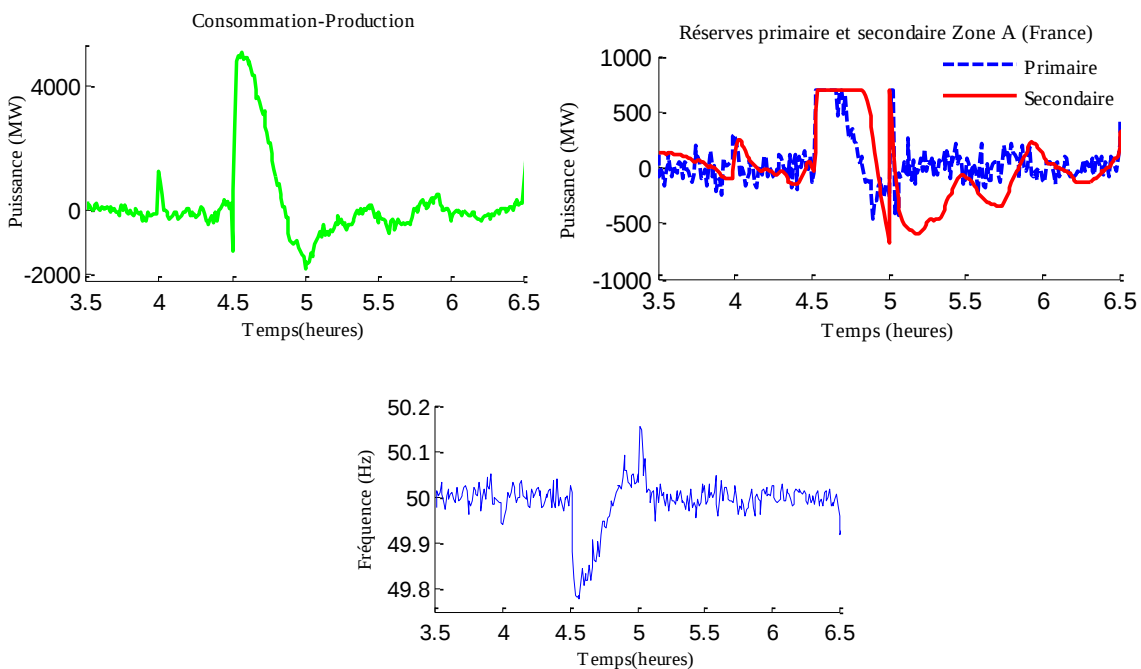
Figure 7-21 Le déséquilibre créé avec et participation de l'effacement de 4h à 4h30 (en haut à gauche) et la réserve secondaire mobilisée pour compenser le CLPU (en haut à droite) et l'évolution de la fréquence pendant l'heure qui suit l'effacement (en-dessous).
