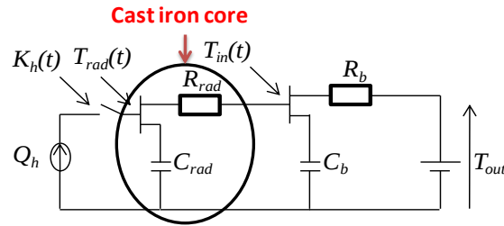
Figure 3-9 Model physique d'un radiateur à inertie
