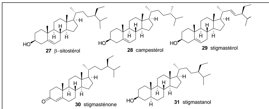
Figure 1-6. Stérols isolés des rhizomes d' A. sceptrum .
