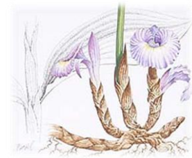
Aframomum sceptrum K. Schum. Dessin de B. Smith
