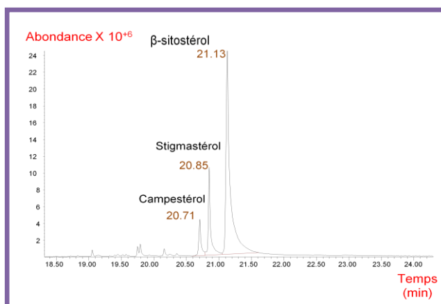
Figure 1-9. Chromatogramme du mélange de stérols analysé par GC-MS après silylation.
