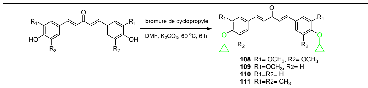
Figure 2-21. Analogues cyclopropoxy diénoniques de la curcumine (Chandru et al. , 2007 ).
