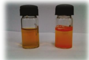
Figure 2-15. Solubilité de la nanocurcumine (à gauche) et de la curcumine (à droite) dans l'eau (Bhawana et al. , 2011).
