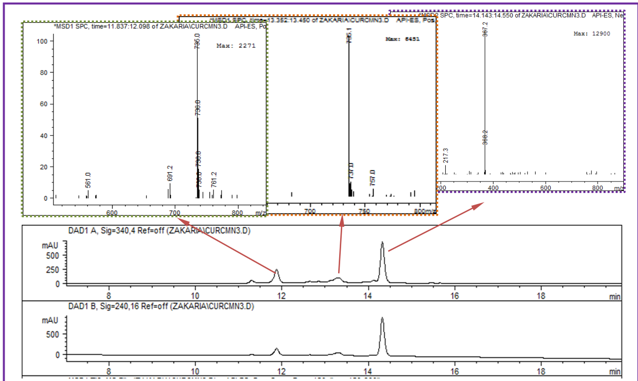
Chromatogramme 4-1. Le Chromatogramme du couplage homodimérique en présence de \text{MnO}_2+\text{Mn}(\text{OAc})_3 .
