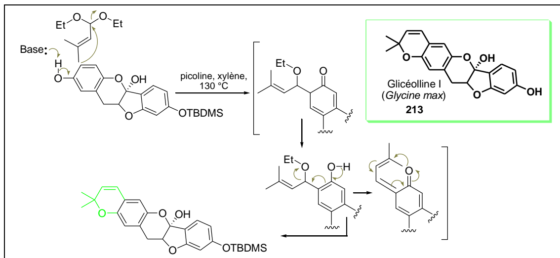
Schéma 3-15. Synthèse de diméthylbenzopyranes développée pour la synthèse de la glycéolline I 213 basée sur une condensation aldolique modifiée.
