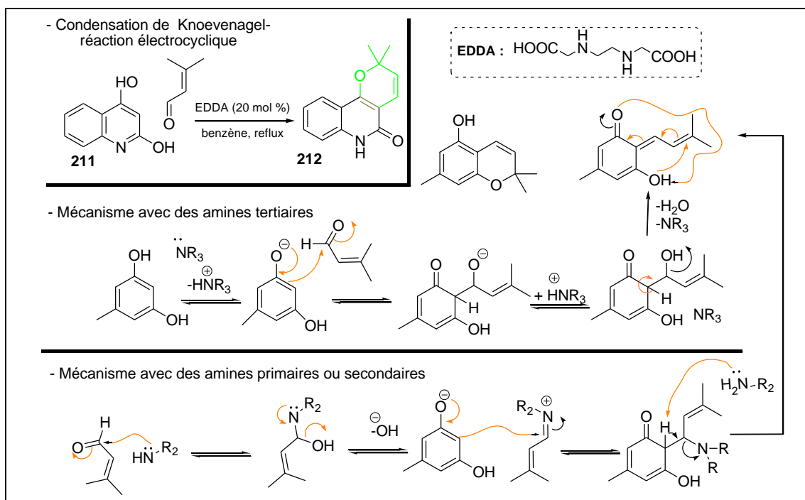
Schéma 3-14. Synthèse de benzopyrane développée par le groupe de Lee : une réaction tandem avec une condensation de Knoevenagel organocatalysée et une réaction électrocyclique.
