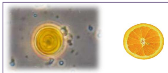
Figure 2-14. Vue microscopique du complexe curcumine-phospholipide grossi 400 fois.
