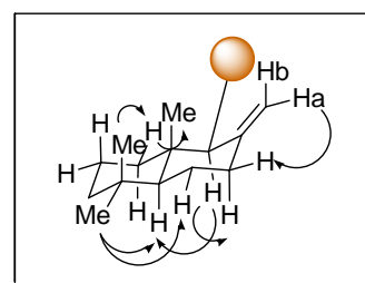
Figure 1-11. Corrélations NOESY observées pour la partie terpénique
