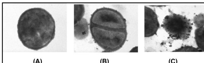
Figure 2-16. Images de MET (A) cellules de S. aureus (contrôle, non traité) (B) S. aureus traité avec des nanoparticules de curcumine, avec l'ancrage de la curcumine nanoparticulaire à la paroi cellulaire, (C) attaque des nanoparticules curcumine, perturbation de la paroi cellulaire (couche de peptidoglycane), et pénétration des nanocurcumines à l'intérieur de la cellule (Bhawana et al. , 2011).
