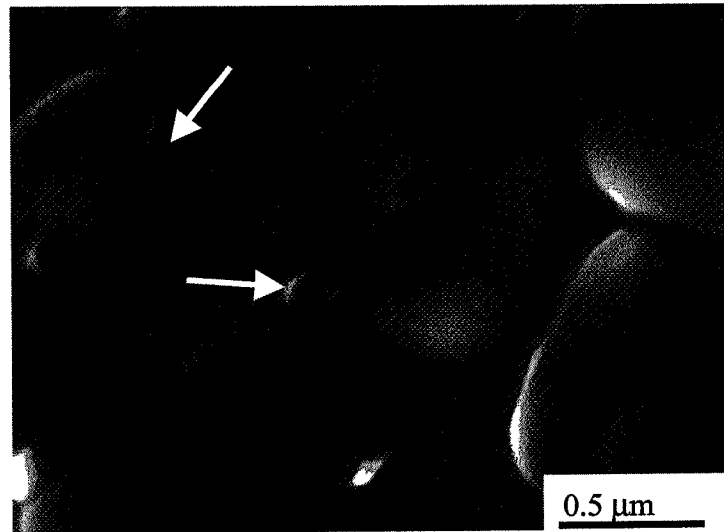
Figure 4.45 Micrographie SEM de la poudre YSZ MC post-BM et EPD et soumise à traitement thermique à 1550°C
