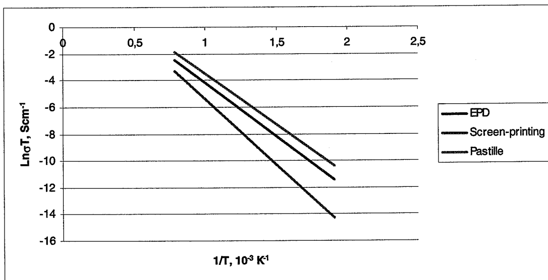
Figure 4.46 Courbes d'Arrhenius pour les doubles couches sérigraphiques et les monocouches électrophorétiques traitées à 1200°C et pour la pastille traitée à 1550°C.
