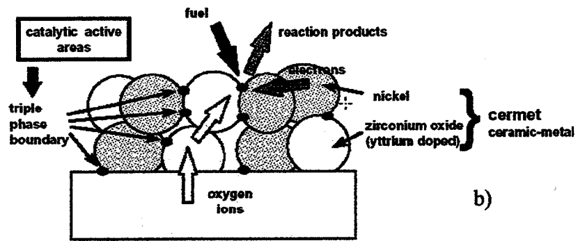
Figura 1.73 (a) Reazioni di riduzione di ossigeno per un conduttore puro e per uno misto (b) caso specifico del cermet Ni-YSZ 221
