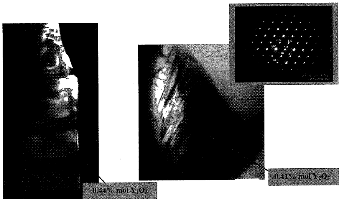
Figure 5.23 Micrographies MET de grains de zirconne accolés au substrat et cliché de diffraction indexé dans la phase monoclinique (JCPDS 37-1484) en axe de zone [1-11]. Le taux d'yttrine obtenu par analyse EDX est aussi reporté.
