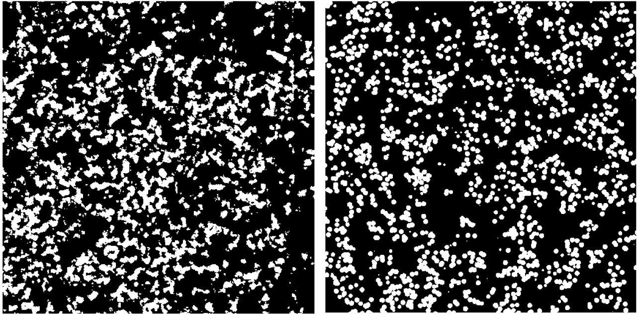
FIG. 5.35 – Comparaison d’une image réelle de taille 3.6 \times 3.6 \mu\text{m}^2 d’une lame mince de l’échantillon chargé à 13.96% en noir de la série A (à gauche) et d’une image simulée (à droite)
