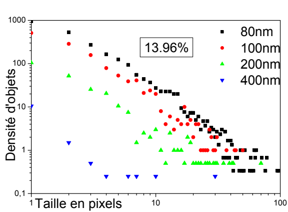
C8 - Distributions des objets suivant leur taille de quatre concentrations de la série C. Un graphique par concentration, une série par épaisseur.
