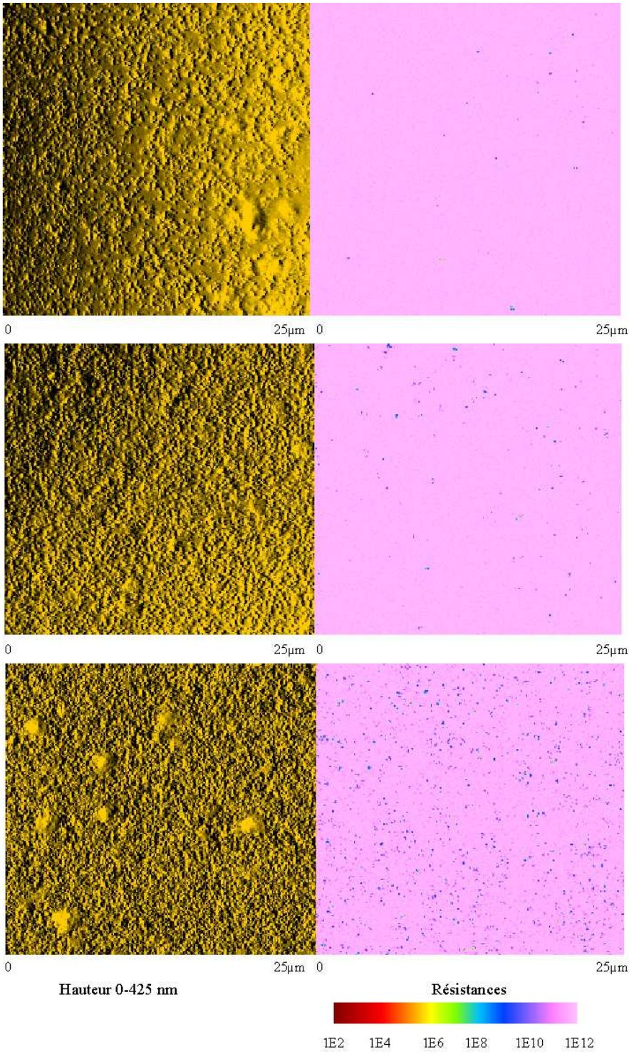
B1 - Couple d'images topographie/résistance de trois échantillons de la série A chargé à 7.97%(en haut), 12.47%(au milieu) et 21.69% (en bas) en noir à une épaisseur de 100 nm
