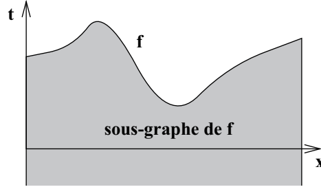
FIGURE A.1 – Sous-graphe d’une fonction f (Vachier, 1995).
