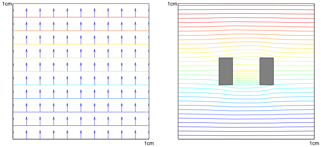
(a) Équipotentielles dans une cellule unitaire vide (b) Équipotentielles dans une cellule contenant un anneau de section carrée (en gris)
