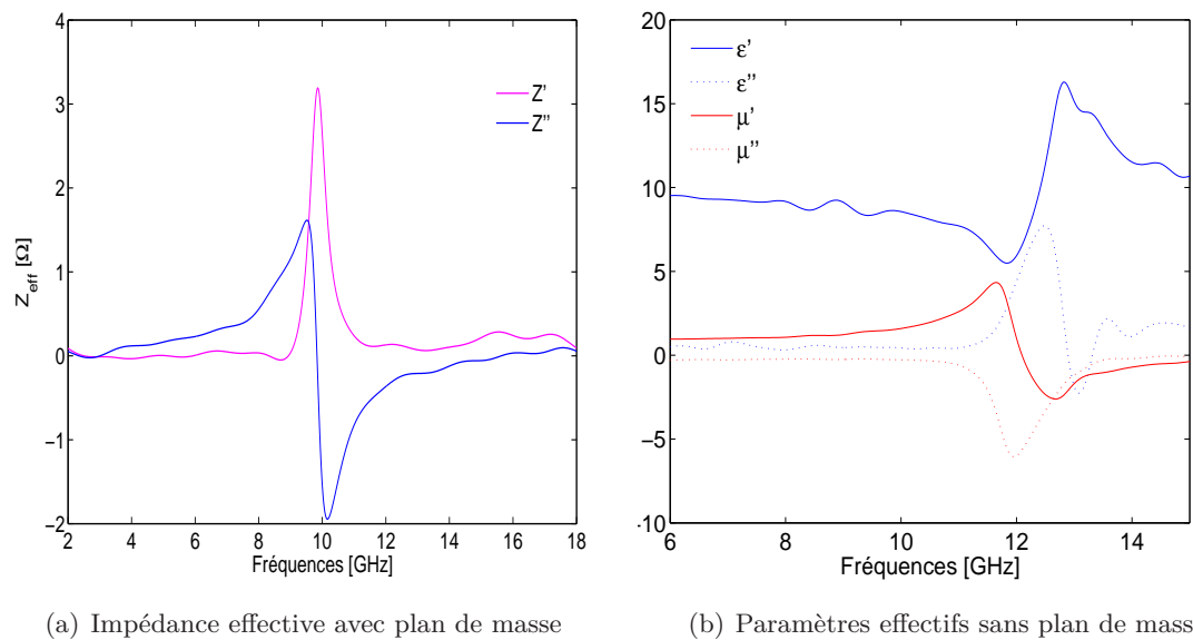
FIGURE 69 – Paramètres effectifs d'un réseau de "mushrooms" avec et sans plan de masse
