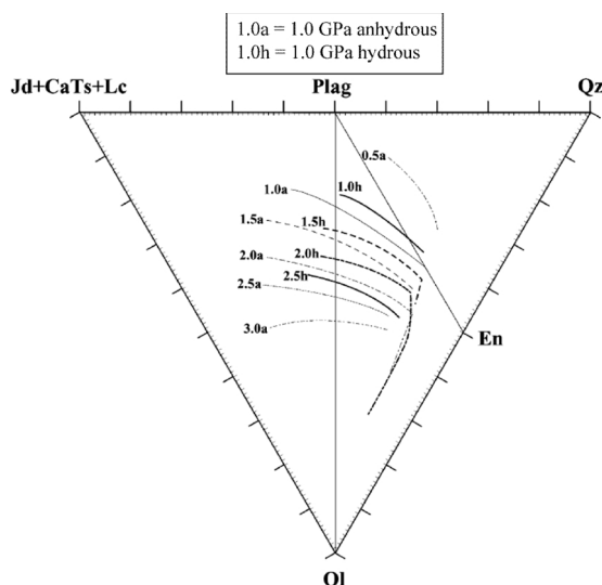
Figure I.12. Projection dans le plan [Jd+CaTa+Lc]-Plag-Qz du tétraèdre normatif, d'après Ulmer (2001), illustrant le décalage des cotectiques ol + opx + (cpx) des expériences entre 0,5 et 3 GPa en conditions anhydres (a) et hydratées (h). la courbe qui se rapproche du pôle olivine connecte les compositions uniquement saturées en olivine. La ligne Ol-Plag représente le plan de sous-saturation en silice.
