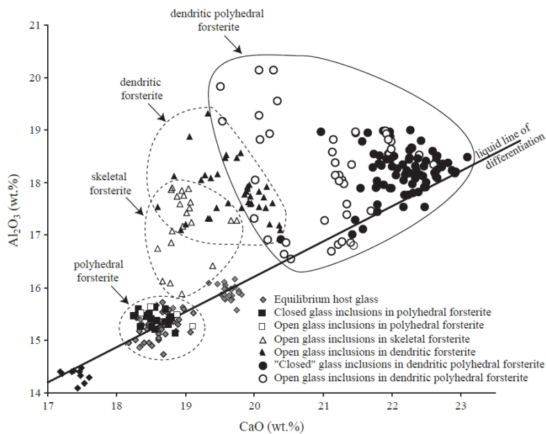
Figure II.02. Figure montrant les concentrations en Al_2O_3 et CaO des verres et des inclusions synthétisés lors des expériences de cristallisation dynamique de forstérites automorphes, dendritiques et squelettiques de Faure et Schiano (2005). Les compositions des inclusions magmatiques sont comparées à la ligne de différenciation définie à partir des verres basaltiques.
