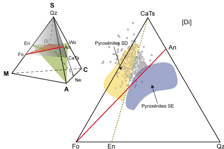
Figure I.15. Tétrahédre CMAS et projection par le pôle diopside dans le plan CaTs-Fo-Qz (plan gris du tétraèdre) montrant le plan de sous-saturation en silice Di-Fo-An (plan et ligne rouge) et la division thermique des pyroxènes alumineux, effective à P > 2 GPa pour les pyroxénites et leur liquides dérivés (plan et ligne pointillée verts), qui sépare les pyroxénites déficitaires en silice (SD : surface jaune) et les pyroxénites excédentaires en silice (SE : surface bleue). Les champs des pyroxénites ont été déterminés par Lambart et al. (2013). Les inclusions primitives (points gris) sont reportées pour comparaison.
