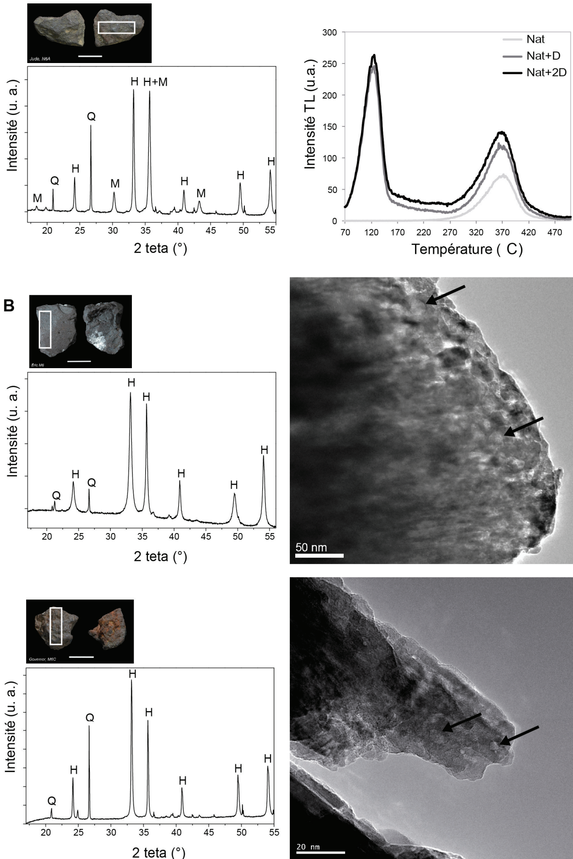
Figure 72 – Indices de chauffage décelés par DRX, TL et MET, dans trois pièces de ferricrètes. Hématite et maghémite, courbes de TL avec croissance en dose du signal : chauffé (A). Hématite avec élargissement anisotrope des raies, pores dans les cristaux: chauffage de goethite (B). Hématite et pores dans les cristaux : chauffage de goethite (C). Barre d'échelle photos : 1 cm.
