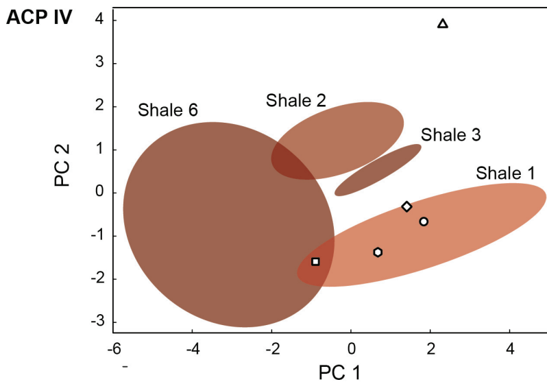
Figure 38 - Attribution de 5 échantillons archéologiques selon l'ACP IV réalisées sur une sélection de logs de rapports éléments traces sur le fer. Répartition des sources de shale.
