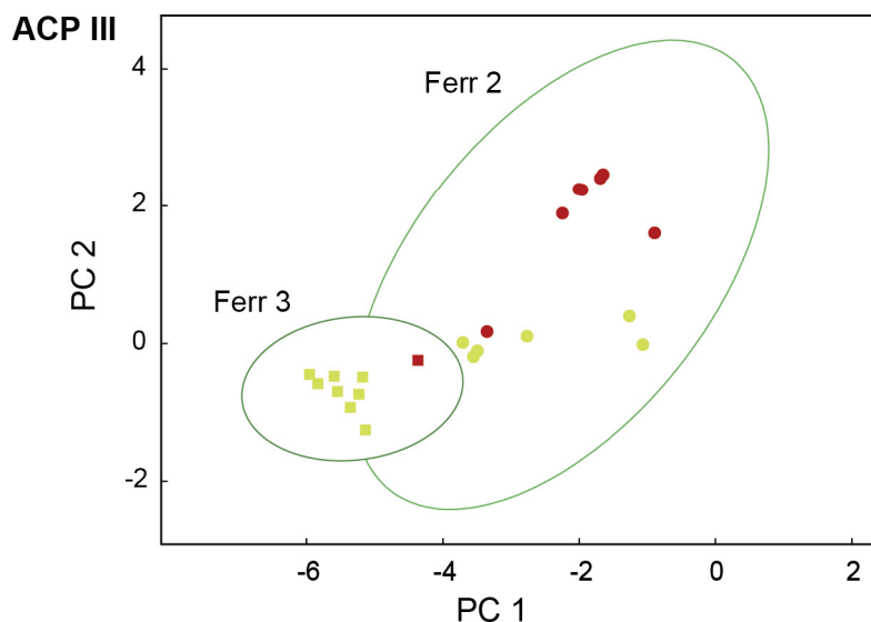
Figure 41 – Répartition des échantillons riches en goéthite (jaune) ou en hématite (rouge) dans les sources de ferricrètes.
