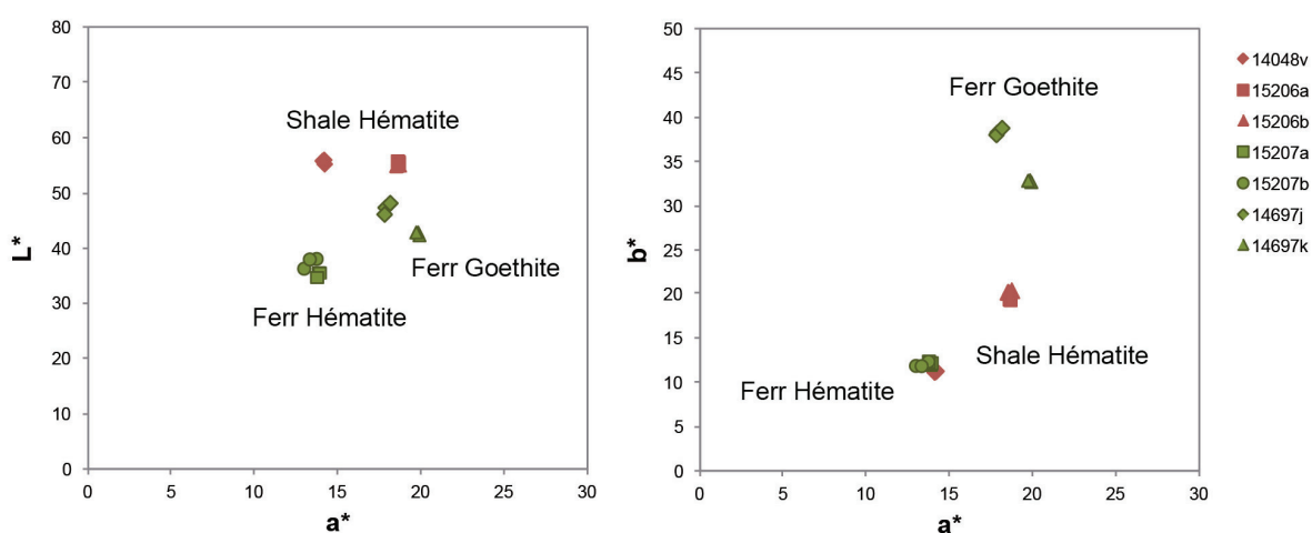
Figure 79 – Diagrammes binaires de coordonnées L^* et a^* , ainsi que des coordonnées a^* et b^* de différents échantillons géologiques, shales (rouge) ou ferricrètes (vert), à base de goethite ou d'hématite.
