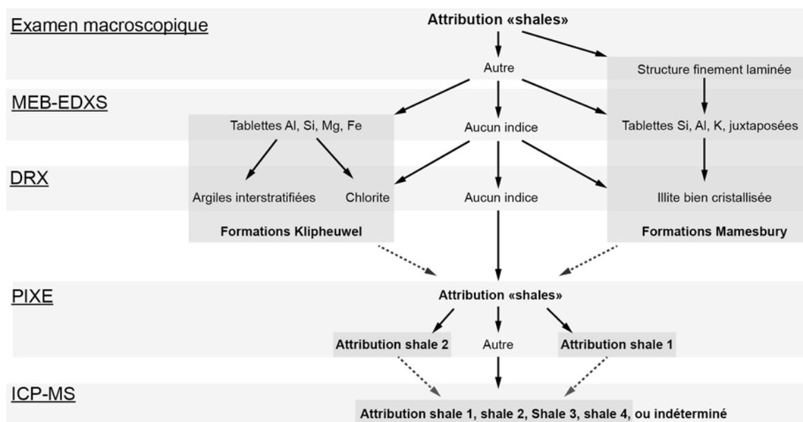
Figure 46 – Schéma de synthèse établi à partir de différentes méthodes pour déterminer la provenance ou l'origine géologique d'ocre (shales) dans le contexte proche de Diepkloof Rock Shelter, Afrique du Sud.
