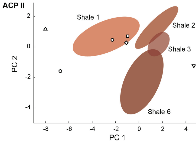
Figure 37 – Attribution de 5 échantillons archéologiques selon l'ACP II sur une sélection d'éléments traces. Répartition des sources de shale.
