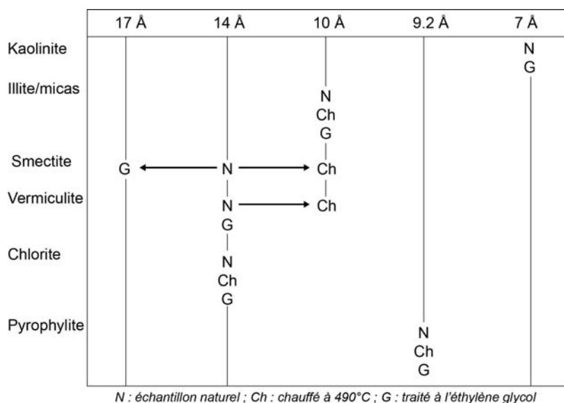
Figure 4 – Position de la raie principale des différentes familles d'argiles, utilisée pour leur identification d'après Millot, 1964, et Moore et Reynolds, 1980).
