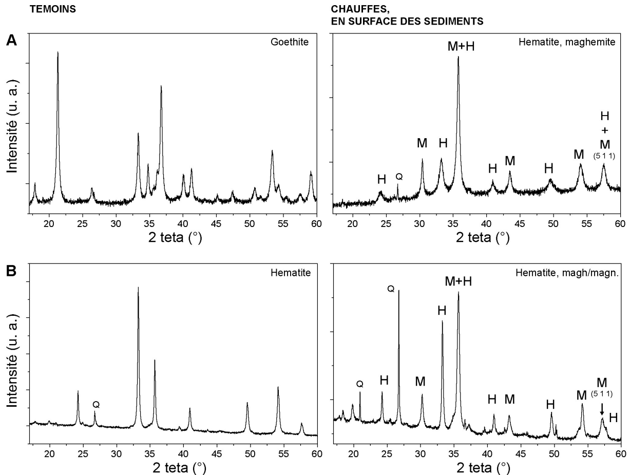
Figure 51 – Diffractogramme montrant les différentes transformations thermiques pouvant se produire lorsqu'une pièce est placée en surface des sédiments, directement sous le feu. Nodule de goethite (source Ferr 1) se transformant en hématite et maghémite (A) ; nodule d'hématite (source Ferr 5) se transformant en une phase intermédiaire entre maghémite et magnétite (B).
