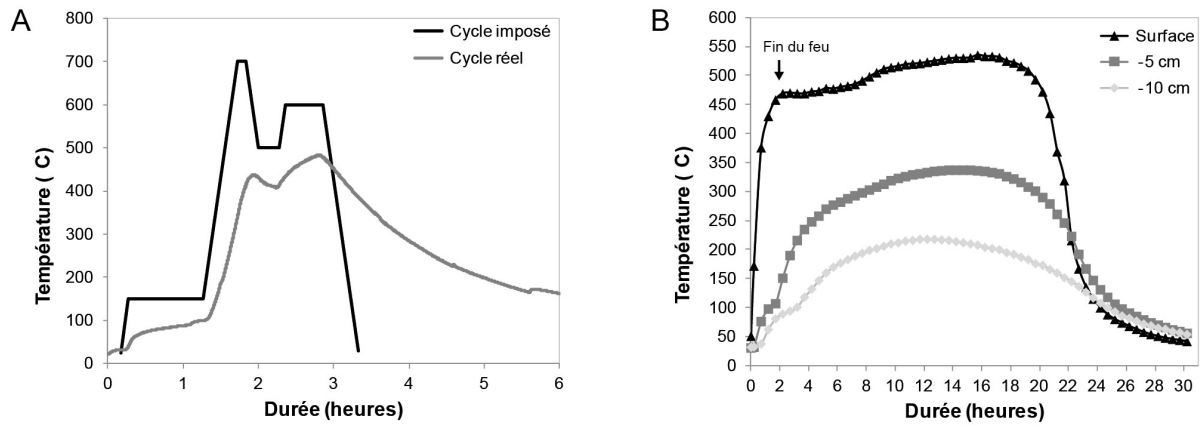
Figure 47 – Cycle thermique imposé aux échantillons expérimentaux dans un four à moufle (A) et températures enregistrées à l’aplomb du feu expérimental, à la surface des sédiments, à 5 cm et à 10 cm en dessous du foyer (B).
