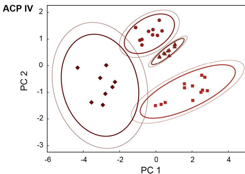
Figure 34 - Composantes 1 et 2 de l'ACP IV réalisées sur les logs des rapports au fer des éléments As, Ba, Cr, Sb et V, discrimination entre les sources de shale.
