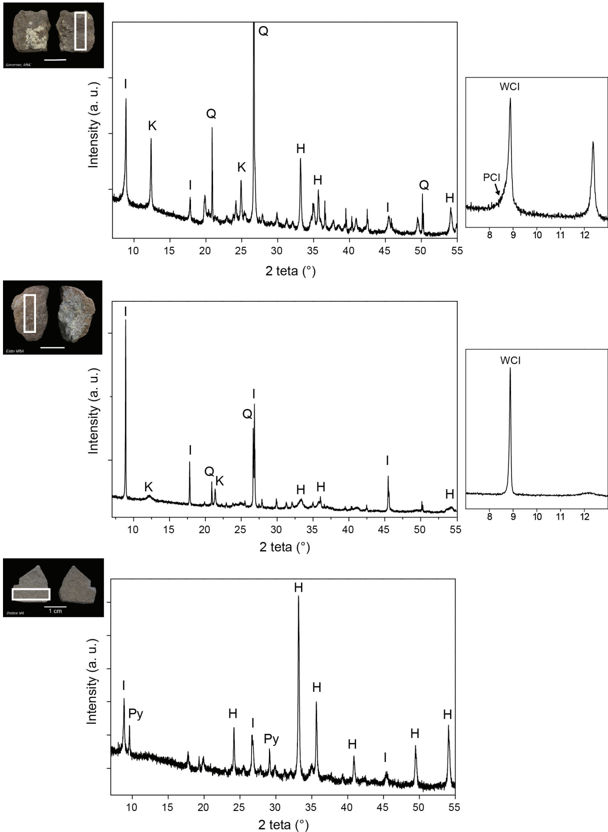
Figure 65 – Résultats de l'analyse par DRX permettant d'identifier les phases minéralogiques pour les shales. Shale sans caractéristiques particulières, illite WCI et illite PCI toutes deux présentes (A). Shale avec uniquement illite PCI (B). Shale avec pyrophyllite (C).
