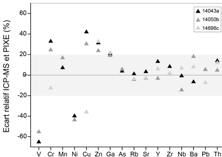
Figure 22 – Diagramme présentant l'écart relatif entre les teneurs PIXE et ICP-MS en fonction des éléments traces, pour 3 échantillons de shale géologiques. Des différences supérieures à 20 % s'observent pour les éléments dont la raie principale est proche de celle du fer, soit avant (V, Cr), soit après (Ni, Cu, Zn, et Ga).
