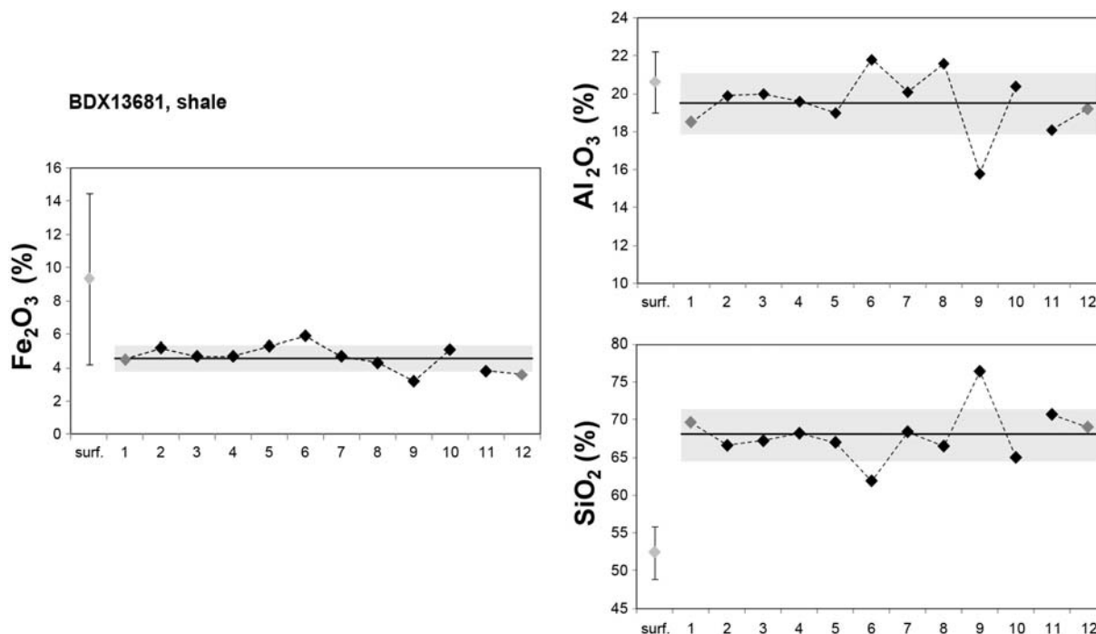
Figure 21 – Profils de composition déterminés par EDXS sur section de un échantillon de shale, comparé à la composition déterminée en surface. Une moyenne et un écart-type (droite et un rectangle gris) ont été calculés sur l'ensemble du profil (12 zones d'analyse). La moyenne et l'écart-type (point gris) ont été calculés à partir de 6 zones d'analyse en surface. Les résultats ont été normalisés à 100 %, en prenant en compte les éléments potentiellement présents dans les dépôts.
