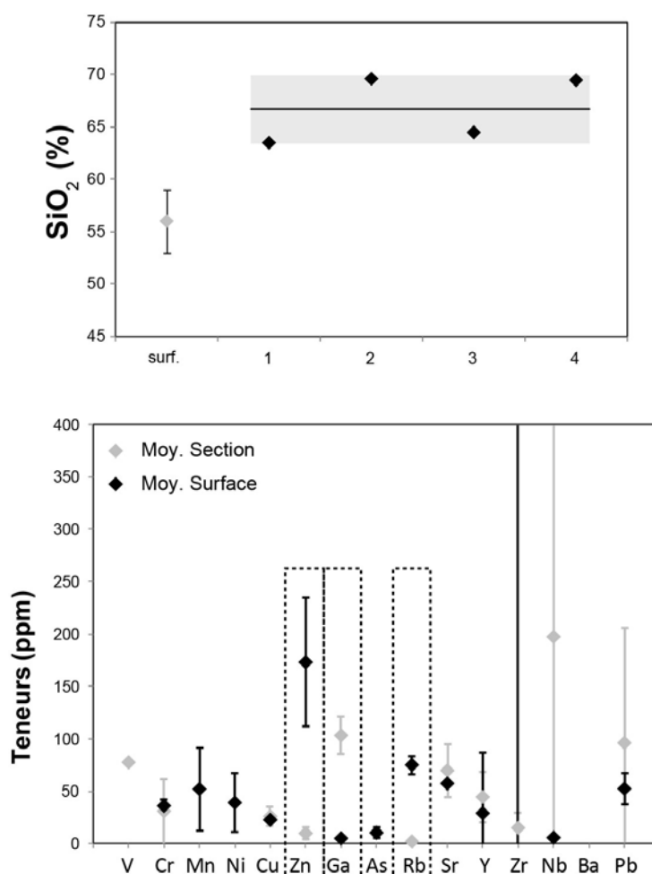
Figure 24 – Comparaison des teneurs en Si, ainsi qu'en éléments traces en surface et section obtenues par PIXE sur un échantillon particulièrement touché par l'altération de surface. Pour le silicium, le point gris correspond à la moyenne en surface, tandis que les points noirs correspondent à l'analyse en section, dont la moyenne et l'écart type sont représentés pour un rectangle gris et une droite.
