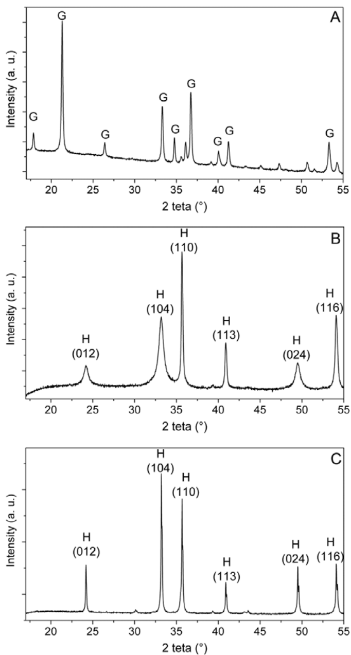
Figure 49 – Diffractogramme d'une goethite synthétique (A) de la même goethite chauffée à 300°C (B) et d'une hématite naturelle bien cristallisée (C) (provenance : île d'Elbe).
