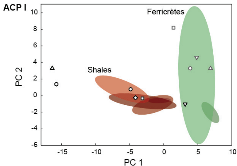
Figure 35 - Attribution de 10 échantillons archéologiques selon l'ACP I réalisées sur l'ensemble des éléments traces. Discrimination selon le type de matière première.
