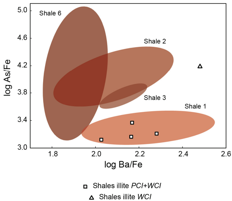
Figure 67 – Attribution de 5 shales archéologiques, avec illite bien cristallisée (WCI), ou illite plus ou moins bien cristallisée (WCI+PCI), selon le diagramme binaire log As/Fe en fonction de log Ba/Fe (ICP-MS).
