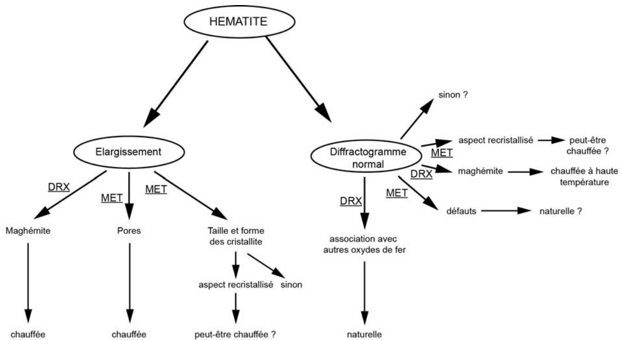
Figure 8 – Schéma illustrant le protocole d'étude du chauffage de la goéthite par DRX et MET (Extrait de Pomies, 1997).
