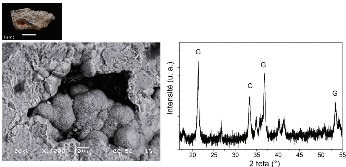
Figure 28 – Suite figure précédente, image MEB et diffractogramme d'un échantillon de ferricrète géologique collecté sur l'une des sources associées aux formations Malmesbury (Ferr 1).
