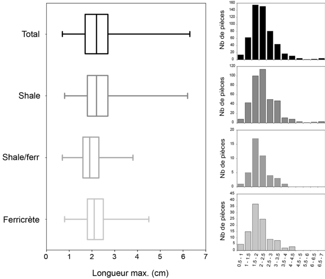
Figure 62 – Distribution de la longueur maximale des pièces en fonction des trois principales catégories de matière première. Les box-plots représentent les quartiles ainsi que les minima et maxima (distribution non normale).
