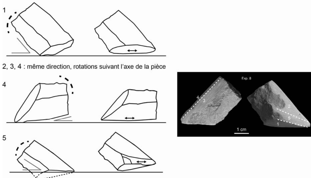
Figure 56 – Reconstitution des différentes étapes de l'abrasion d'un bloc de shale pour la production de poudre (2h de traitement). Les pointillés indiquent la zone tenue par l'expérimentateur, la double flèche la direction des stries et l'angle représente l'angle de dépouille aigu.
