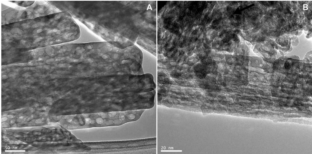
Figure 52 – Images en transmission des cristaux d'hématite obtenue par chauffage de goethite, une goethite synthétique chauffée au maximum à 480°C et une goethite naturelle chauffée selon le même cycle.
