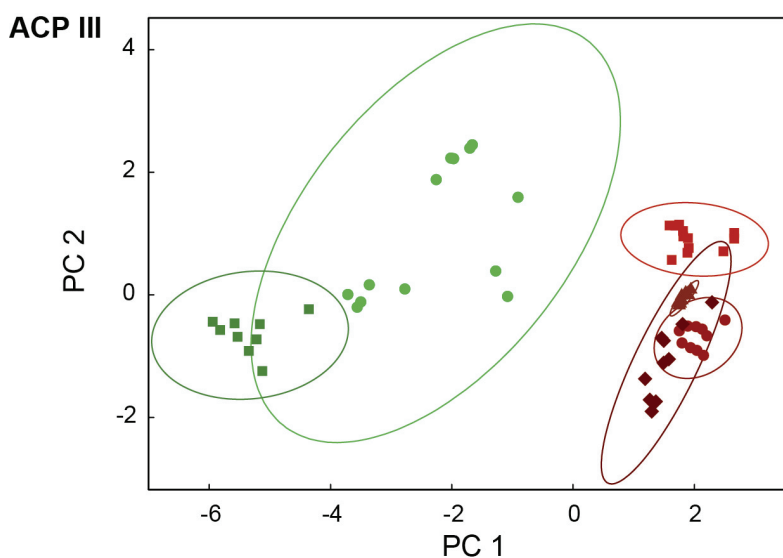
Figure 32 - Composantes 1 et 2 de l'ACP III réalisées sur les logs des rapports au fer de 10 éléments traces, discrimination selon le type de matière première.
