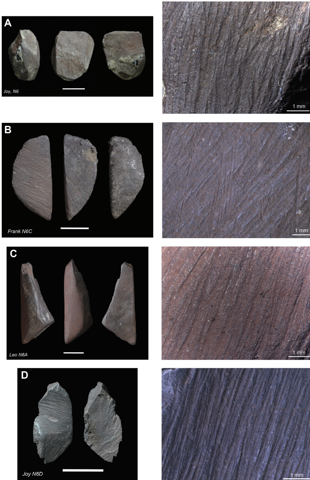
Figure 73 – Pièces facettés et détails des surfaces striées. Shale avec une facette d'abrasion recoupée par plusieurs fractures (A) ; ferricrètes avec facettes d'abrasion (B et C) ; et ferricrètes avec une face concave striée, recoupée par une fracture, soit raclée, soit abrasée sur une surface convexe (D).
