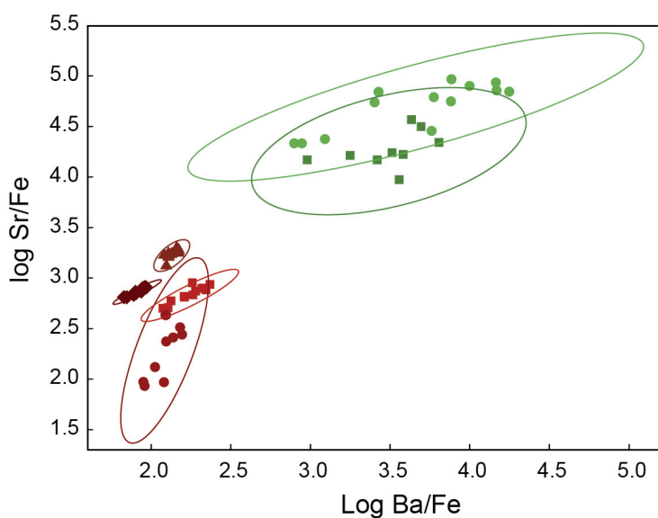
Figure 33 – Diagramme binaire log Sr/Fe et log Ba/Fe, éléments corrélés au fer dans les ferricrètes, discrimination selon le type de matière première. Ellipses de confiance : 95 %.
