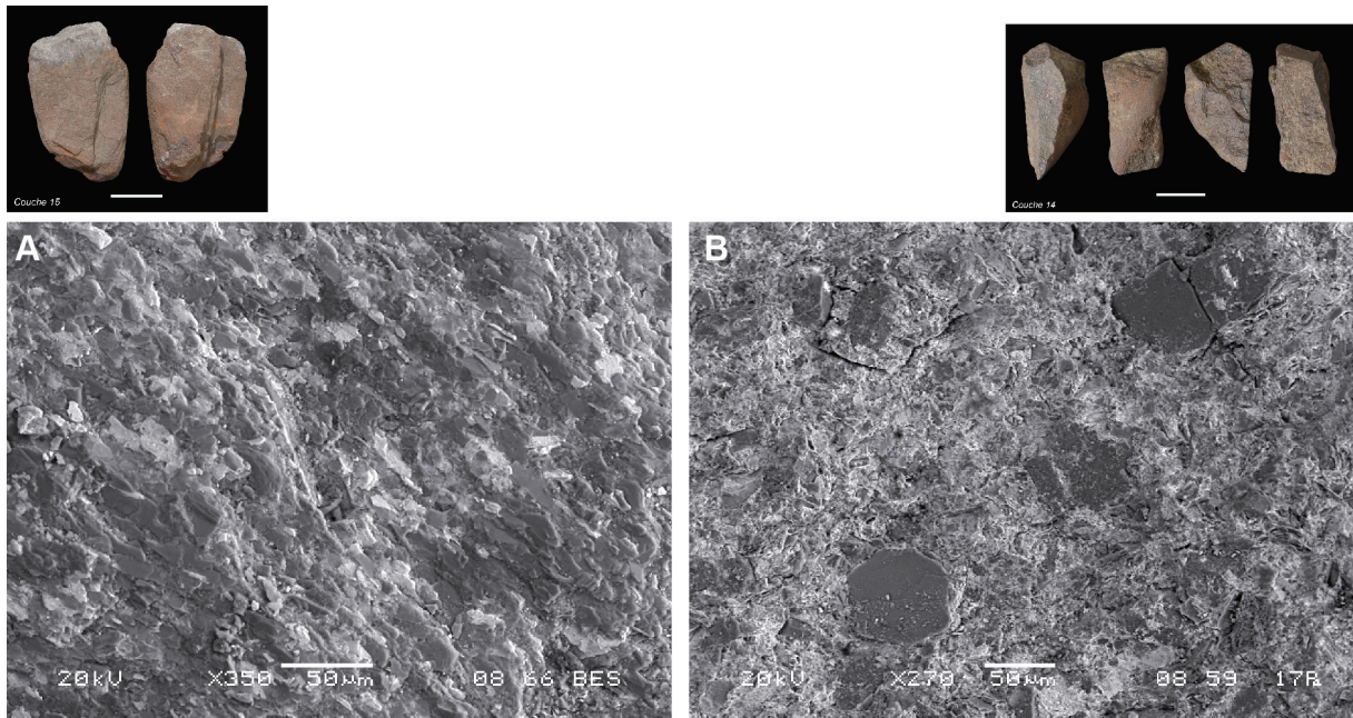
Figure 86 – Microstructures de roches à grains fins observées au MEB-EDXS en électrons rétrodiffusés. Microstructure en feuillet juxtaposée (A), et microstructure avec tablettes silteuses (taille entre 4 et 66μm) dispersées au sein de la fraction fine (B).
