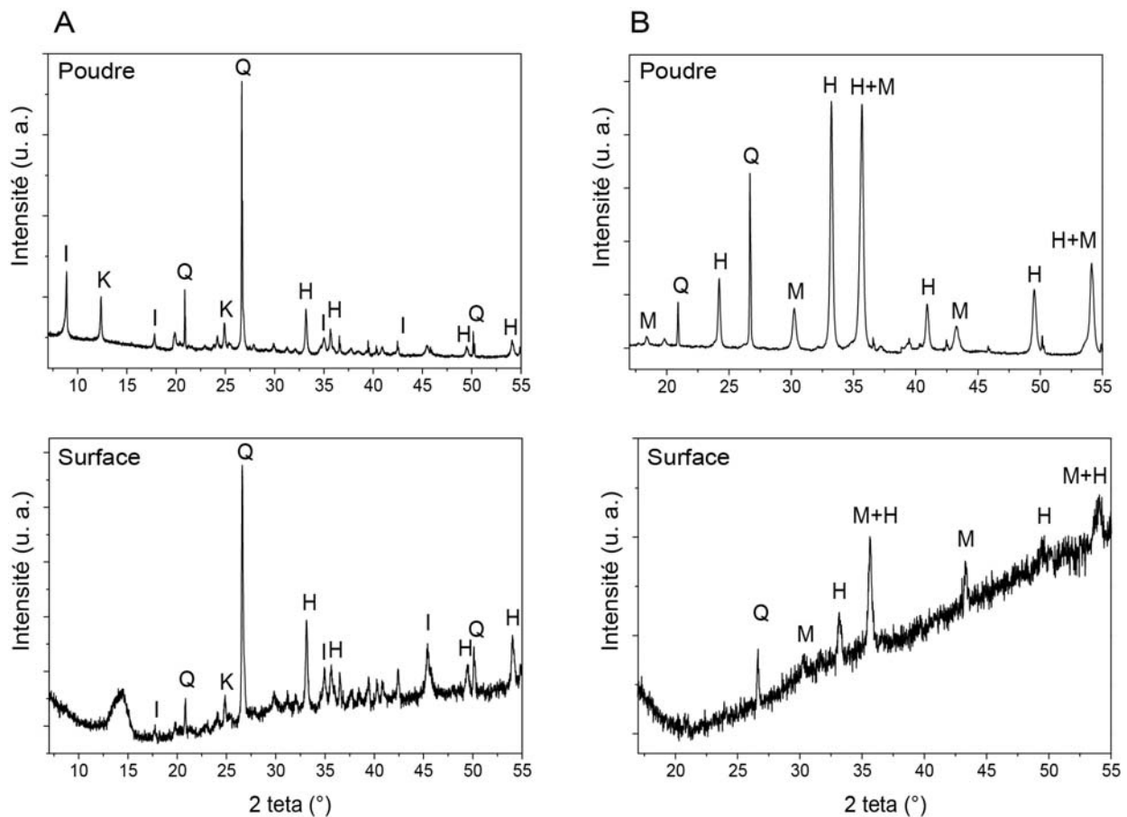
Figure 25 – Comparaison de l'analyse sur poudre (montage Bragg-Brentano) et de l'analyse en surface (montage faisceau parallèle) pour un échantillon de riche en argiles et un riche en oxydes de fer.
