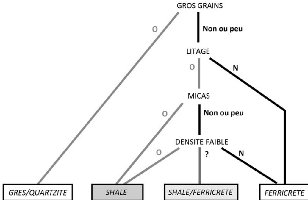
Figure 26 – Arbre de décision établi pour la classification des matières premières par l'observation seule.
