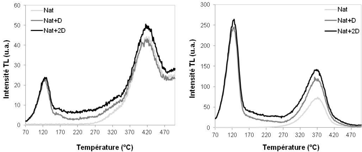
Figure 53 – Courbes de thermoluminescence d'un échantillon géologique (gauche) et d'un échantillon archéologique (droite). Alors qu'aucune croissance en dose n'est observée pour le premier, le signal augmente en fonction de la dose ajoutée pour le second, ce qui est caractéristique d'une chauffe dans le passé.
