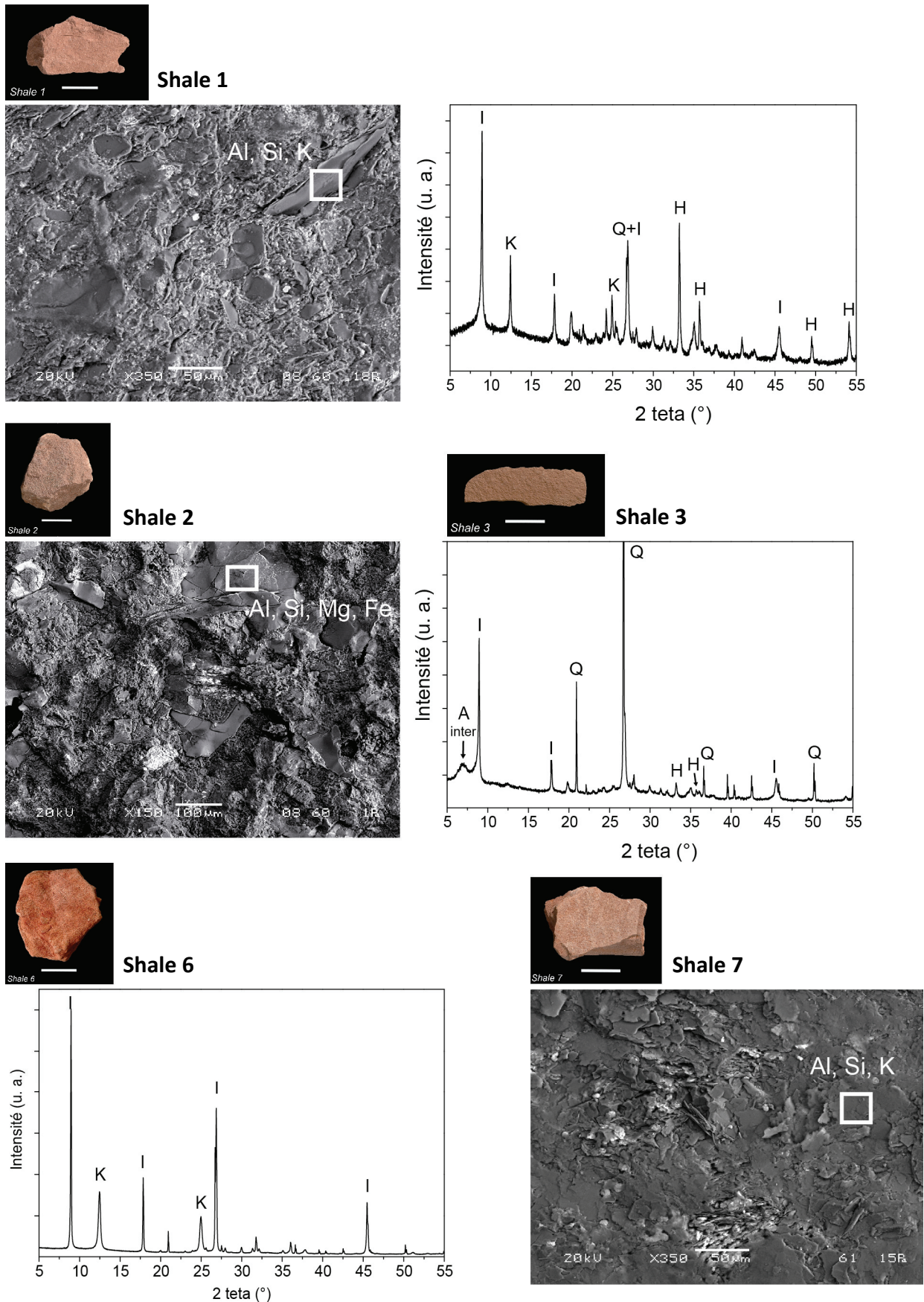
Figure 27 – Images MEB en électrons rétrodiffusés montrant la microstructure des shales selon les sources, et diffractogrammes montrant leur composition minéralogique.
