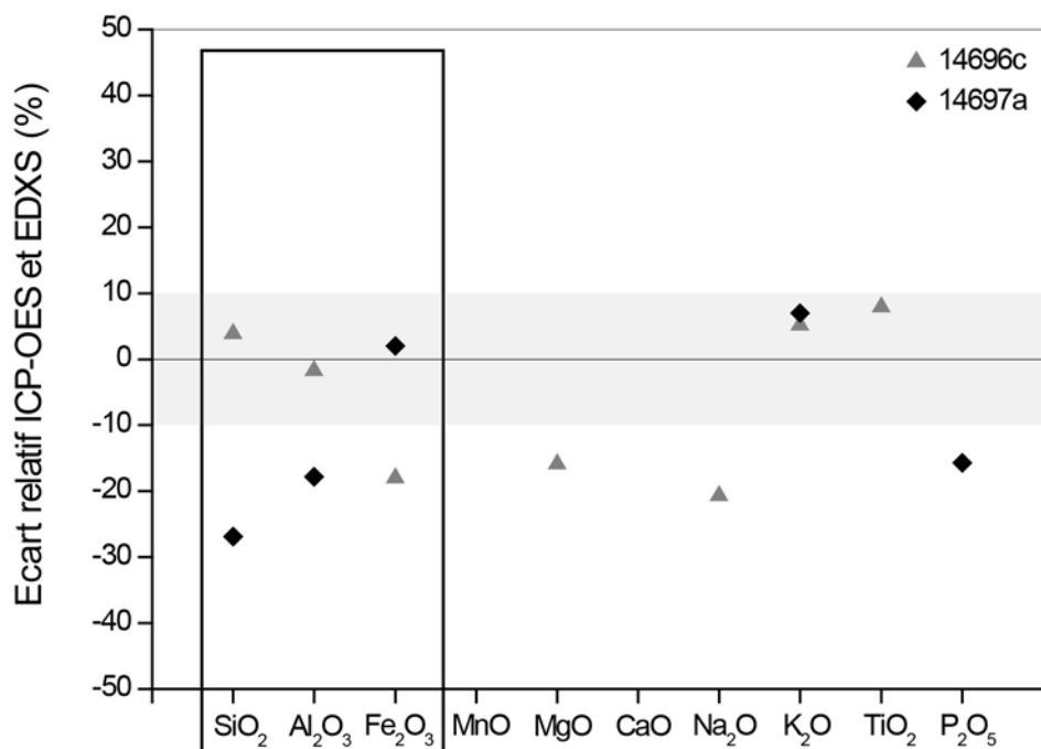
Figure 19 – Diagramme présentant les écarts relatifs entre EDS et ICP pour les éléments majeurs et mineurs (teneurs >1%), pour un échantillon de shale avec Si et Al majeurs (14696ca) et pour un échantillon de ferricrète avec Fe majeur (14697a).
