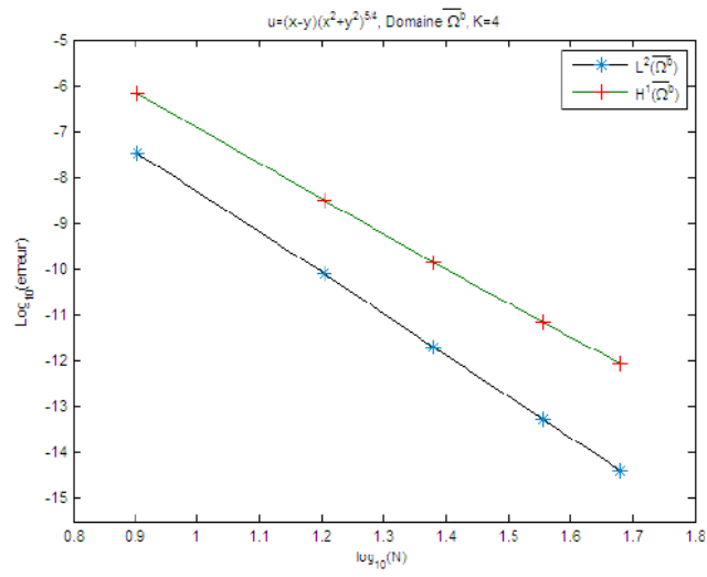
Fig. 2.7.30: Courbe d'erreur
