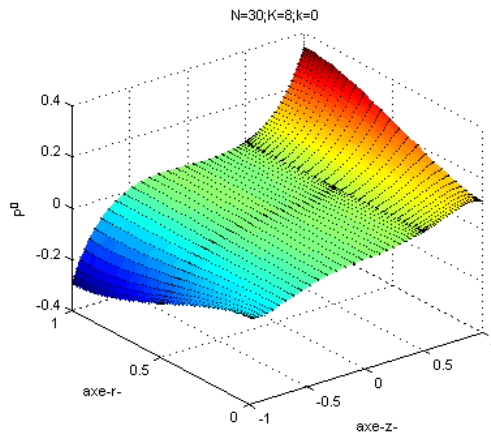
Fig. 3.6.24: Tracé de la fonction p^0
