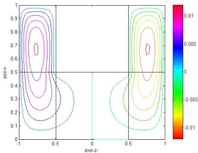
Fig. 2.7.29: Isovaleurs de \text{Re}(u^1)
