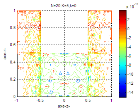
Fig. 3.6.37: Isovaleurs de u_r^0
