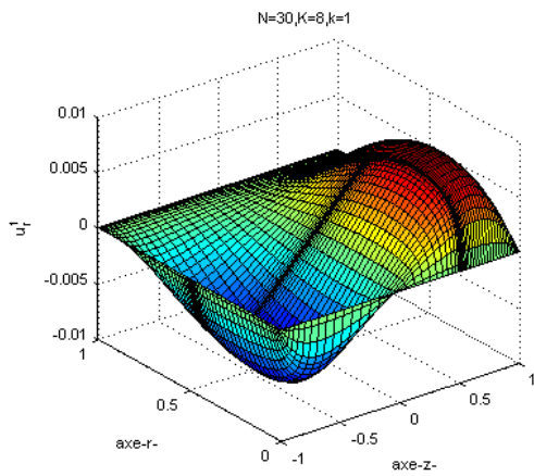
Fig. 3.6.25: Tracé de la fonction u_r^1
