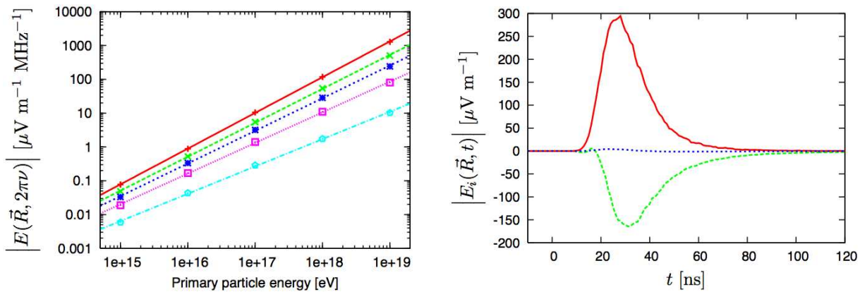
FIGURE 3.2 – Gauche : simulation (REAS1) du champ électrique émis par une gerbe verticale de 10^{17} eV en fonction de l'énergie de la particule primaire, pour différentes distances. De bas en haut : 20 m, 100 m, 180 m, 300 m and 500 m du coeur de la gerbe. Droite : impulsions simulées (REAS1) observées à 200 m au nord d'une gerbe verticale de 10^{17} eV en polarisation est-ouest (en rouge), nord-sud (en vert) et verticale (en bleu). Extraits de [163].
