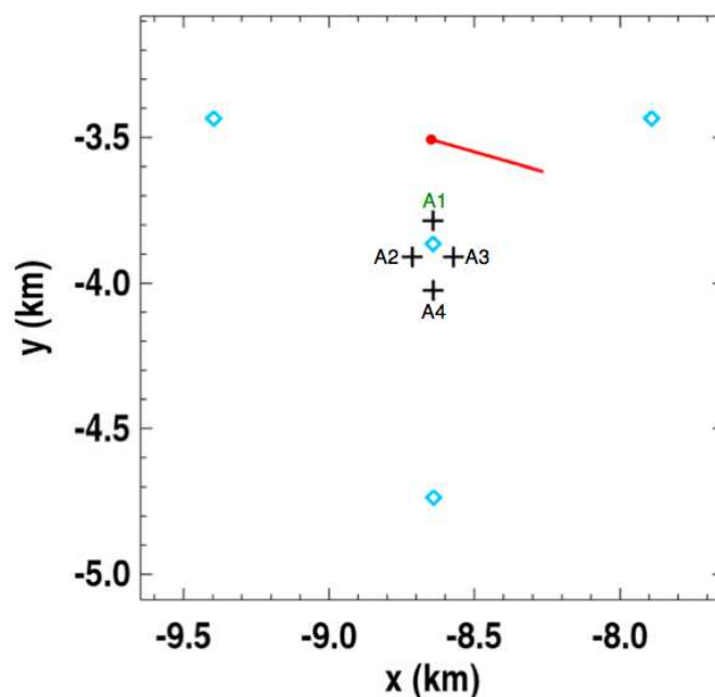
FIGURE A.1 – Géométrie de l'évènement répertorié dans la base de données Auger sous le numéro 1293405794. Voir texte pour le détail.
