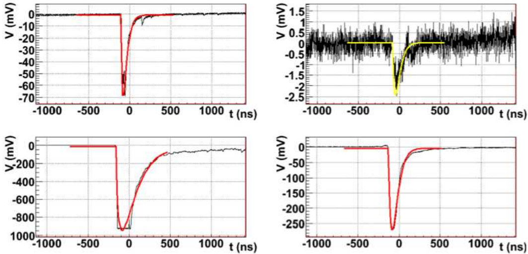
FIGURE 2.17 – Exemple de deux évènements différents (haut et bas) observés par deux couples de photomultiplicateurs (à gauche, haut gain, à droite, bas gain) ainsi que leur ajustement (courbes). En haut, aucun des photomultiplicateurs ne sature, c'est le haut gain qui sera utilisé. En bas, le photomultiplicateur haut gain sature, c'est le bas gain qui sera utilisé.
