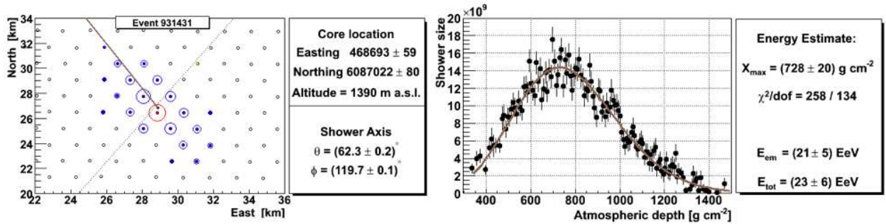
FIGURE 1.38 – Gauche : Empreinte au sol déposée par un évènement hybride de 23 EeV mesurée par le détecteur de surface. Droite : même évènement observé par les détecteurs de fluorescence. Cette figure donne la taille de la gerbe en fonction de la profondeur traversée. Un ajustement de l'évolution du profil permet d'obtenir la grandeur X_{max} où le nombre de particule atteint son maximum.
