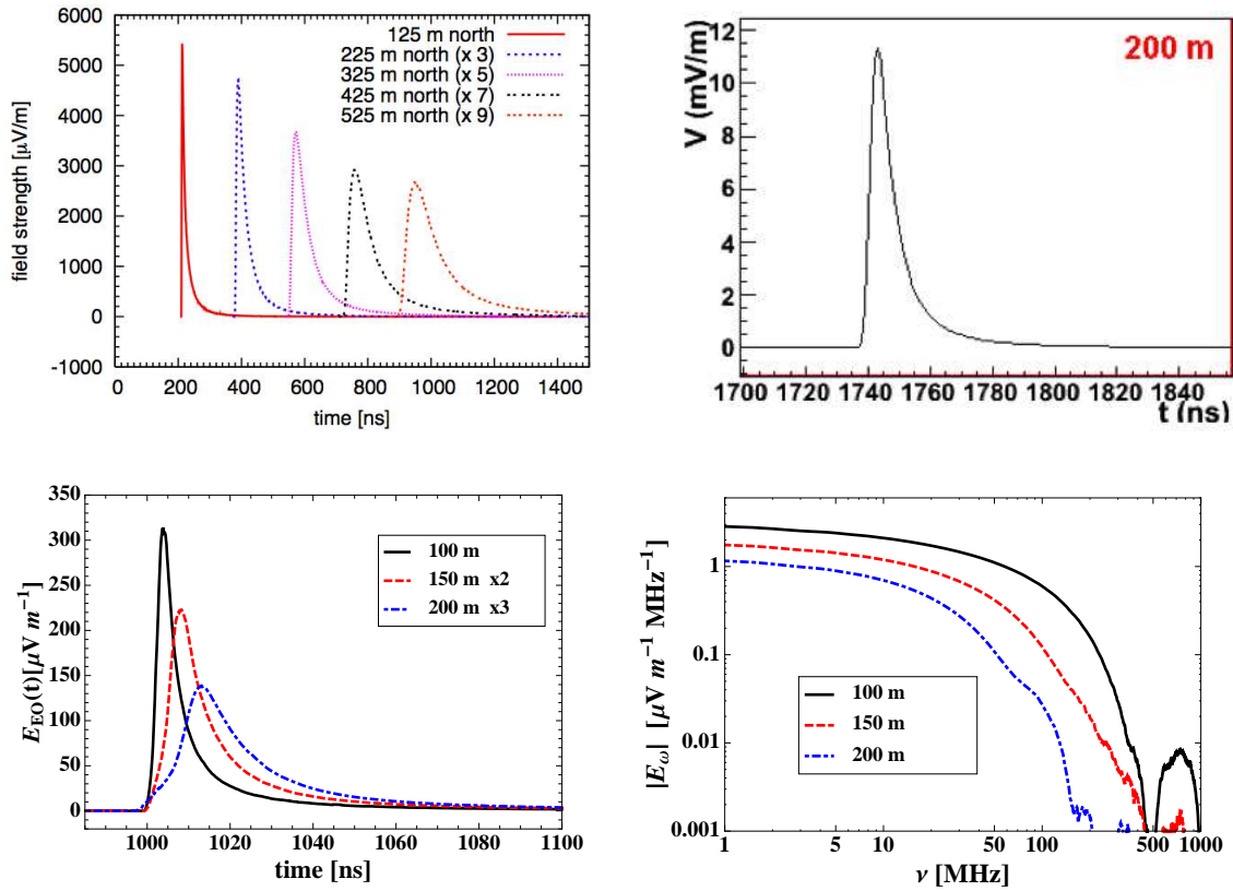
FIGURE 3.8 – Exemple de résultats obtenus avec REAS2 (en haut à gauche) [176] , ReAires (en haut à droite) [138] et SELFAS1 (en bas à gauche) [175]. Les cas de gerbes simulées correspondent toutes à des gerbes initiées par des protons de 10^{17} eV mais ont des directions d’arrivée différentes. L’idée étant de montrer que toutes ces impulsions ont une caractéristique commune : elles sont monopolaires. En bas à droite : spectres correspondant aux impulsions obtenues avec SELFAS1.
