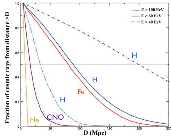
FIGURE 1.23 – Fraction de rayons cosmiques qui survivent en fonction de la distance parcourue, de leur nature et de leur énergie initiale [48].
