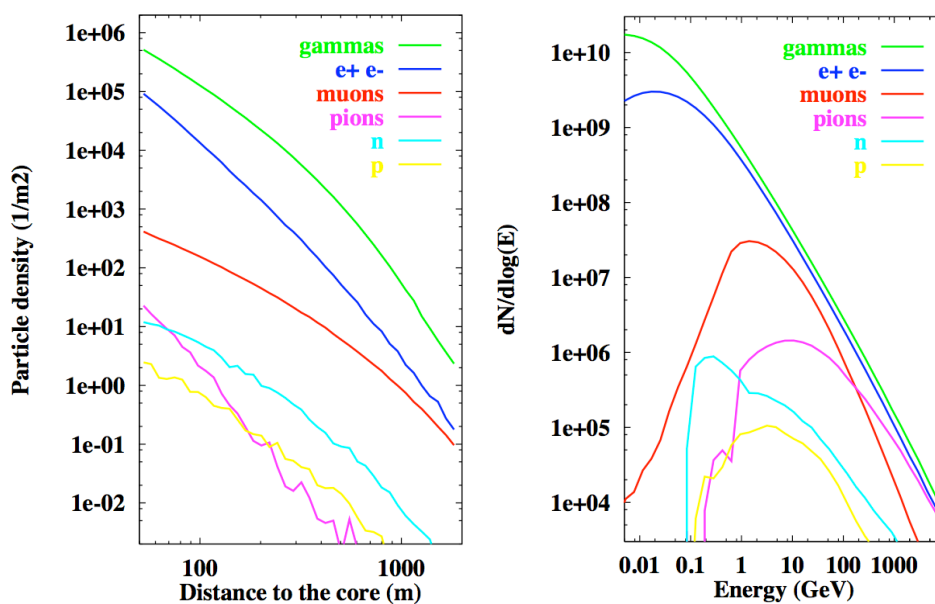
FIGURE 1.28 – Gauche : distribution latérale du nombre de particules en fonction de leur nature. Droite : distribution latérale en énergie des particules en fonction de leur nature. Ces deux figures correspondent au cas d'une gerbe initiée par un proton de 10^{19} eV [66].
