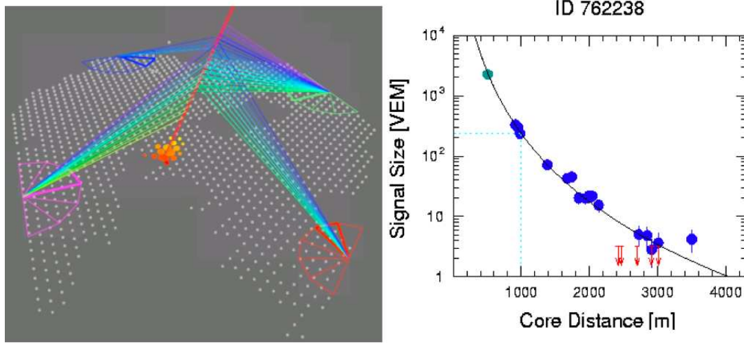
FIGURE 1.36 – Gauche : premier évènement hybride observé par les quatre télescopes de fluorescence ainsi que 15 cuves du réseau de surface le 20 mai 2007. Droite : distribution latérale au sol de l'énergie déposée par cet évènement de 10^{19} eV.
