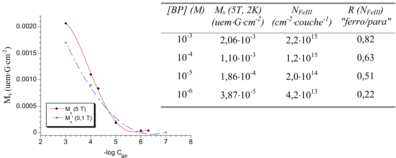
Fig. 3.9. Aimantation à saturation (5 T) obtenue de la courbe d'aimantation en fonction du champ à 2 K et aimantation à 0,1 T des cycles d'hystérésis pour films LB \text{Rub}^{2+}/\text{BP} en fonction de la concentration de BP en sous-phase.
