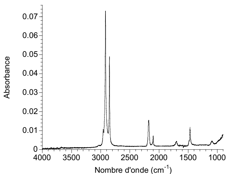
Fig. 4.4. Spectre IR du film LB DODA / \text{FeCNCu} 10^{-4} M (20 couches sur \text{CaF}_2 + \text{AB} ).
