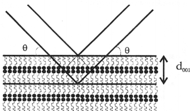
Fig. AIII1. Réflexion de Bragg d'un film LB de type Y.
