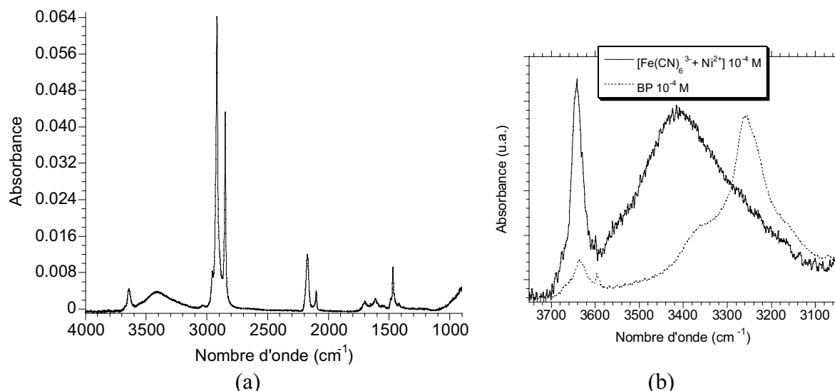
Fig. 4.6. (a) Spectre IR du film LB DODA / \text{FeCNNi} 10^{-4} M (20 couches sur \text{CaF}_2 + \text{AB} ). (b) Comparaison des bandes de vibration O-H avec celles du film LB \text{Ru}^{2+} / BP 10^{-4} M (chapitre 2).
