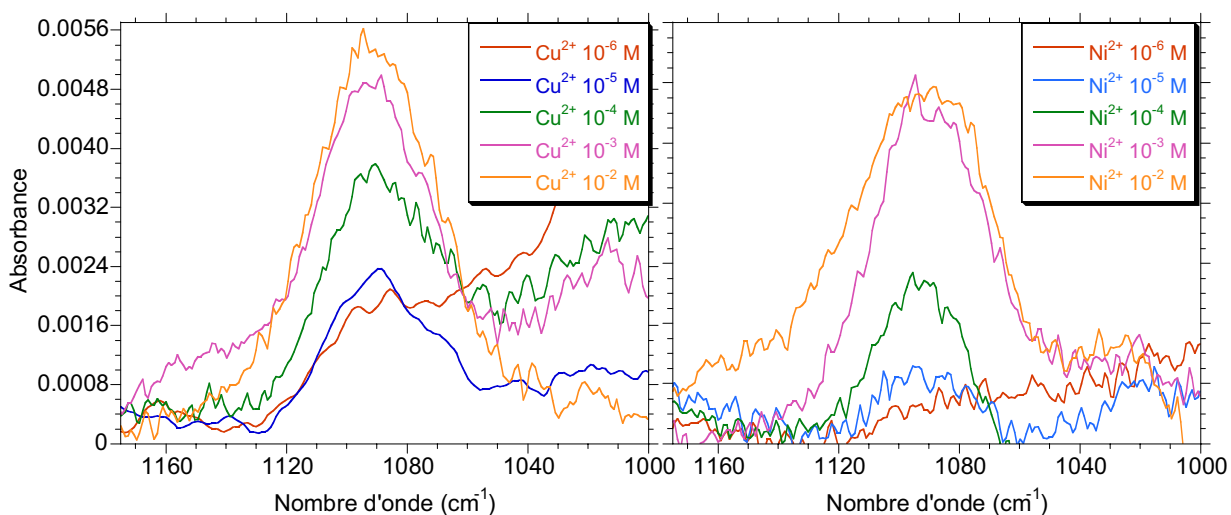
Fig. 5.10. Bandes de vibration Cl-O des spectres IR des films LB RubCN / \text{A}(\text{ClO}_4)_2 (20 couches sur \text{CaF}_2 ).
