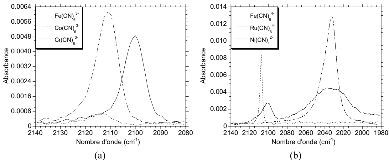
Fig. 1.20. Bandes du spectre IR de la vibration CN du film LB (a) DODA / M(\text{CN})_6^{3-} \cdot 5 \cdot 10^{-6} M et (b) DODA / M(\text{CN})_6^{4-} et DODA / \text{Ni}(\text{CN})_4^{2-} \cdot 5 \cdot 10^{-6} M (20 monocouches sur \text{CaF}_2 + \text{AB} ).
