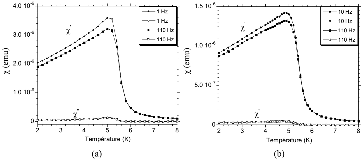
Fig. 3.8. Dépendance de la température des susceptibilités magnétiques AC à différentes fréquences pour les films LB (a) \text{RuB}^{2+} / BP et (b) DODA / BP 10^{-6} M (100 couches).
