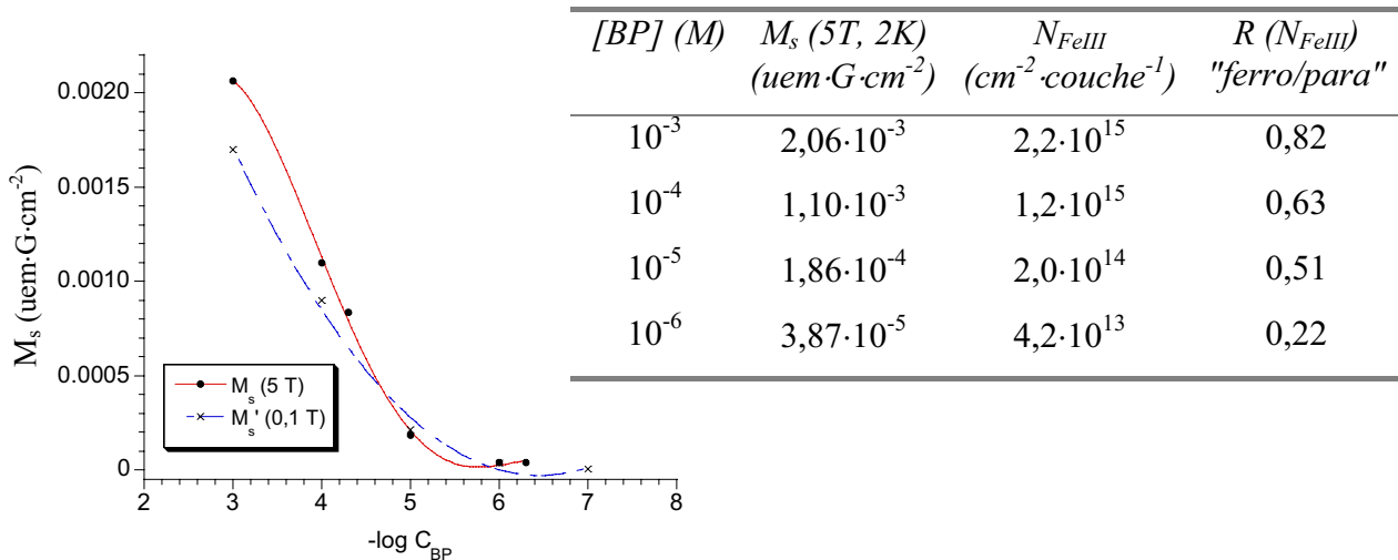
Fig. 3.9. Aimantation à saturation (5 T) obtenue de la courbe d'aimantation en fonction du champ à 2 K et aimantation à 0,1 T des cycles d'hystérésis pour films LB \text{RuB}^{2+} / BP en fonction de la concentration de BP en sous-phase.
