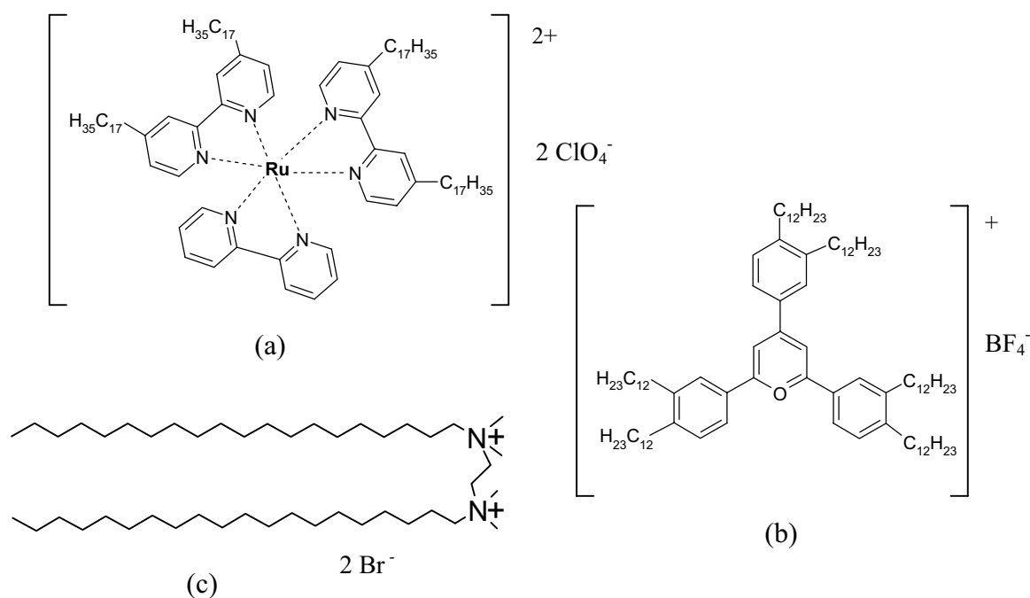
Fig. 2.4. Structures moléculaires des amphiphiles (a) \text{Rub}^{2+} (b) \text{Ar}_3 et (c) \text{Gem} .
