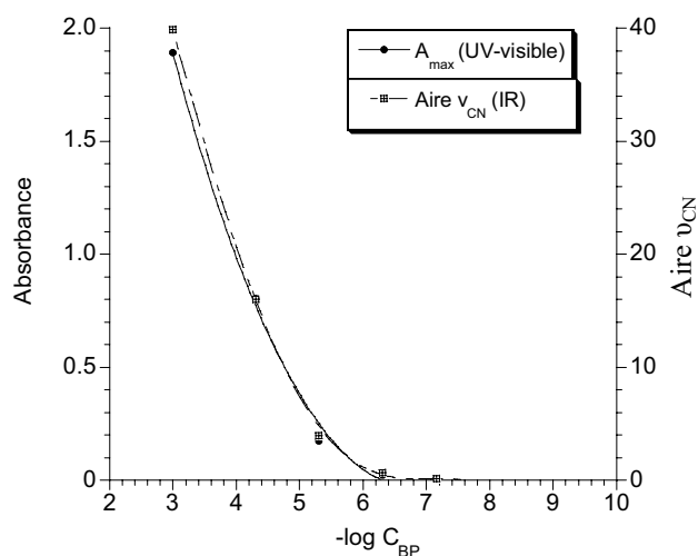
Fig. 3.13. Comparaison des résultats obtenus en UV-visible et IR pour les signaux correspondants de la vibration cyanure.
