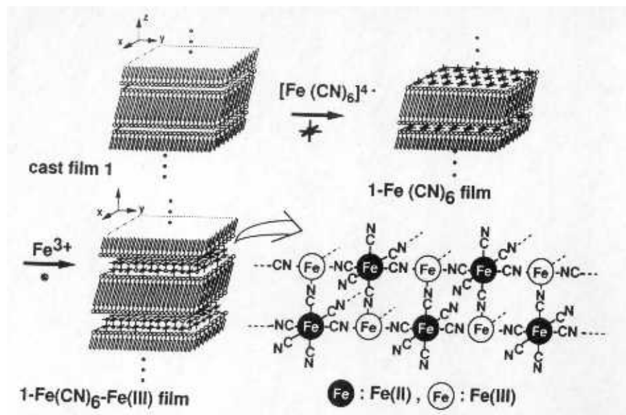
Fig. 2.2. Illustration schématique de la synthèse du complexe bimétallique à valence mixte par l'utilisation du film multicouche [19] .
