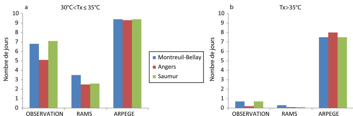
Figure XI.7. Nombre de jours moyen avec températures observées et simulées par ARPEGE-Climat et RAMS à 2 mètres du sol, comprises entre 30 et 35°C (a) et avec températures supérieures au seuil de 35°C (b) pour le mois d'août sur la période 1991-2000.
