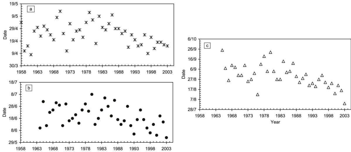
Figure II.20. Evolution des dates des stades de débournement (a), floraison (b) et véraison (c) du cépage Riesling à Bergheim (Alsace)
