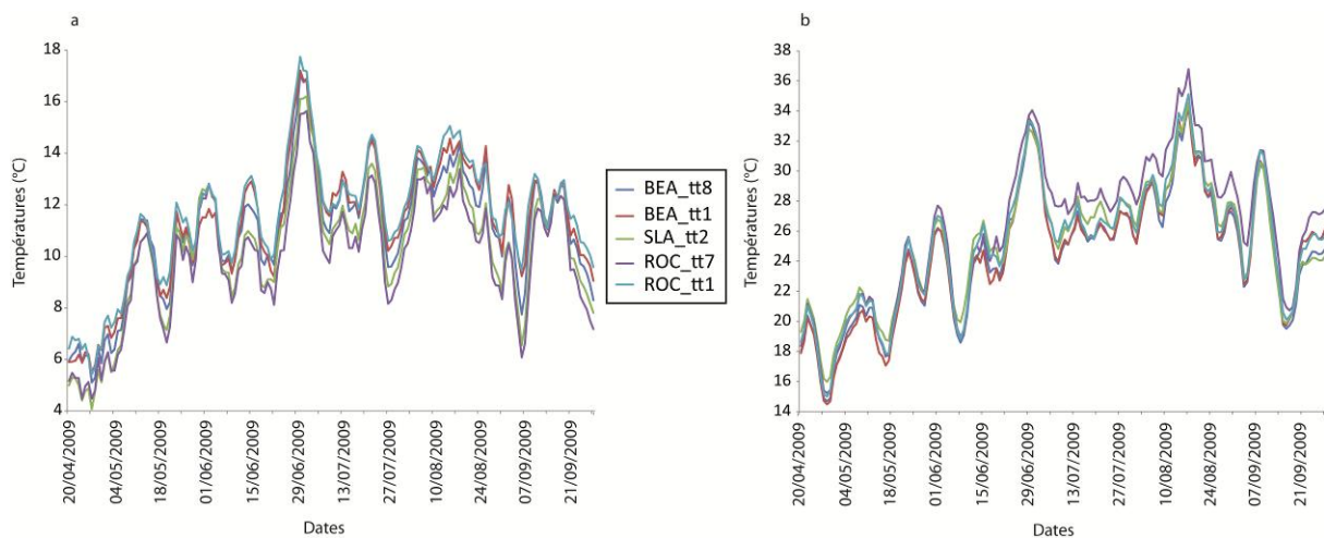
Figure IX.6. Evolution des températures minimales (a) et maximales (b) pour 5 capteurs représentatifs dans les vignobles des Coteaux du Layon durant la saison végétative de 2009. Données : [TERVICLIM/INRA]
