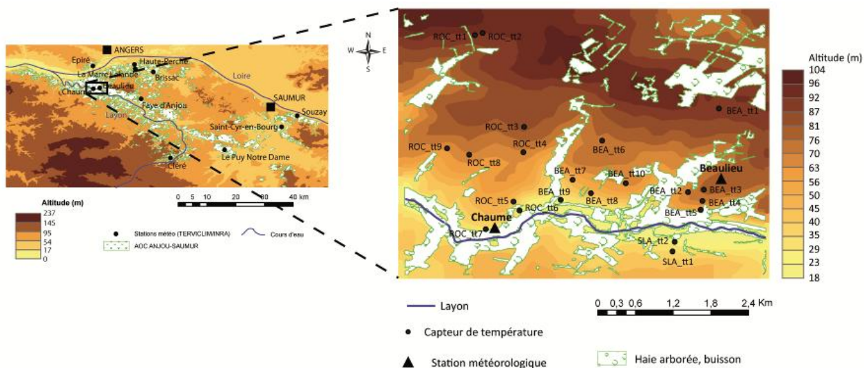
Figure V.9. Zoom sur le réseau de capteurs de température installé dans les Coteaux du Layon. Données : [TERVICLIM/INRA-CTV et BD TOPO-49]
