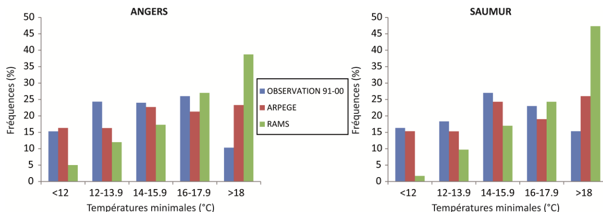
Figure XIII.2. Fréquences des températures minimales journalières, du mois d'août observées et simulées par ARPEGE-Climat et RAMS, selon les classes de l'indice de fraîcheur des nuits, sur la période 2041-2050, d'après le scénario A2 du GIEC, et comparaison avec les données d'observations de la période 1991-2000.
