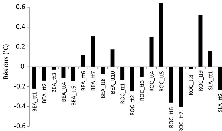
Figure X.7. Résidus moyens (observé-simulé), issus de la modélisation multicritères des moyennes des températures minimales journalières, pour chaque capteur dans le site des Coteaux du Layon. Données : [TERVICLIM]
