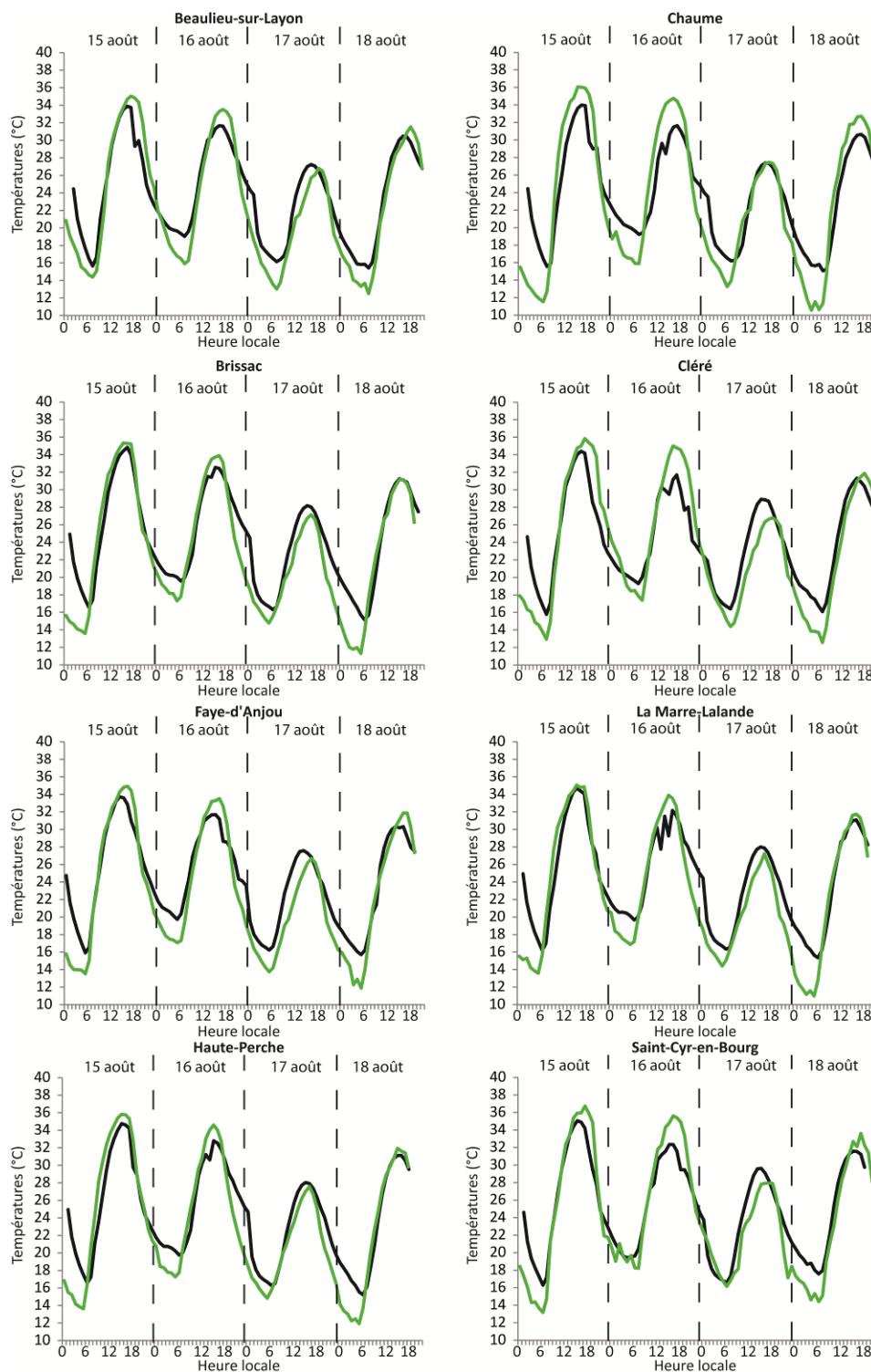
Figure XII.8. Températures horaires observées (en vert) par les différentes stations du réseau TERVICLIM/INRA et simulées par RAMS (en noir) pour la période de fortes chaleurs du 15 au 18 août 2009. Données : [TERVICLIM/INRA et RAMS]
