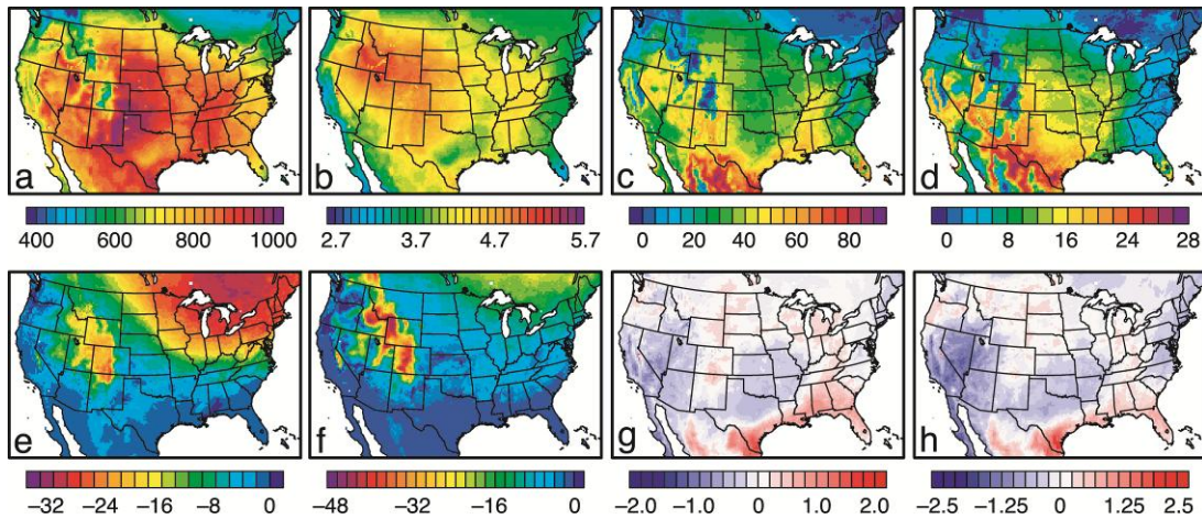
Figure II.10. Changements entre les périodes d'intégration (1961-1989) et future (2071-2099 ; scénario A2) simulés par le modèle RegCM3 du SRES. (a) Degrés-jours ; (b) Température moyenne saisonnière ; (c) Journée chaudes ( T_x > 35^\circ\text{C} ) durant la saison végétative ; (d) Jours chauds ( T_x > 35^\circ\text{C} ) durant la période de maturation ; (e) Jours froids hivernaux ( T_n < -12,2^\circ\text{C} ) ; (f) Jours froids en automne et au printemps ( T_n < -6,7^\circ\text{C} ) ; (g) amplitude thermique diurne moyenne sur la saison végétative ; (h) amplitude thermique diurne moyenne sur la période de maturation.
