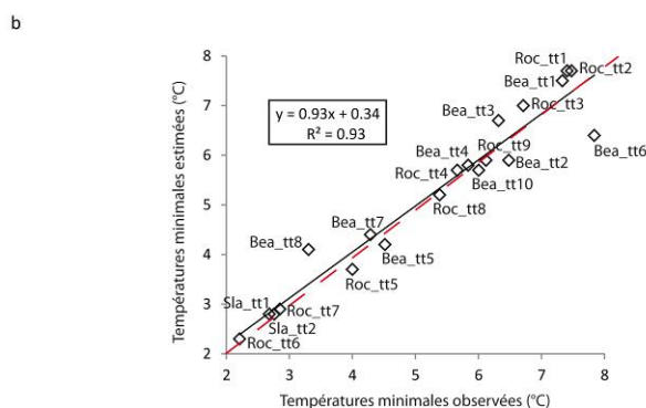
Figure X.8. Spatialisation de la température minimale pour la journée du 29 octobre 2009 (a) et graphique cartésien des températures minimales enregistrées par les capteurs et des températures minimales estimées par le modèle multicritères (b).
