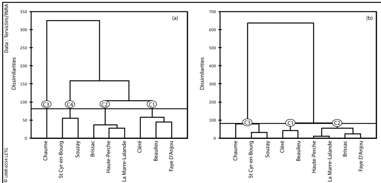
Figure IX.1. Dendrogramme de la classification ascendante hiérarchique appliquée sur les séries de données de températures de la saison végétative 2010 (a : températures minimales, b : températures maximales) du réseau TERVICLIM/INRA en Anjou et Saumurois.
