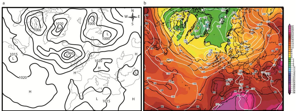
Figure IX.10. Analyses des champs de pression en surface à 12h TU (a) et des températures à 850 hp à 0h TU (b) sur l'Europe durant un épisode caniculaire (15 Août 2009)
