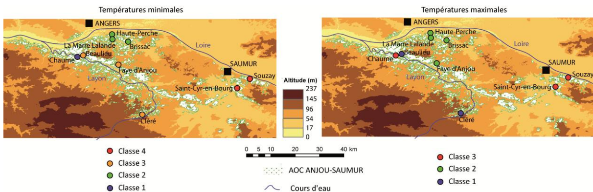
Figure IX.2. Localisation des stations météorologiques utilisées pour la classification ascendante hiérarchique et indication de leur appartenance aux différentes classes.
