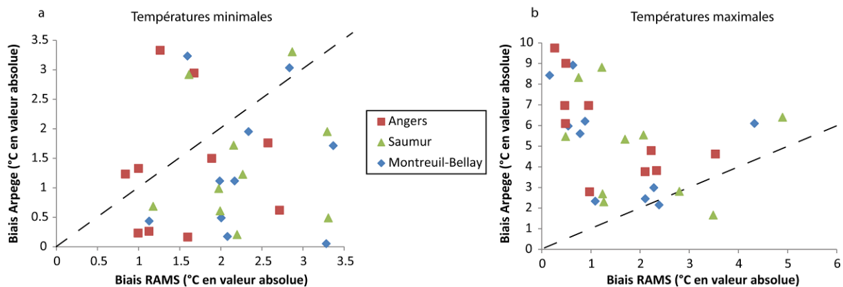
Figure XI.6. Graphique cartésien des biais (en valeur absolue) de ARPEGE-Climat et RAMS pour les températures minimales (a) et maximales (b) moyennes du mois d'août issues de la modélisation de la période de contrôle 1991-2000 (la droite en pointillé représente la 1 ère bissectrice).
