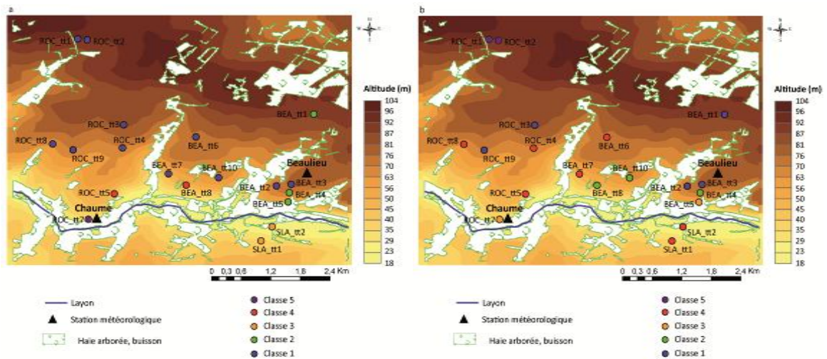
Figure IX.5. Localisation des capteurs de températures utilisés pour les classifications ascendantes hiérarchiques et indication de leur appartenance aux différentes classes.
