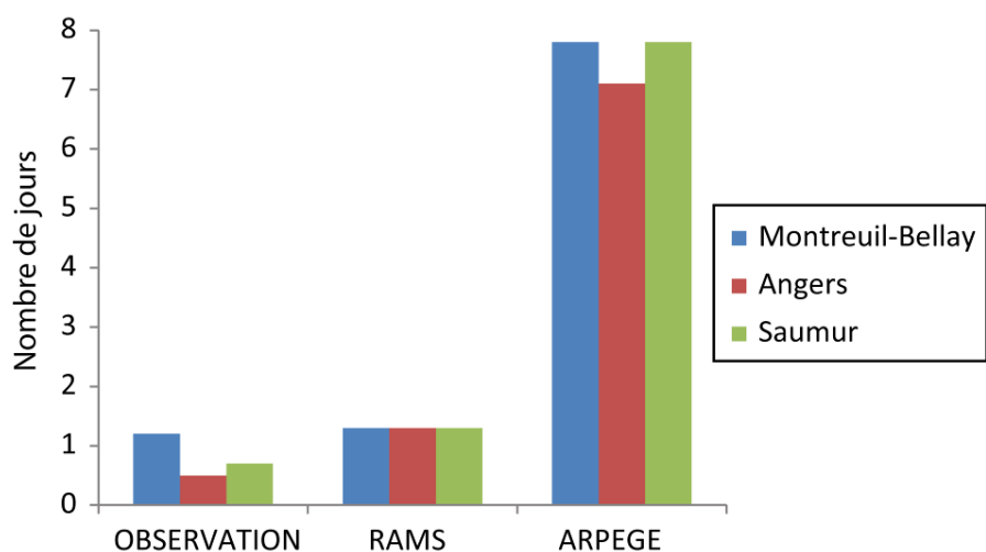
Figure XI.2. Nombre de jours moyen d'occurrence du gel ( T_n < 0^\circ\text{C} ) observé et simulé par RAMS et ARPEGE-Climat à 2 m du sol.
