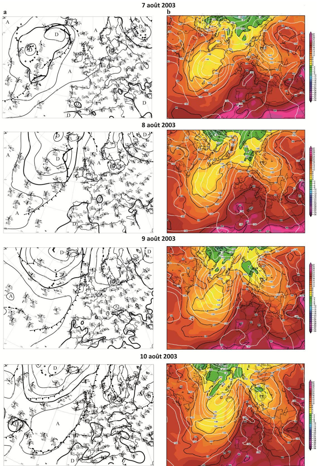
Figure XII.5. Analyses des champs de pression en surface à 12 h TU (a) et des températures à 850 hp à 0h TU (b) sur l'Europe durant l'épisode caniculaire du 7 au 10 août 2003.
