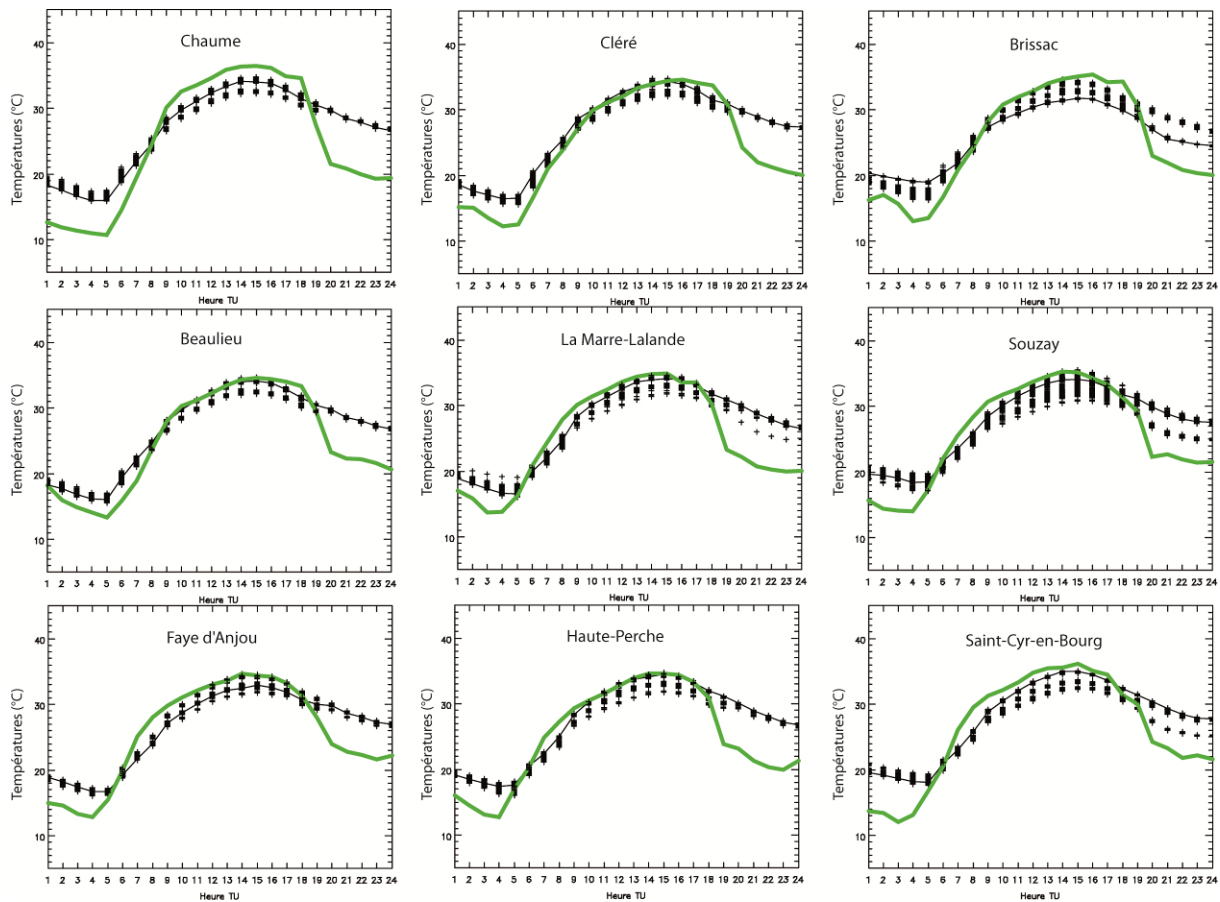
Figure XII.13. Températures horaires observées (en vert) par les différentes stations du réseau TERVICLIM/INRA et simulées par RAMS (en noir) pour le 8 juillet 2010. Les barres de part et d'autre de la courbe noire représentent la variabilité spatiale de la température dans un rayon de 1,5 km autour de la maille correspondant à la station.
