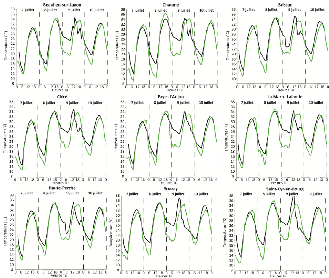
Figure XII.11. Températures horaires observées (en vert) par les différentes stations du réseau TERVICLIM/INRA et simulées par RAMS (en noir) pour la période de fortes chaleurs du 7 au 10 juillet 2010. Données : [TERVICLIM/INRA et RAMS]
